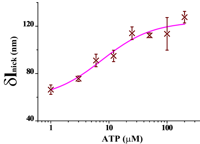
FIG. 4.16 – Translocation de l'ADN en fonction de la concentration d'ATP. Sur cette courbe sont représentées les valeurs moyennes de la taille de la boucle transportée par ISWI ( \langle \delta l_{nick} \rangle ) sur l'ADN nické. Les données ont été ajustées par une cinétique de type Michaelis-Menten ( \delta l_{nick} = l_{sansATP} + \frac{\delta l_{max}[ATP]}{K_M + [ATP]} ), avec un \delta l_{max} \approx 65.5 \pm 7.1 nm, un K_M de 7.6 \pm 3.3 \mu M, et l_{sansATP} ajusté à 58.6 \pm 7.6 nm.
