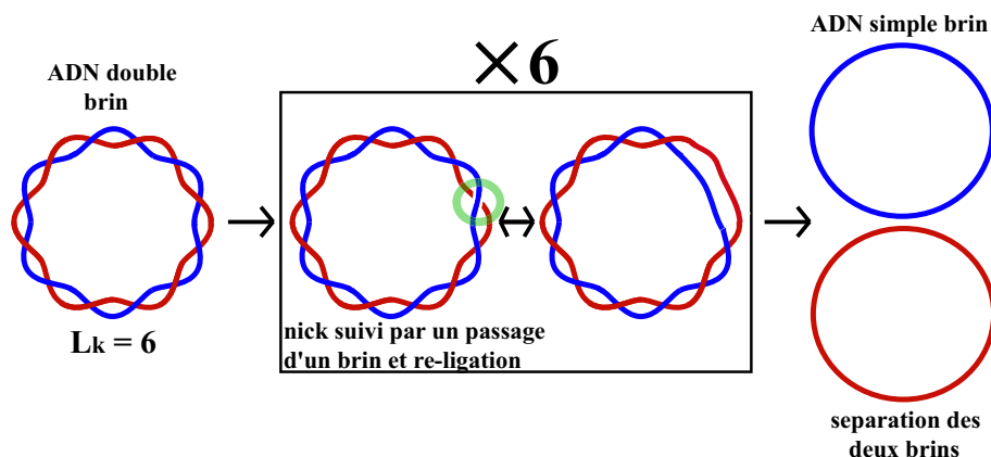
FIG. 4.1 – Schéma montrant une molécule d'ADN circulaire ayant un indice d'enlacement L_{k_0} égal à 6. Une valeur de L_{k_0} = 6 signifie que la molécule d'ADN a 6 tours hélice double brin ou 6 croisements hélice. Si on veut séparer les deux brins de cette molécule d'ADN, on doit effectuer 6 fois une cassure d'un des deux brins de la molécule, forcer ensuite le passage de l'autre brin d'ADN par la cassure et liguer enfin le brin cassé.
