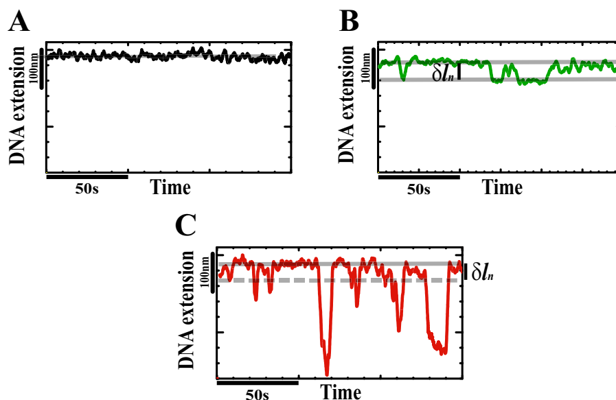
FIG. 4.15 – Translocation de l'ADN par ISWI, en présence d'ATP à F=0.4 pN. Extension de la molécule d'ADN en temps réel sans protéine A), avec ISWI sans ATP B), et avec 200 \mu\text{M} ATP C).
