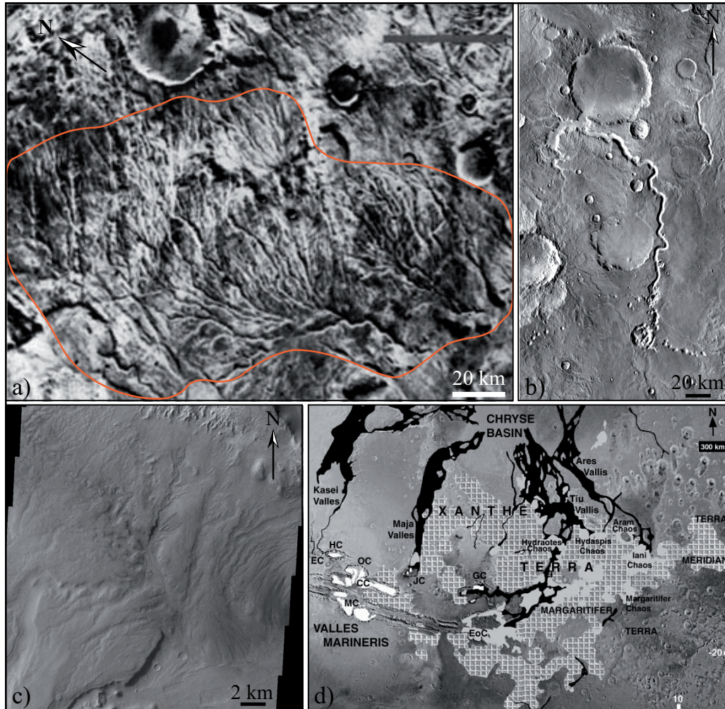
FIGURE 1.11. Extrait d'images représentant les différents réseaux fluviatiles de Mars selon l'époque de formation. a) Extrait d'une image Viking (063A08) représentant Warrego Vallis ( 43^{\circ}\text{S} , 267^{\circ}\text{E} ). Le trait orange souligne la limite possible du bassin-versant de ce système et montre que celui-ci est un réseau mature (d'après Craddock et Howard (2002)). Ce bassin s'est formé durant la période du Noachien. b) Extrait d'une mosaïque THEMIS IR de jour (*-30_150) qui montre un chenal typique de la période Noachien - Hespérien, plus profond, plus large et présentant moins de méandres que ceux formés durant le Noachien ( 4^{\circ}\text{S} , 111^{\circ}\text{E} ). c) Extrait d'une image THEMIS visible (V03249001) montrant un réseau mature formé durant l'Hespérien supérieur (d'après Mangold et al. (2004), 10^{\circ}\text{S} , 77.5^{\circ}\text{E} ). d) Carte représentant la localisation des grands chenaux de débâcle dans la région de Chryse Planitia. Légende d'après Chapman et al. (2003) EC, Echus Chasma; HC, Hebes Chasma; OC, Ophir Chasma; CC, Candor Chasma; MC, Melas Chasma; JC, Juventae Chasma; GC, Ganges Chasma; and EoC, Eos Chasma. Les chenaux de débâcle sont en noirs.
