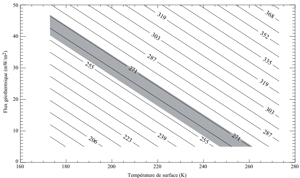
FIGURE 5.15. Graphique de la température moyenne pour une couche de 5000 m recouverte d'une couche de basalte de 1 km d'épaisseur, en fonction de la température de surface et du flux géothermique. La zone grisée représente la zone possible de convection à partir de 258 K jusqu'à 273 K.
