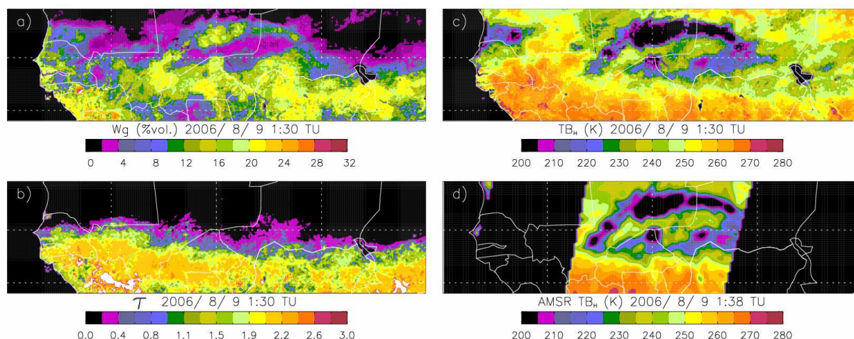
Fig. 4.11: Cartographie de l'humidité du sol (a) obtenue avec le modèle API et les pluies satellite (EPSAT-SG) pour la journée du 9 août 2006 après assimilation. Le modèle C-MEB permet de simuler les températures de brillance micro-onde (H-pol) associées (c). Les observations micro-ondes AMSR-E de la même échéance (9 août 2006, 1:38) sont présentés en (d).
