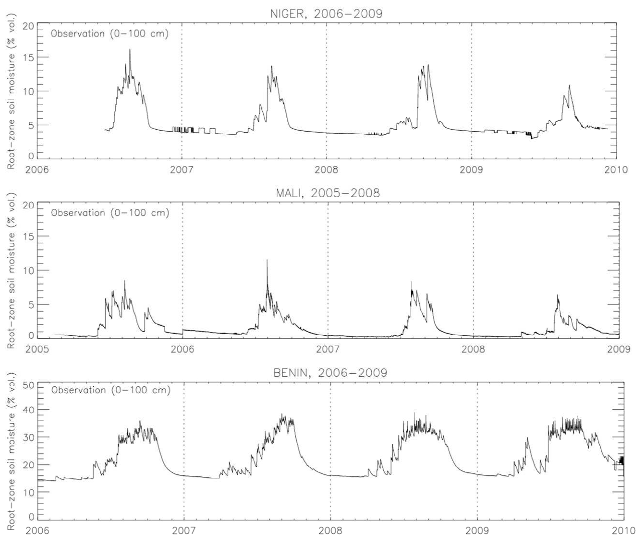
Fig.2.7: Evolution temporelle de l'humidité du sol dans le premier mètre de sol mesurée sur les trois sites au Mali, Niger et Bénin
