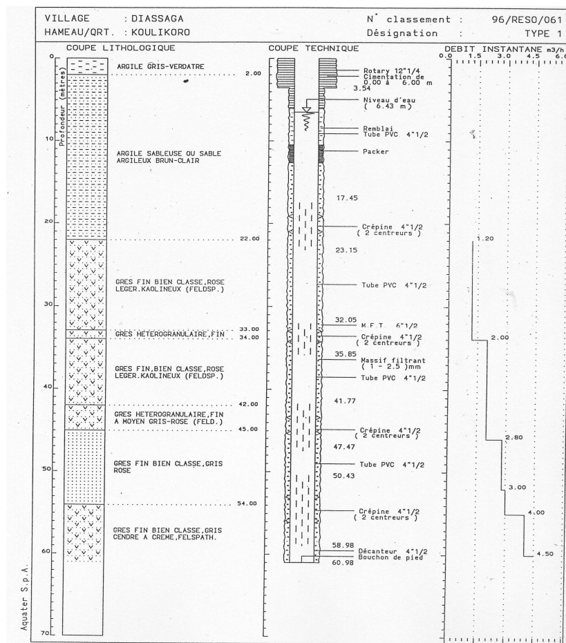
Figure 47: Type d'équipement de forages admettant des mélanges d'eau.
