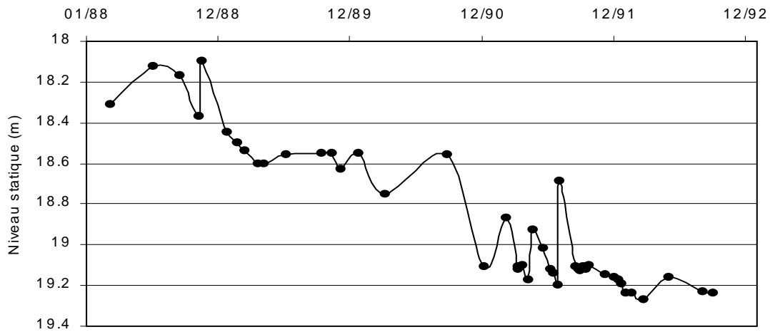
Fluctuations du piézomètre Dédougou-1
