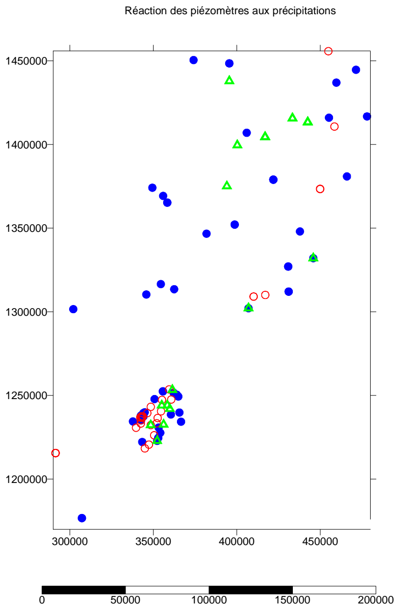
Figure 18 : carte de réactions piézométriques (en cercle plein bleu : réaction positive, en cercle creux rouge : réaction négative, en triangle vert : réaction douteuse)
