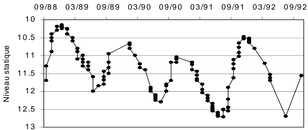
Piézométrie de Banfora 2
