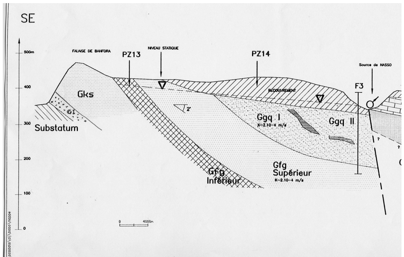
Figure 15-b : Coupe géologique synthétique de la région de Bobo-Dioulasso (extrait de SOGREAH, 1994)
