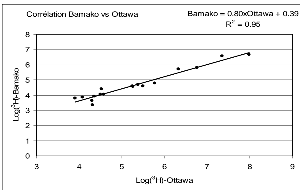
Figure 36: Corrélation entre Bamako et Ottawa en tritium
