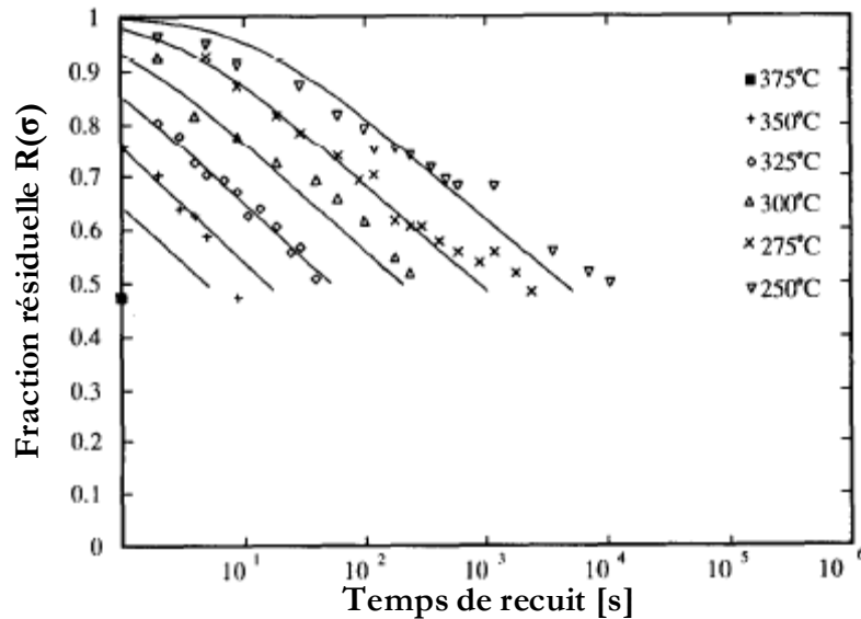
Figure II-17 : Evolution de la fraction résiduelle R(\sigma) au cours d'un recuit pour différentes températures (AA 1050 déformé à froid \epsilon=3 ). Les lignes correspondent à la modélisation. [Furu et al. 1995]
