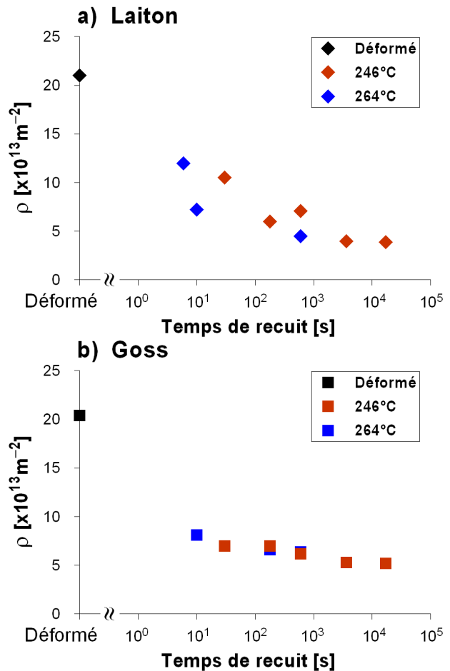
Figure V-14 : Evolution de la densité de dislocations au cours de recuits à 246°C et 264°C pour les monocristaux Laiton (a) et Goss (b) déformés ( \epsilon = 2,3 ).
