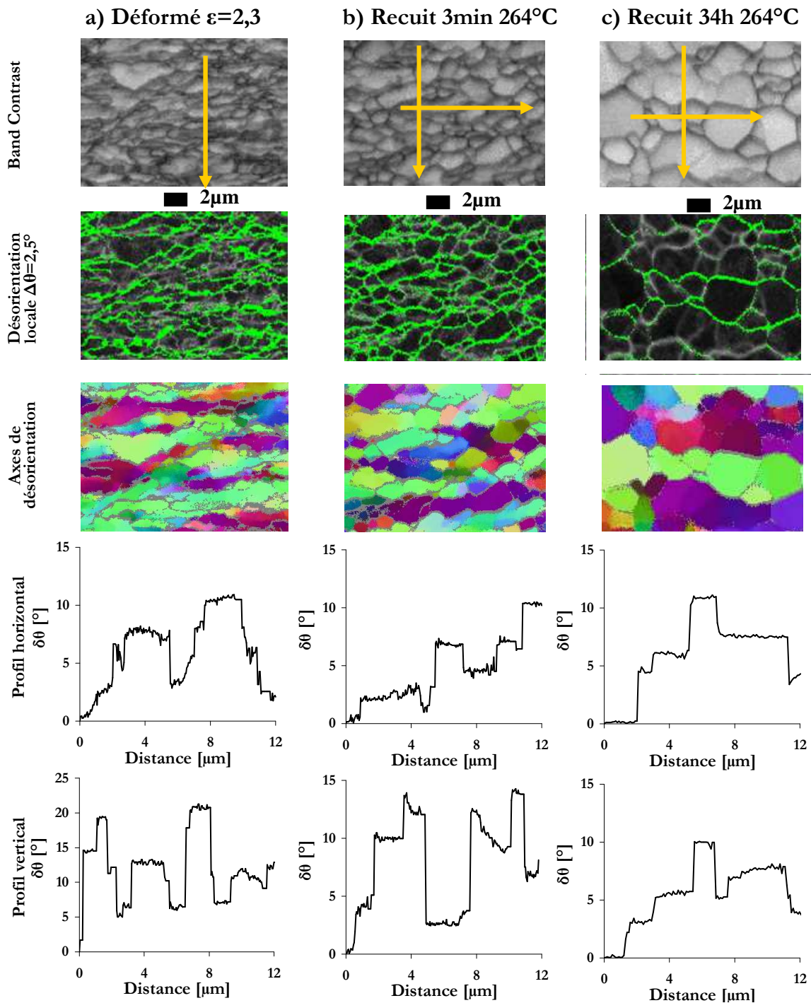
Figure V-8 : Monocristaux Goss déformé ( \epsilon=2,3 ) et recuits 3min et 34h à 264^\circ\text{C} : voir détails de la légende de la Figure V-6. (pas de 0,05\mu\text{m} pour a-b) et de 0,1\mu\text{m} pour c) ).
