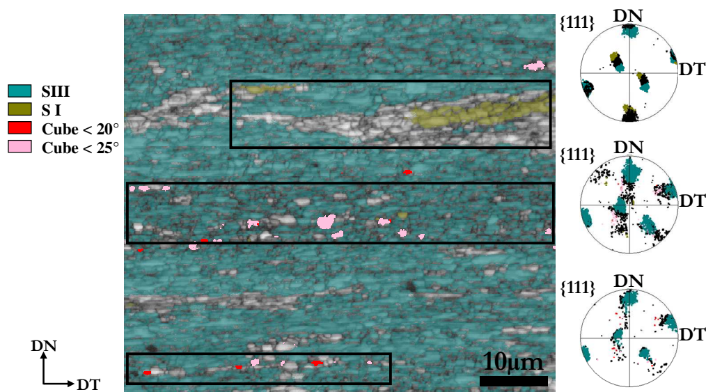
Figure IV-11 : Hétérogénéités de déformation d'un monocristal S Al-0,1%Mn déformé à ( \epsilon = 2,3 ) (Cartographie EBSD du Band Contrast associé aux textures avec un pas de 0,1µm).
