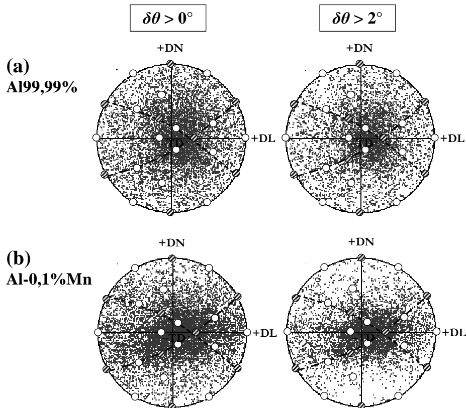
Figure IV-20 : Projection stéréographique des axes de désorientations des monocristaux Al99,99% (a) et Al-0,1%Mn (b) déformés en grande déformation ( \varepsilon = 2,3 ).
