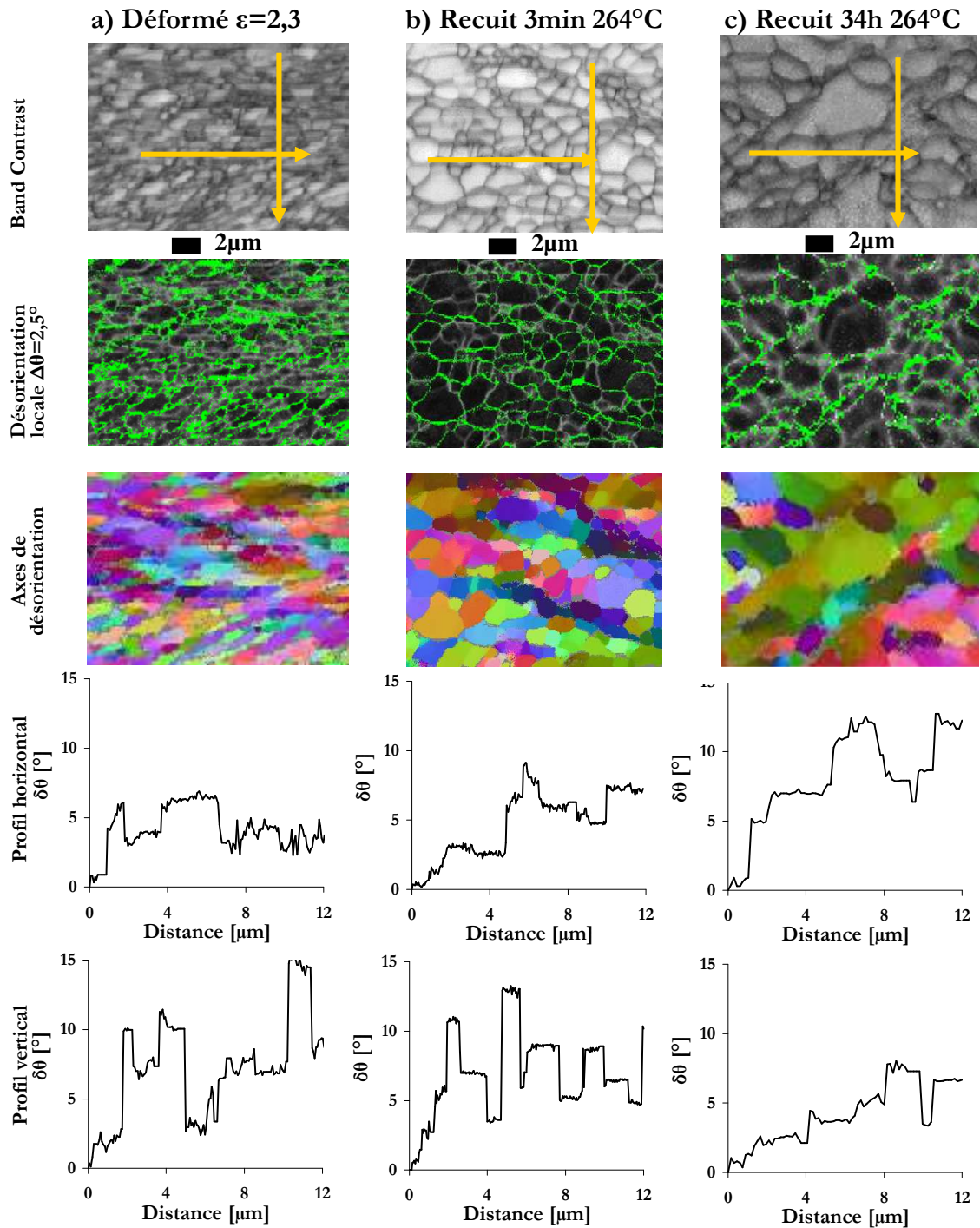
Figure V-9 : Monocristaux S déformé ( \epsilon=2,3 ) et recuits 3min et 34h à 264^\circ\text{C} : voir détails de la légende de la Figure V-6. (pas de 0,05\mu\text{m} pour a-b) et de 0,15\mu\text{m} pour c) ).
