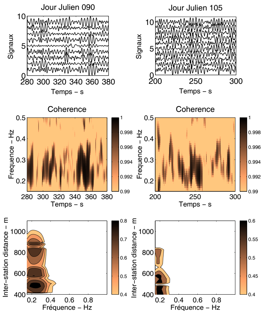
FIG. 5.17 – Exemple de signaux enregistrés dans la tranche horaire 15h00-16h00 TU pour les jours 090 (sec) et 105 (mouillé). Les deux séries de figures du bas correspondent à la cohérence moyenne dans le domaine temps-fréquence pour les portions de signal temporel représentées ici (paramètres de calcul précisés dans le texte) et à la cohérence en fonction de la fréquence et de l'espacement intercapteur (cohérence calculée sur 1h00). Les valeurs de cohérence ne sont valables qu'au delà de 0.2 Hz.
