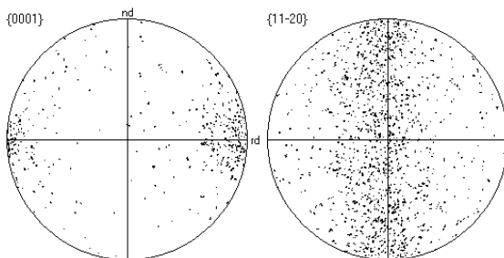
Figure 6.16 : figure de pôles simulée, 10%, modèle de Taylor FC, CRSS = 1\ 2\ 8\ 3\ 4\ 7\ 8
