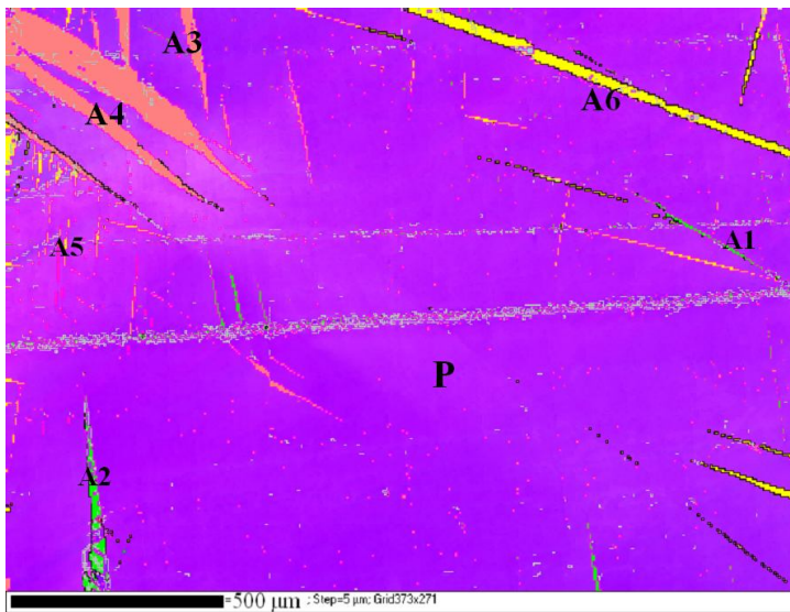
(a) Carte de (88 75 34) déformé de 0.123 à 250°C
