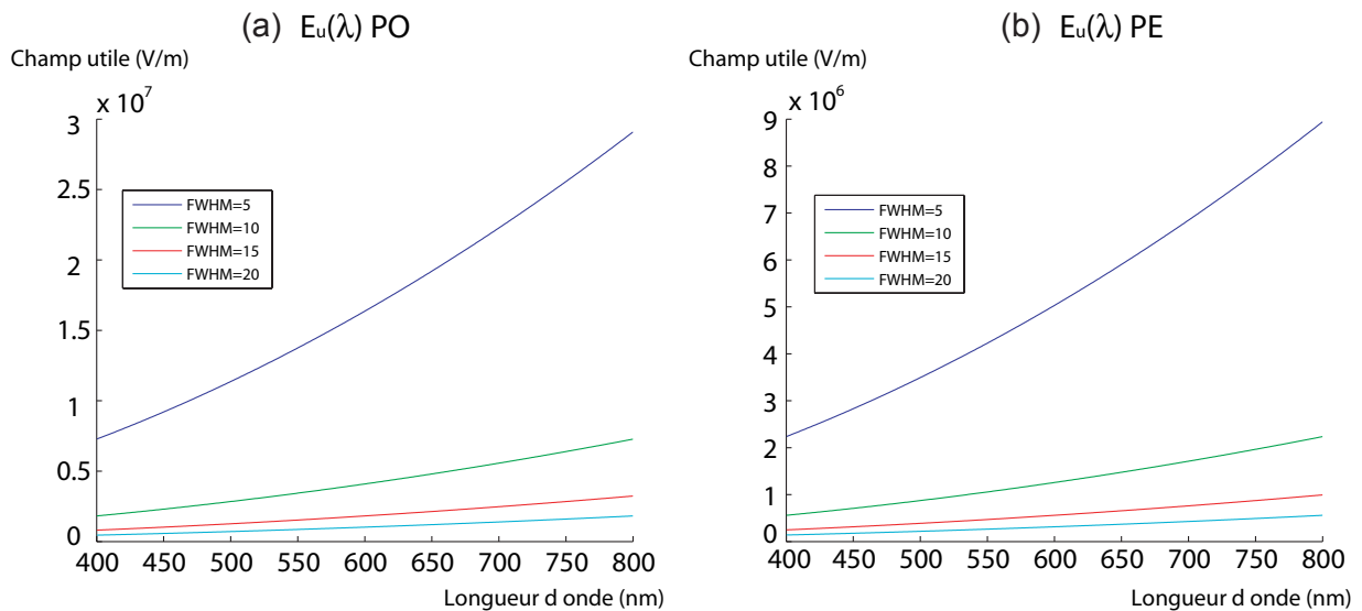
FIGURE 4.38 – Evolution du champ utile E_u pour générer des soliton de taille ( 5\mu\text{m} , 10\mu\text{m} , 15\mu\text{m} et 20\mu\text{m} ) en polarisation ordinaire (a) et une polarisation extraordinaire (b) dans le LN en fonction de la longueur d'onde d'induction
