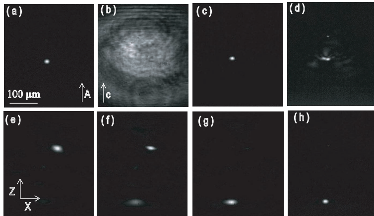
FIGURE 5.5 – Dynamique d'auto-déviaton pyroélectriques d'un faisceau laser de polarisation extraordinaire dans un échantillon de LN stoechiométrique. (a) Spot d'entrée, (b) diffraction, (c) maximum de focalisation, (d-f) dynamique de courbure et (e) refocalisation de faisceau.
