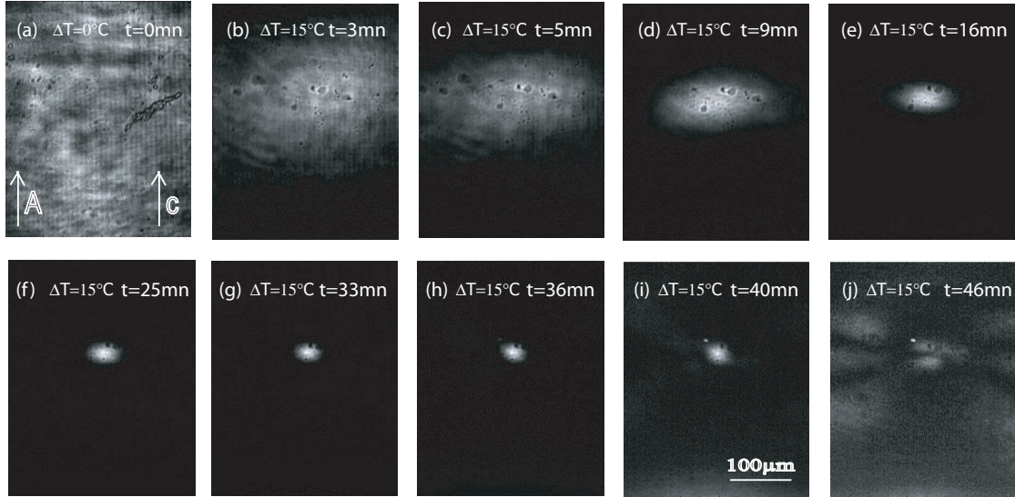
FIGURE 3.4 – Dynamique de l'autofocalisation pour une polarisation extraordinaire de l'onde optique A du faisceau laser \lambda = 532nm par effet photoréfractif dans un cristal de LN dont la température a été augmentée de 15°C par rapport à la température d'équilibre.
