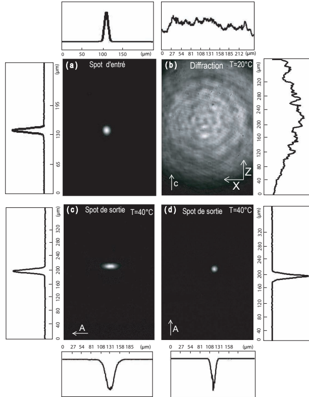
FIGURE 4.10 – Comparaison de l'auto-focalisation dans un cristal de LN de 17mm de long en fonction de la polarisation optique. (a) spot d'entrée (13 \mu m FWHM), (b) diffraction, (c) focalisation en polarisation ordinaire et (d) focalisation en polarisation extraordinaire. Paramètres : LN congruent X \times Y \times Z = 8\text{mm} \times 17\text{mm} \times 0.5\text{mm} , P = 80\mu\text{W} et \Delta T = 20^\circ\text{C} .
