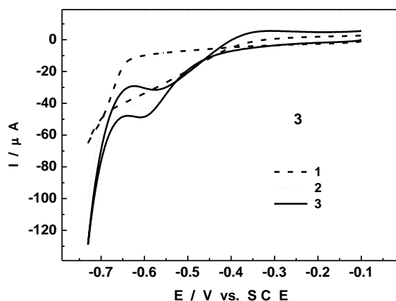
Figure II-5: Voltammogrammes cycliques répétés de {3} dans 1 M CH 3 COOLi/H + pH 5,9. Concentration: 4 \times 10^{-5} M. Electrode de travail: carbone vitreux. Electrode de référence: SCE. Vitesse de balayage: 2 \text{ mV s}^{-1} .
