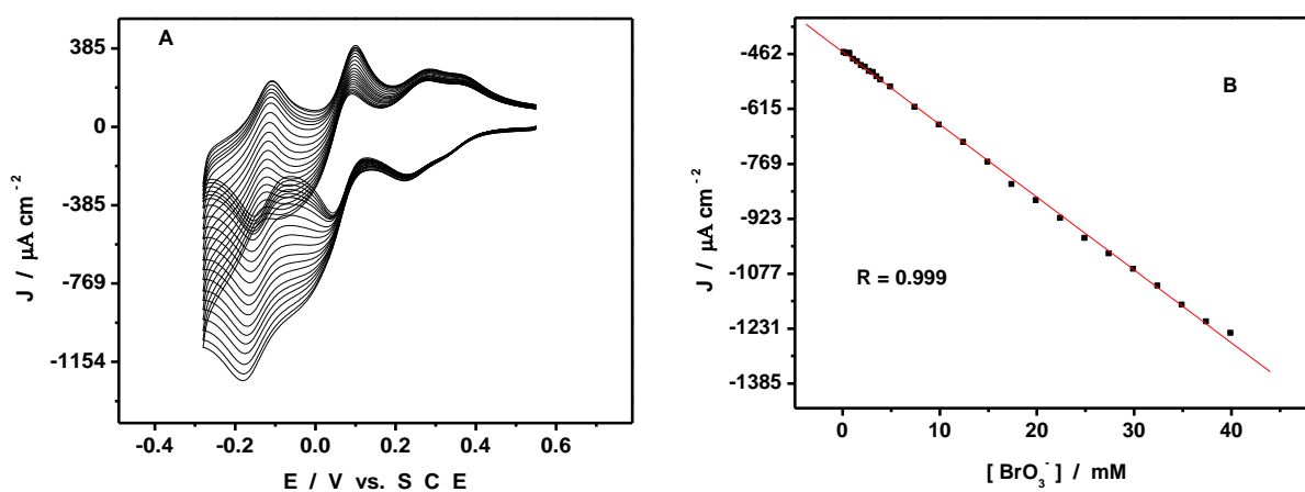
Figure V-10: (A) CVs de Z-POMOF1-PVAE dans 1 M LiCl/ HCl pH 2 en absence et en présence de bromate. (B) Variation de l'intensité du courant de pic de la troisième vague de réduction en fonction de la concentration en bromate; v = 50 \text{ mV s}^{-1} . Electrode de référence: SCE.
