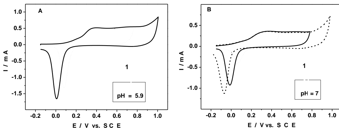
Figure IV-14: CVs de {1} limités à la zone de formation d'oxydes de palladium et de leur réduction. Concentration: 2 \times 10^{-4} M. Electrode de référence: SCE ; v = 10 \text{ mV s}^{-1} . Milieu acétate: (A) pH = 5,9; (B) pH = 7,0.
