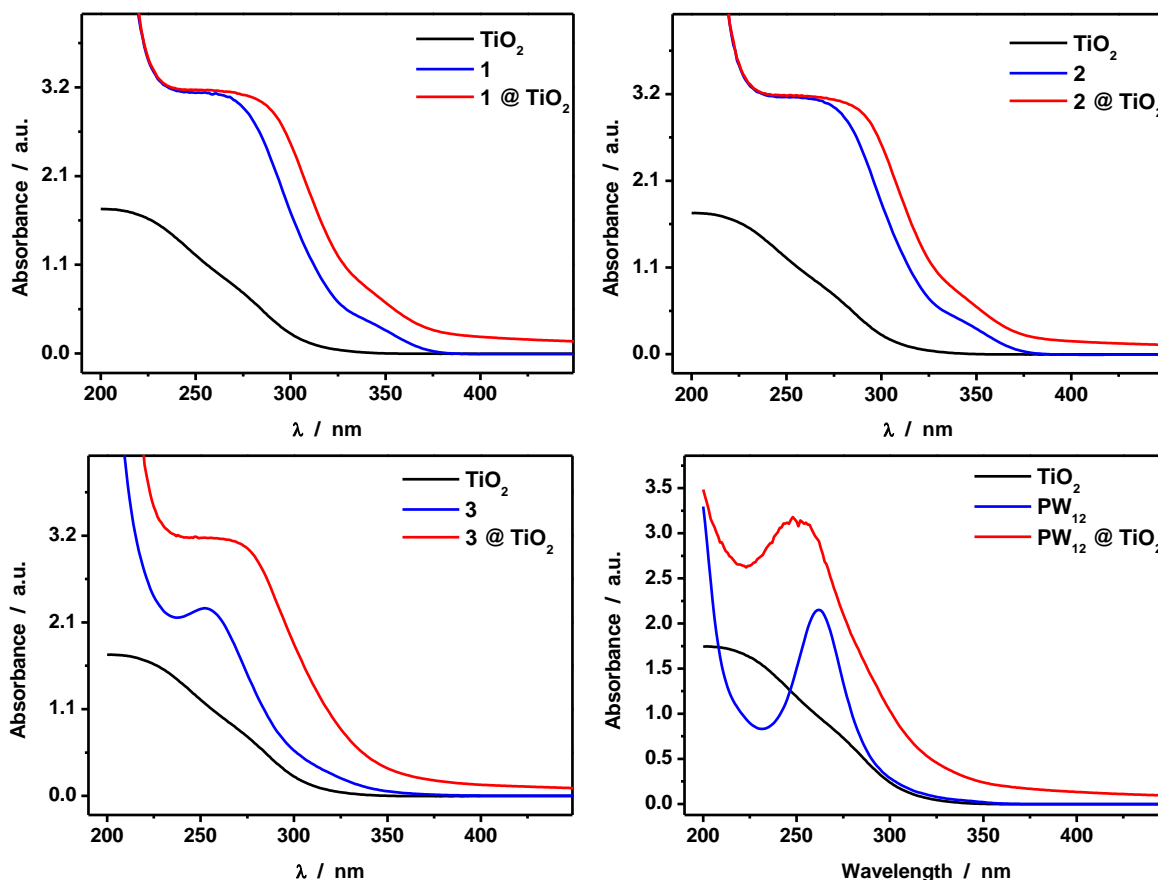
Figure V-18: Comparaison des spectres UV des POMs en absence et en présence de TiO 2 dans 0,1 M HCl (pH 1). Le spectre de TiO 2 est ajouté pour comparaison. [POM] = 0,05 mM, [TiO 2 ] = 0,38 mM.
