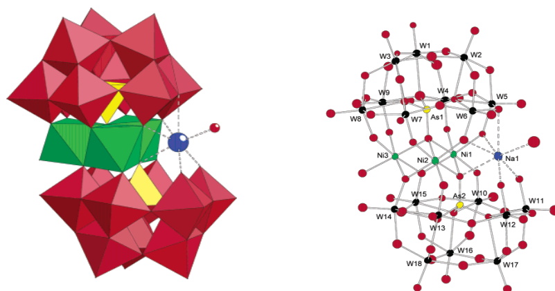
Schéma II-12: (A) Représentation en boules/bâtons et polyédrale de {2}. Les polyèdres AsO 4 , WO 6 et NiO 6 sont respectivement jaune, rouge et vert. Na, boule bleu; la molécule d'eau terminale est en boule rouge. (B) Représentation en boules et bâtons de {2}.
