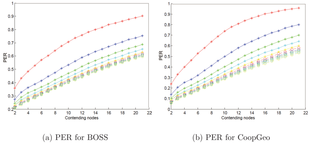
FIGURE C.3 – PER de BOSS et CoopGeo avec T_{max} = 100\dots 1000 \mu s . Les courbes situées dans la partie inférieure du graph correspondent à T_{max} = 100 et celles situées dans la partie supérieure correspondent à la valeur maximale T_{max} = 1000
