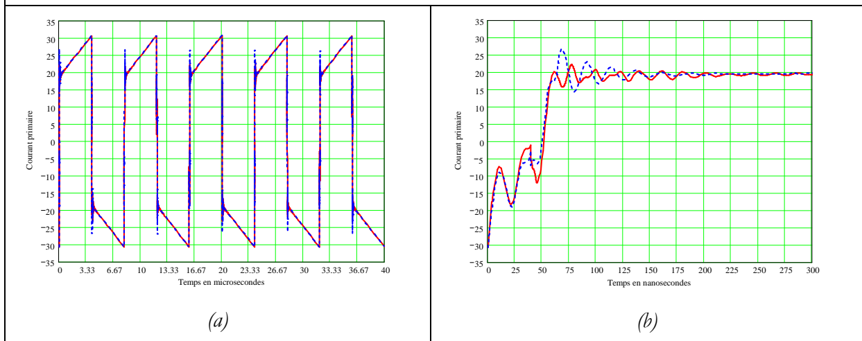
Fig. 2.49 - (a) Courant primaire : circuit réduit (bleu) et circuit complet (rouge) – (b) Zoom sur les oscillations sur un front montant
