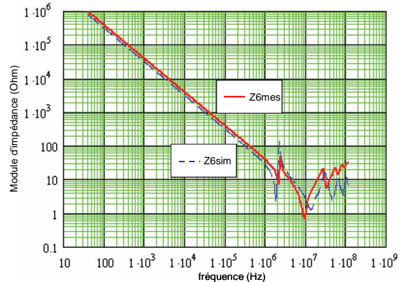
Fig. 5.9 - Comparaison modèle-mesure d'impédances inter-primaires à gauche : secondaire à vide, à droite : secondaire en court-circuit
