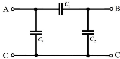
Fig. 3.21 - Quadripôle capacitif
