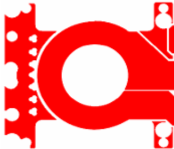
Fig. 2.3 - Forme d'une couche de cuivre d'un transformateur planar
