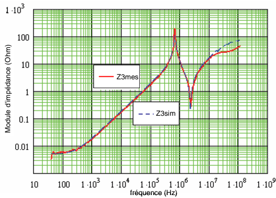
Fig. 5.8 - Comparaison modèle-mesure des modules d'impédances à vide (à gauche) et en court-circuit (à droite) vues du secondaire
