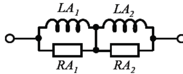
Fig. 2.20 - Circuit équivalent à l'impédance \mathcal{A}
