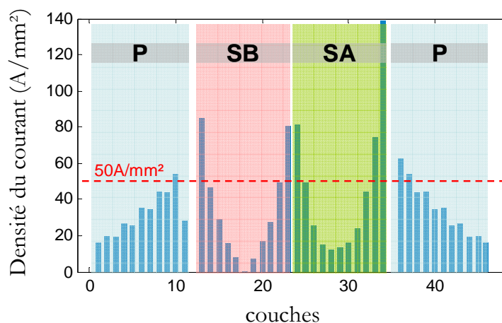
Fig. 4.18 - densité du courant dans les spires et la limite imposée par le cahier des charges ( 50\text{A}/\text{mm}^2 )
