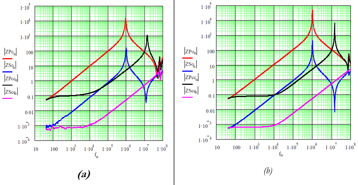
Fig. 2.38 - Comparaison des modules des impédances mesurées (a) et simulées (b) du transformateur 38 couches
