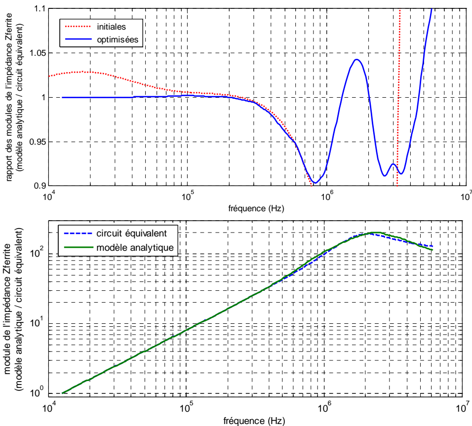
Fig. 4.41 - comparaison entre le module de l'impédance Z_{\text{ferrite}} calculée avec les données constructeur et celle du circuit équivalent
