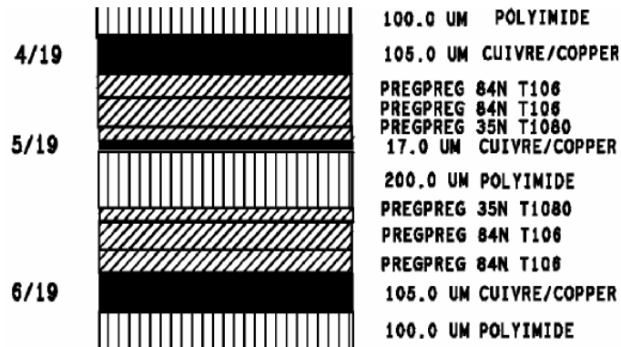
Fig. 2.4 - Arrangement des isolants d'un transformateur planar
