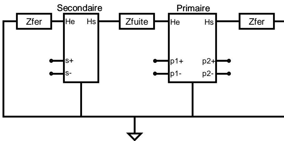
Fig. 5.4 - Schéma équivalent couplage primaire-secondaire du LCT
