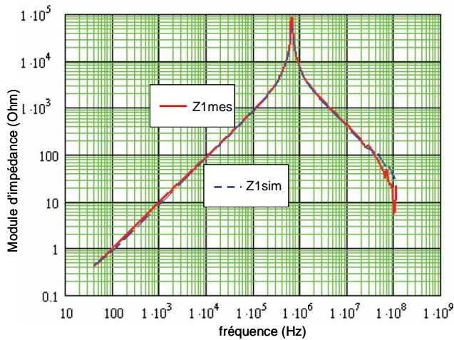
Fig. 5.7 - Comparaison modèle-mesure des modules d'impédances à vide (gauche) et en court-circuit vues d'un primaire
