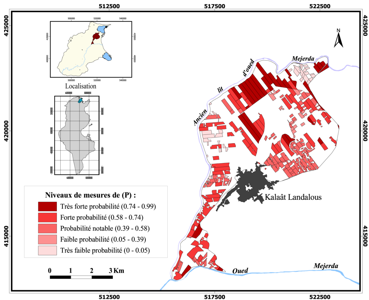
ill. n°130 : Répartition des niveaux de probabilités pignistiques pour l'hypothèse "sols nus à peu couverts" (hiver 2008-2009).
