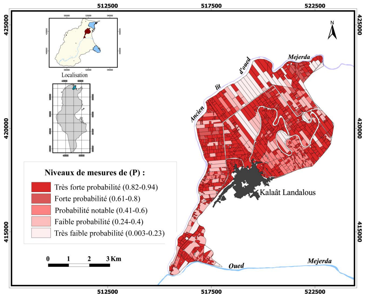
ill. n°129 : Répartition des niveaux de probabilités pignistiques pour l'hypothèse "sols couverts" (hiver 2008-2009).
