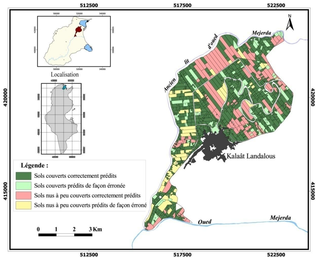
ill. n°131 : Croisement de la vérité terrain de l'hiver 2008-2009 avec la carte de prédiction pour les hypothèses "sols couverts" et "sols nus à peu couverts".
