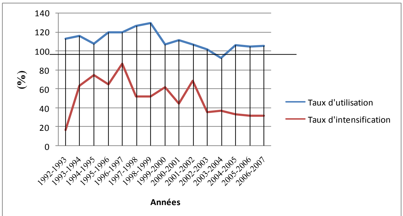
ill. 126 : Taux d'utilisation et d'intensification des sols dans le périmètre public irrigué de Kalaât Landalous (C.T.V. de Kalaât Landalous, 2009)
