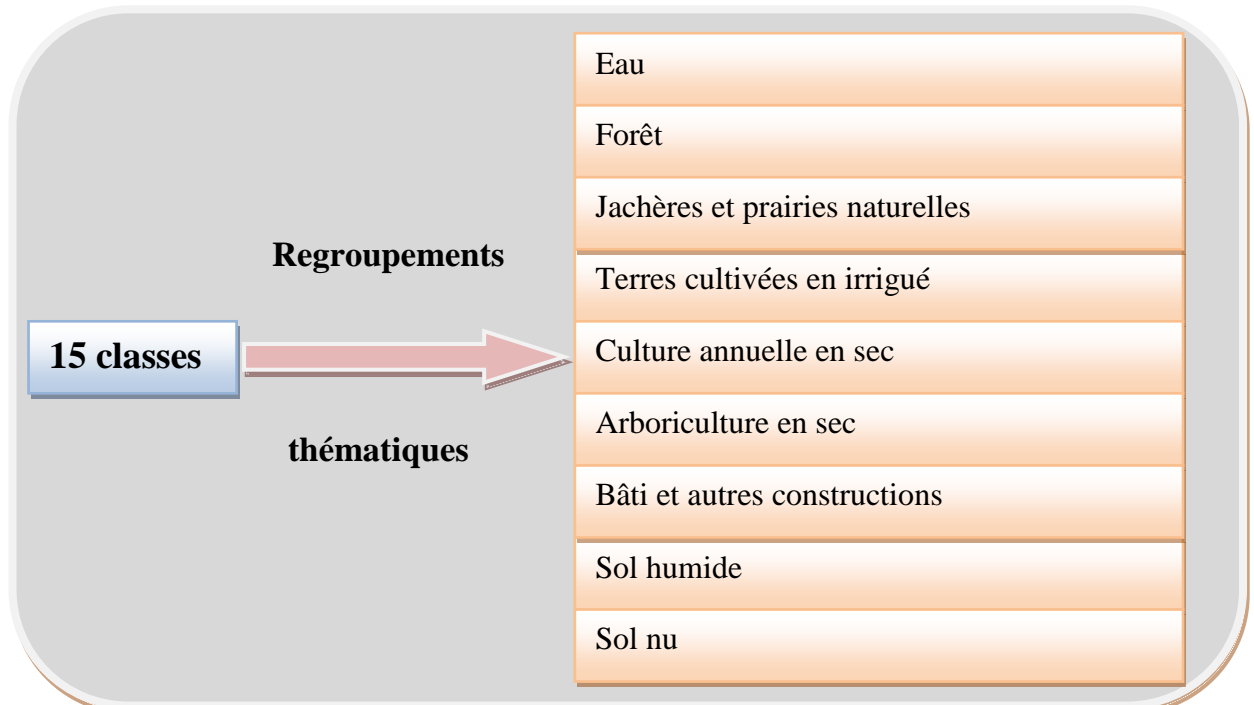
ill. n°32 : Nomenclature retenue après regroupements thématiques opérés sur la classification supervisée par "maximum de vraisemblance".
