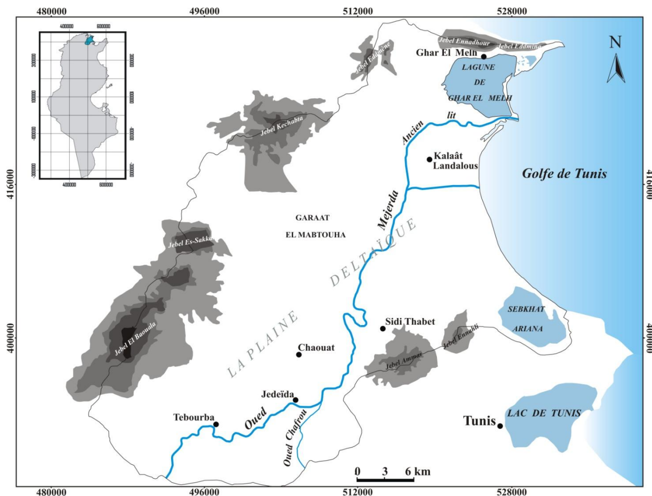
ill. n°9 : Localisation géographique des Jebels limitant le delta de Mejerda.
