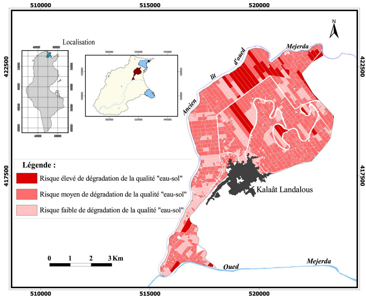
ill. n°133 : Risques de dégradation de la qualité "eau-sol", déterminés à partir des occurrences "sol nu à peu couvert" pour les hivers de la période 2009-2013.
