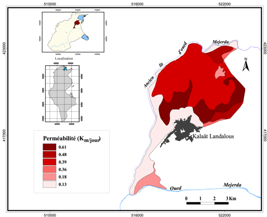
ill. n° 118 : La perméabilité des sols de la plaine de Kalaât Landalous (CRDA de l'Ariana, 2009)
