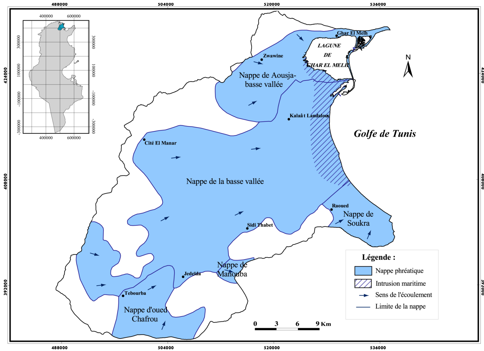
ill. n°19 : Les nappes phréatiques du delta de Mejerda. (Elaboration personnelle à partir des données des CRDA du Grand Tuneset Ministère de l'Agriculture & AHT, 1998)
