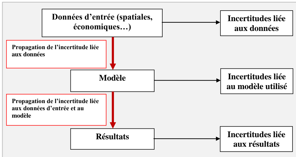
ill. n°115 : Prise en compte de l'incertitude dans un processus de modélisation d'un phénomène (CORGNE S., 2004)
