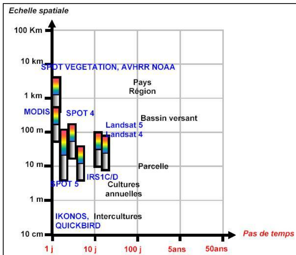
ill. n°26 : Représentation schématisée des échelles de temps et d'espaces auxquels les modes d'occupation et d'utilisation des sols sont étudiés par la télédétection (d'après HUBERT-MOY L et al. , 2001 )
