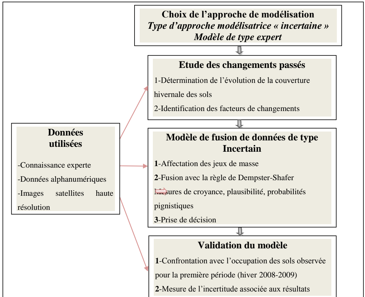
ill. n°122 : Méthodologie du processus de modélisation prédictive de la couverture hivernale des sols appliquée sur le périmètre irrigué de Kalaât Landalous (inspirée des travaux de CORGNE S., 2004).
