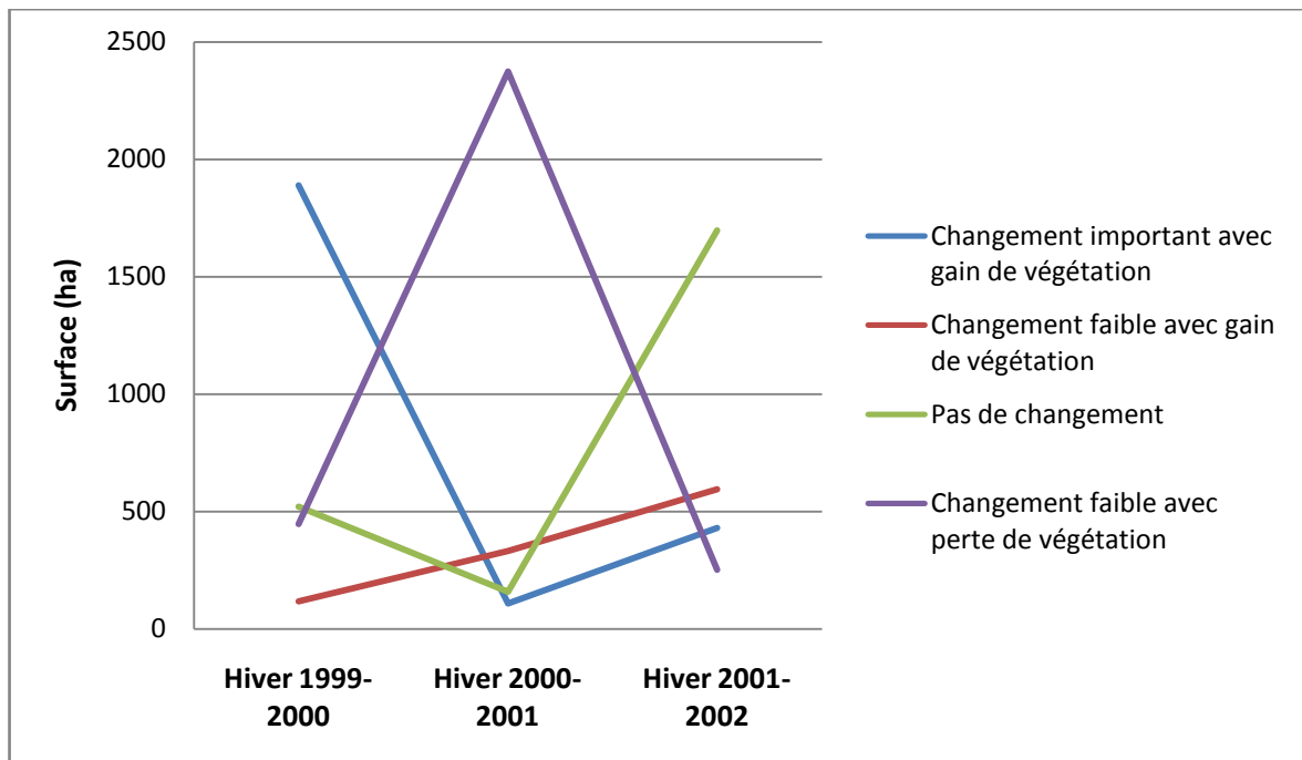
ill. n°124 : Evolution des niveaux de changement de couverture des sols entre les hivers étudiés (1999-2002).
