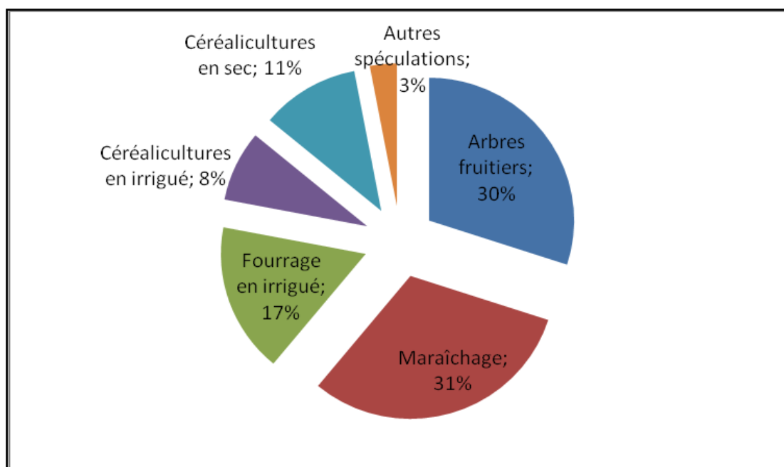
ill. n°79 : Occupation du sol dans les périmètres irrigués du delta de Mejerda en 1974 (Photographies aériennes 1974)
