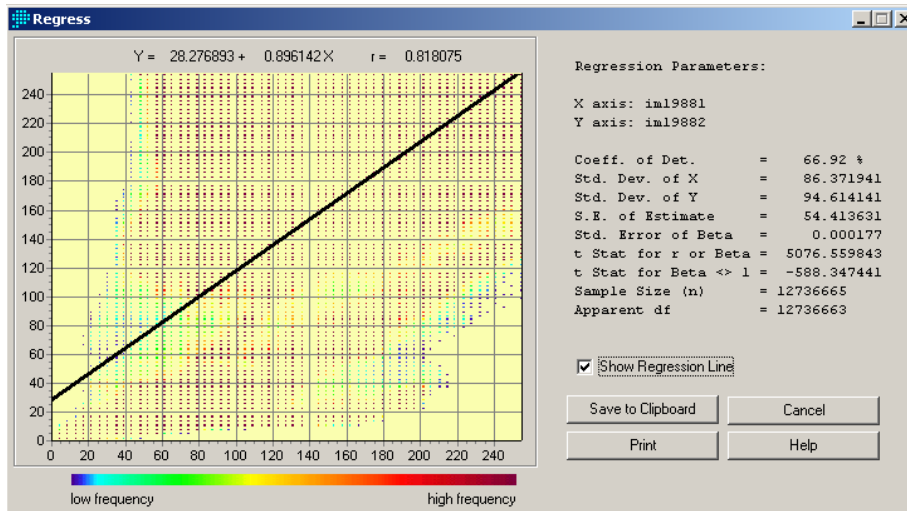
ill. n°9 : Une décorrélation forte entre les bandes XS1/XS2 de l'image 1988.
