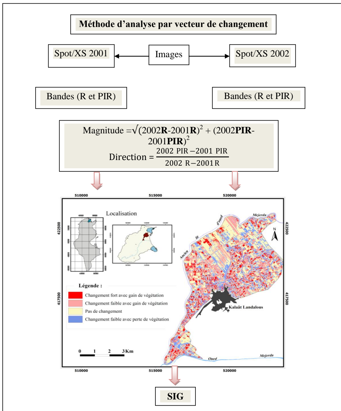
ill. 123 : Méthodologie de l'analyse des vecteurs de changements (AVC) calculés entre deux hivers (inspirée des travaux de CORGNE S., 2004)
