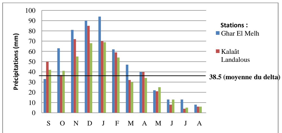
ill. n°11 : Diagramme des moyennes des précipitations mensuelles entre 1987 et 2004, dans quelques stations du delta de Mejerda (DGRE, 2006).
