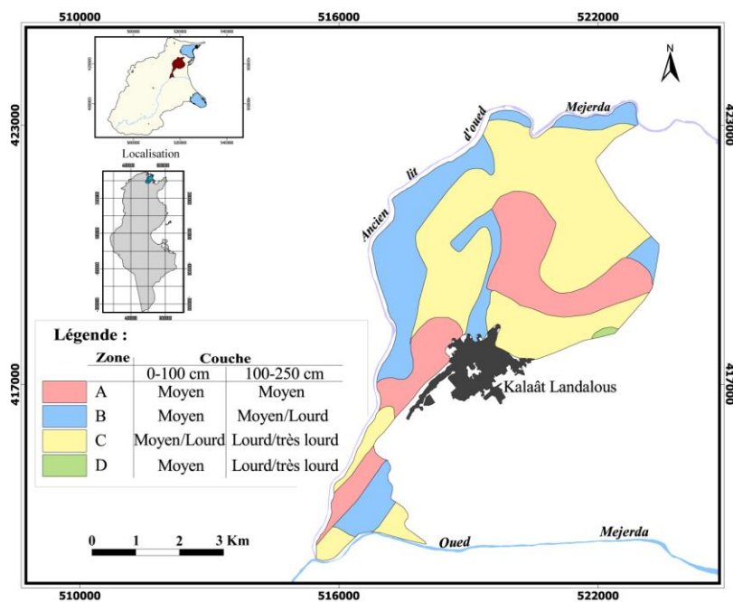
ill. n°117 : Les unités texturales de la plaine de Kalaât Landalous (Carte des textures au 1/50000, secteur de Kalaât Landalous)
