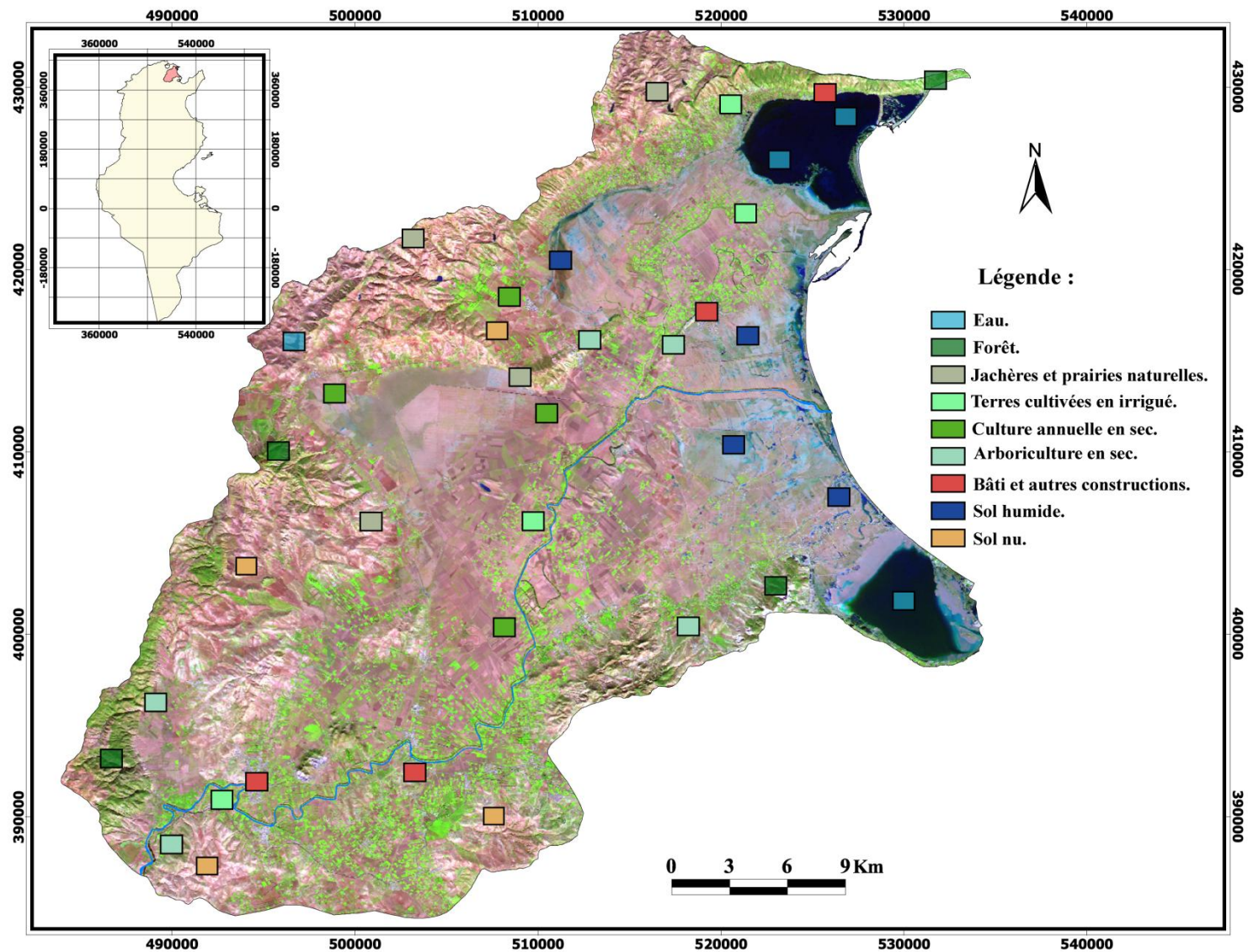
ill. n°29 : Localisation des zones "teste" pour l'établissement de la classification supervisée (image Spot/XS de 1999, ISIS-CNES©) (Les zones tests choisies pour l'image de 1988, ont été modifiées légèrement en fonction du changement de l'état phénologique de la végétation).
