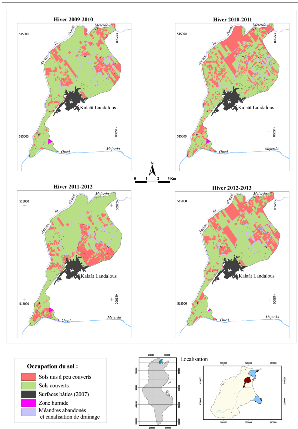
ill. n°132 : Prédiction de l'évolution des couvertures hivernales du sol dans le périmètre irrigué de Kalaât Landalous (2009-2013).
