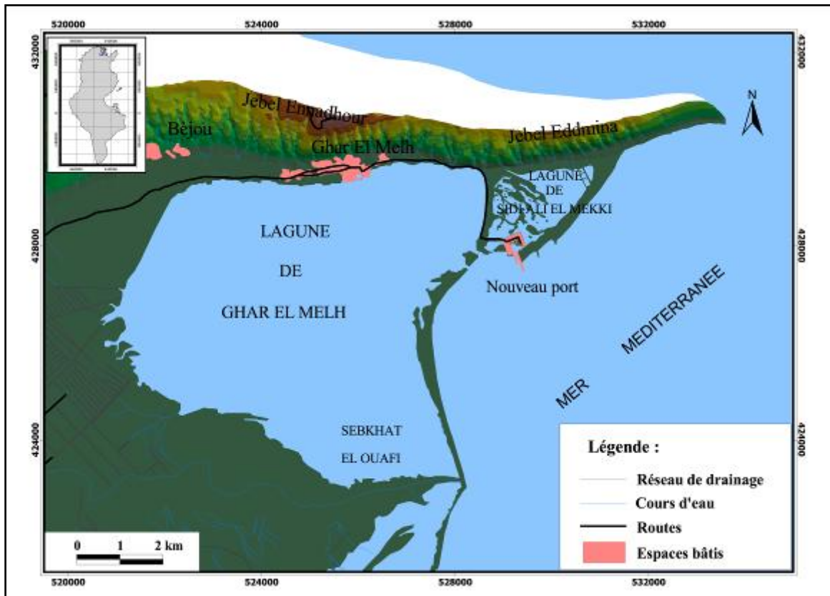
ill. n° 61 : Le complexe lagunaire de Ghar El Melh : Localisation et délimitation (Modèle Numérique d'Altitude, carte topographique de Ghar El Melh N.E. au 1/25000)
