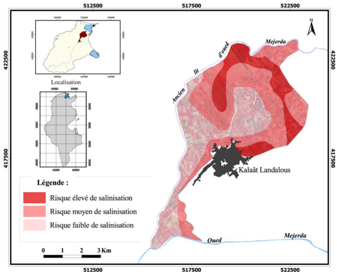
ill. n°120 : Les zones à risque de salinisation dans la plaine de Kalaât Landalous (HACHICHA M. et al. , 1997 : document modifié), (image de fond : Spot/XS 2002, ISIS-CNES).
