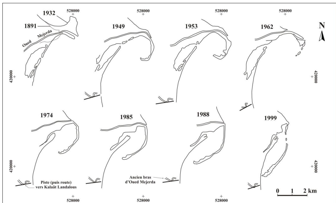
ill. n°53 : La flèche de Fom El Oued : plus d'un demi-siècle d'évolution. (PASKOFF. R, 1978 ; OUESLATI A., 2004 : document repris et modifié)
