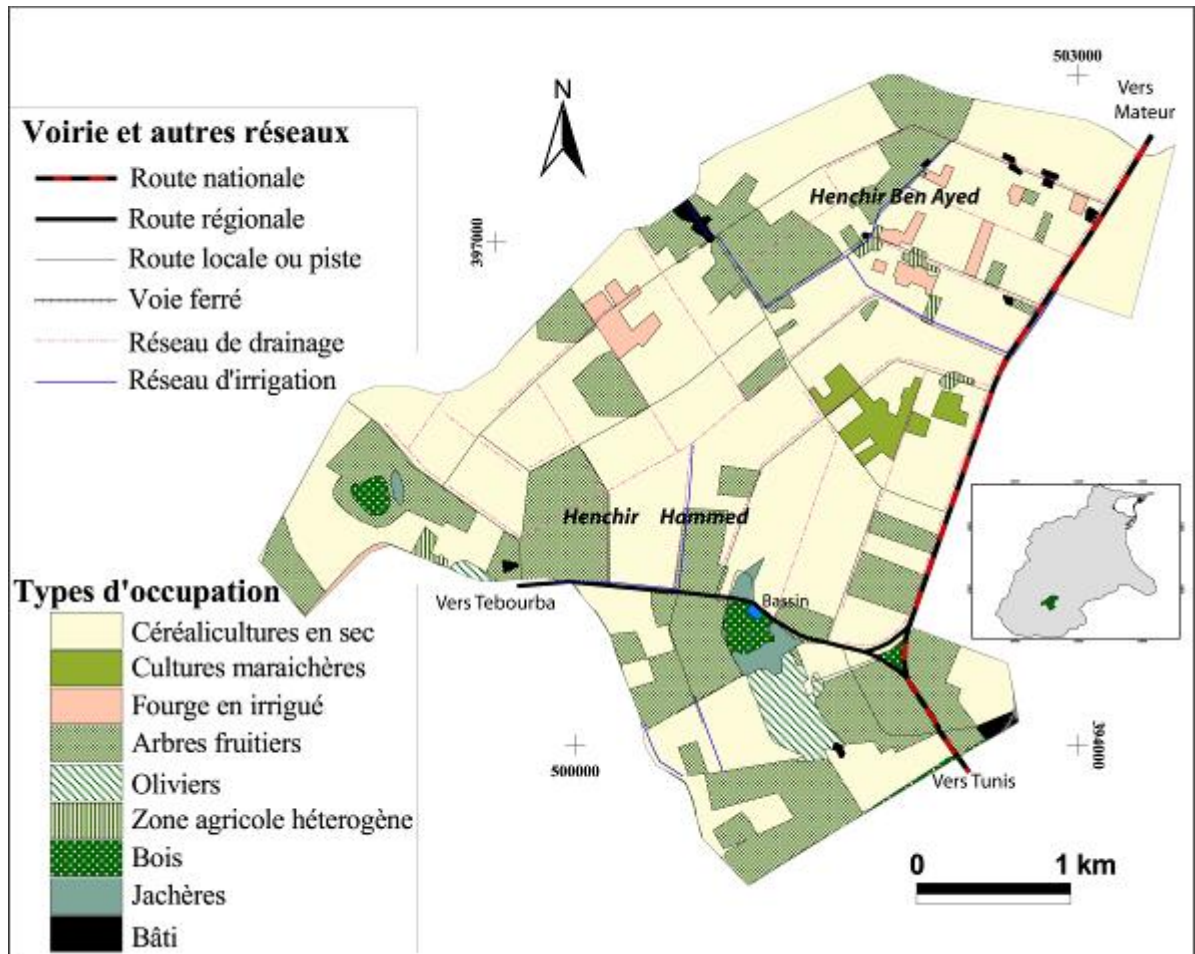
ill. n°88 : L'occupation du sol dans le périmètre irrigué de Hammed en 2007 (extraits d'images Google Earth© 2007).
