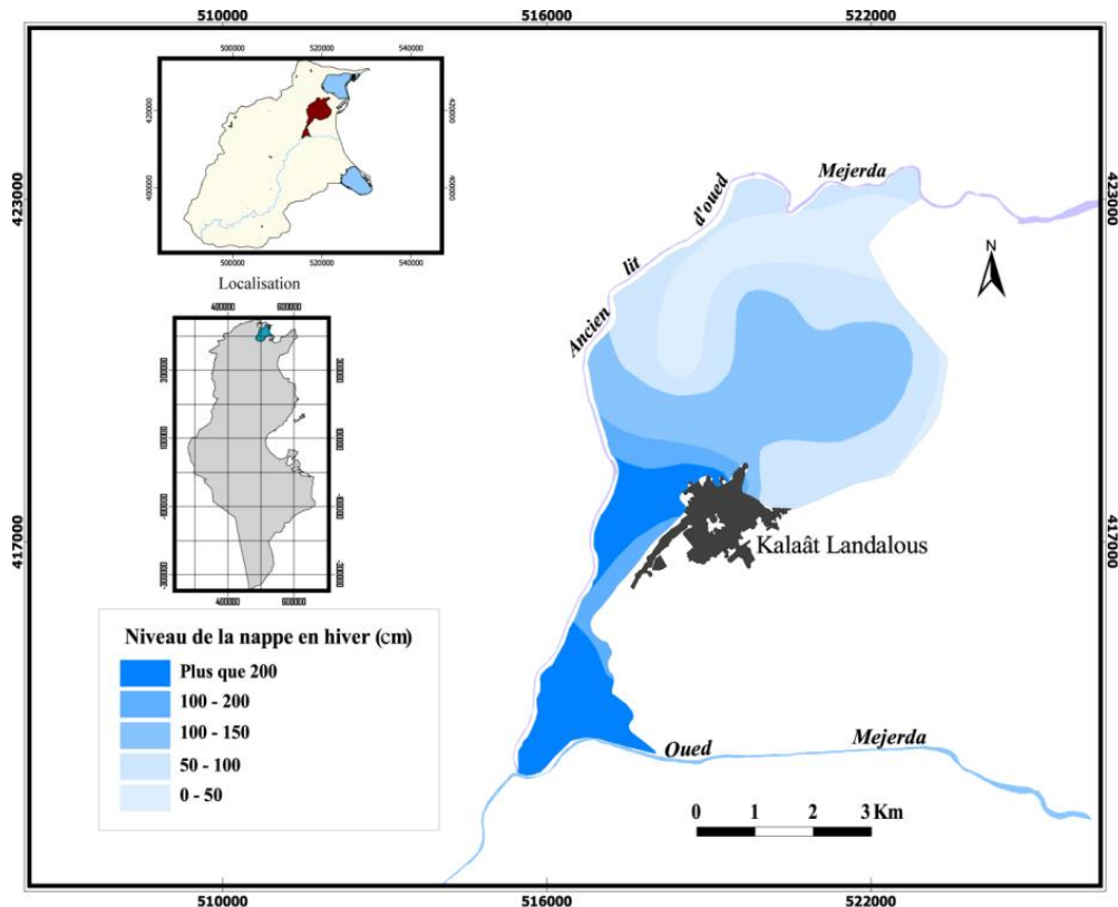
ill. n°119 : Situation de la nappe de Kalaât Landalous en hiver (1990-2002) (CRDA de l'Ariana, 2009)
