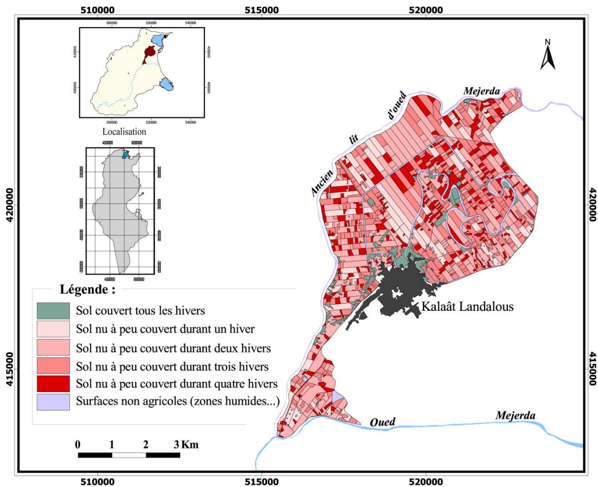
ill. n°128 : Occurrence des "sols nus à peu couverts" pour les hivers étudiés (1999-2002 et 2007-2008) dans le périmètre irrigué de Kalaât Landalous.
