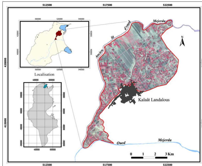
ill. n°116 : Le périmètre public irrigué de Kalaât Landalous : Localisation et délimitation (image Spot/XS 2002, ISIS-CNES)
