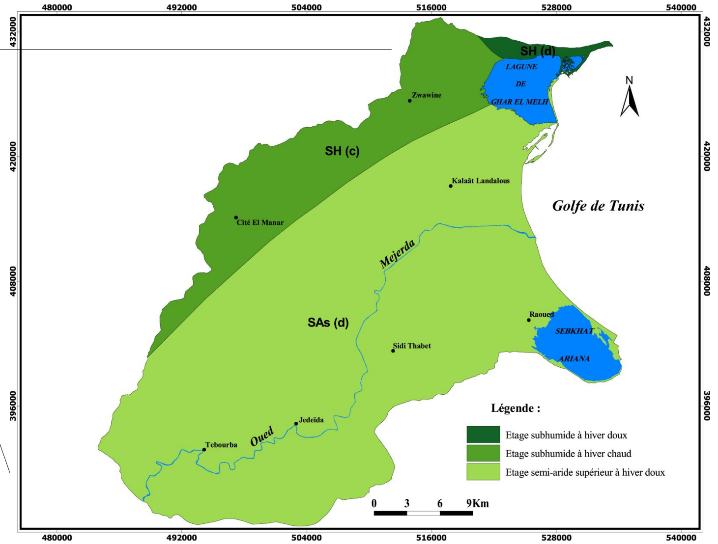
ill. n°16 : Les étages bioclimatiques du delta de Mejerda (d'après GOUNOT M., 1958).
