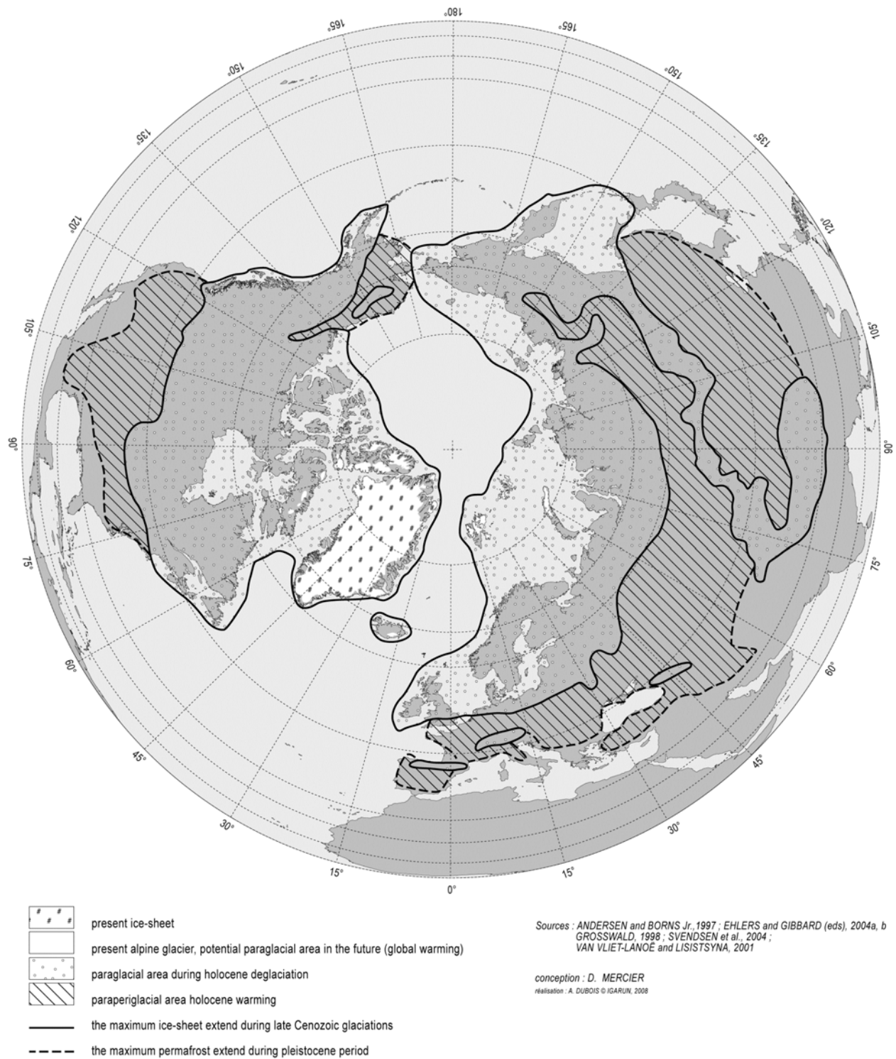
Fig. II.2. Carte du paraglaciaire actif, du paléo-paraglaciaire et du paraglaciaire potentiel (d'après Mercier, 2008e).
