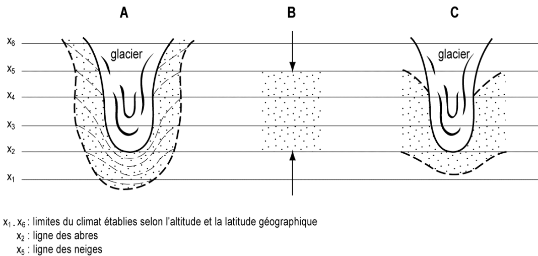
Fig. 1.10. — Les limites de la zone périglaciaire (d'après French, 2007).
