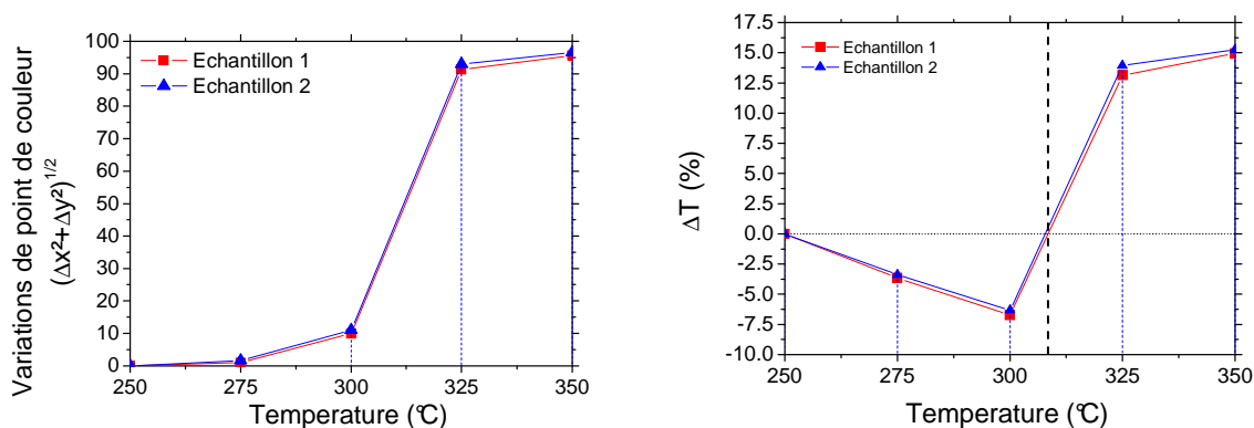
Fig.98 : Variations du point de couleur et de transmission de deux échantillons après recuit cumulé depuis l’élaboration du verre rouge jusqu’à 350°C.
