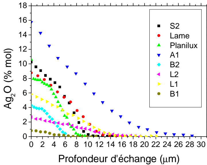
Fig.18 : Profils déterminés au MEB de divers verres échangés dans un mélange composé de 10% AgNO_3 dans NaNO_3 pendant 1 heure à environ 315^\circ C .
