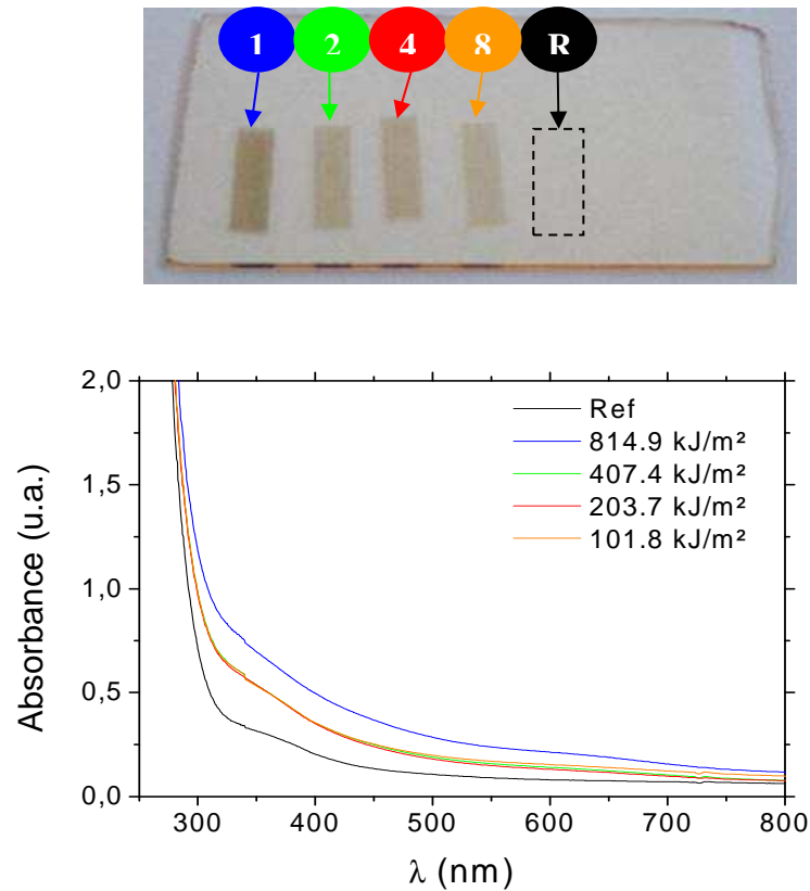
Fig.90 : En haut : photo du verre échangé après irradiation de différentes zones balayées. En bas : spectres d'absorption de l'échantillon échangé dans 10% AgNO 3 -NaNO 3 à T=320°C pendant 10min (Ref). L'échantillon a ensuite été irradié à \lambda=800\text{nm} pour différentes fluences ou vitesses de balayage (0.1 to 0.8mm/s).
