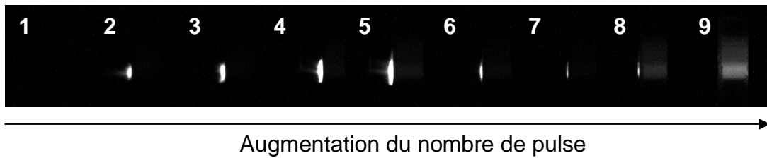
Fig.8b : Echantillon de verre Planilux échangé 10 minutes dans AgNO_3-NaNO_3 puis irradié avec un laser Nd :YAG pulsé à \lambda= 532nm , E=110mJ . Nombre de tirs reçus : 1=280p ; 2= 282p ; 3= 288p ; 4= 307p ; 5=342p ; 6=371p ; 7=395p ; 8=411p ; 9=448p.
