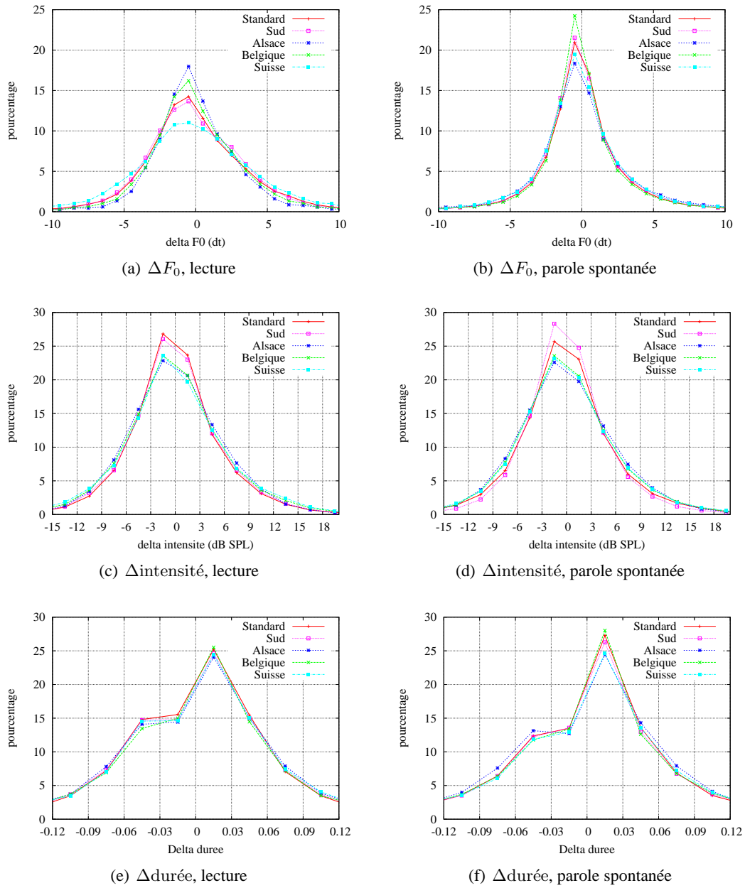
FIGURE 5.2. Répartition des \Delta F_0 (en demi-tons), \Delta intensité (en dB SPL) et \Delta durée (en s) pour le corpus PFC, en lecture et en parole spontanée.
