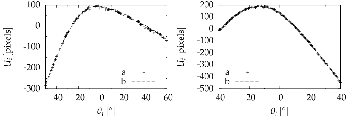
FIG. 5.31: Translation verticale U des images en fonction de l'angle de rotation \theta , pour les séries 20090530-04 (gauche) et 20091107-08 (droite). Aux valeurs calculées par le programme tiltxcorr (a) est superposé l'ajustement par une somme de deux fonctions sinusoidales de périodes respective 2\pi et \pi/2 (b).
