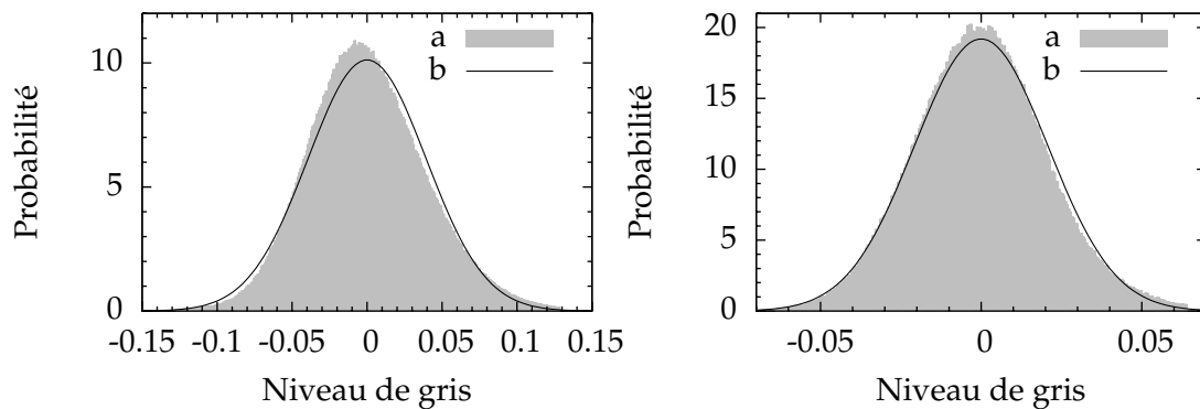
FIG. 5.39: Histogramme des niveaux de gris dans les régions d'intérêt représentées en figure 5.38. Ces histogrammes sont cumulés sur la totalité des images d'une même série. La série 20090530-04 est représentée à gauche, la série 20091107-08 à droite. Sur chaque graphe, la gaussienne (b) de mêmes moyenne et écart-type a été superposée à l'historgramme réel (a).
