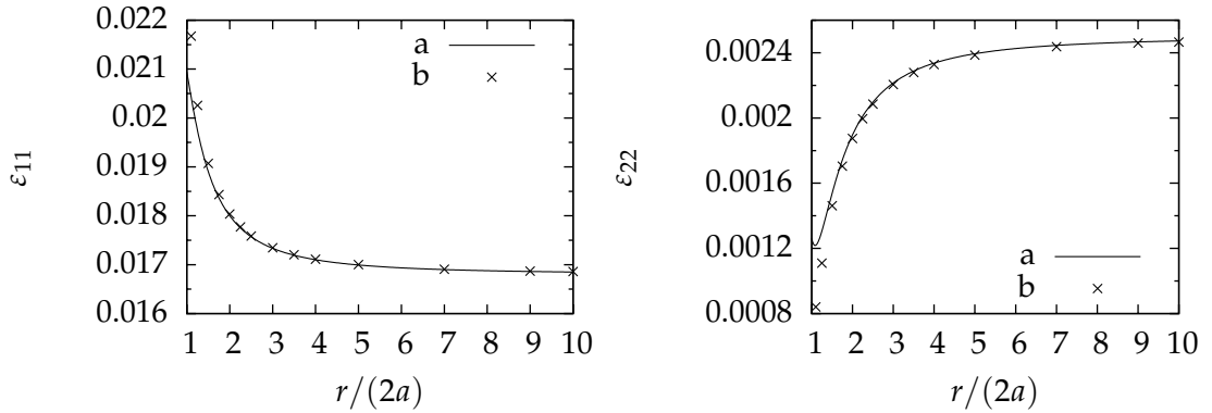
FIG. 2.5: Comparaison des déformations moyennes dans l'inclusion, estimées par polarisation (a) et par éléments finis (b), pour des inclusions raides ( E_i/E_m = 100 ) et une déformation macroscopique \mathbf{E} = \mathbf{e}_1 \otimes \mathbf{e}_1 . A gauche, estimation de \epsilon_{11} ; à droite, estimation de \epsilon_{22} .
