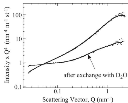
FIG. 4.3: Comparaison des spectres de diffusion obtenus pour une pâte de ciment Portland ordinaire ( w/c = 0.5 ) hydratée, puis saturée en eau ( H_2O ) ou en eau lourde ( D_2O ). Les différences entre les deux spectres caractérisent un milieu multiphasique (extrait de Thomas et coll. , 2004).
