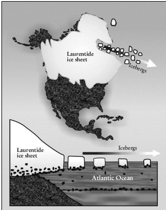
Fig. I-4 : Schématisation d'un évènement de Heinrich (Bard, 2002)
