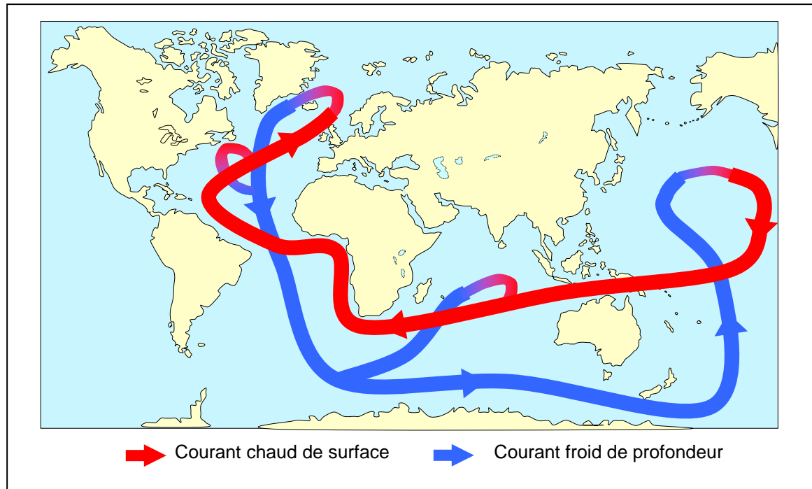
Fig. I-3: La circulation thermohaline (image : http://svt.ac-dijon.fr/schemassvt/article.php3?id_article=982 )
