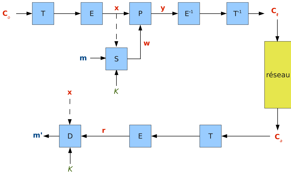
FIGURE 1.2 – Modélisation d'une chaîne de tatouage avec information sous-jacente (la connaissance du contenu hôte x permet d'améliorer la robustesse ainsi que l'imperceptibilité du tatouage [27]).
