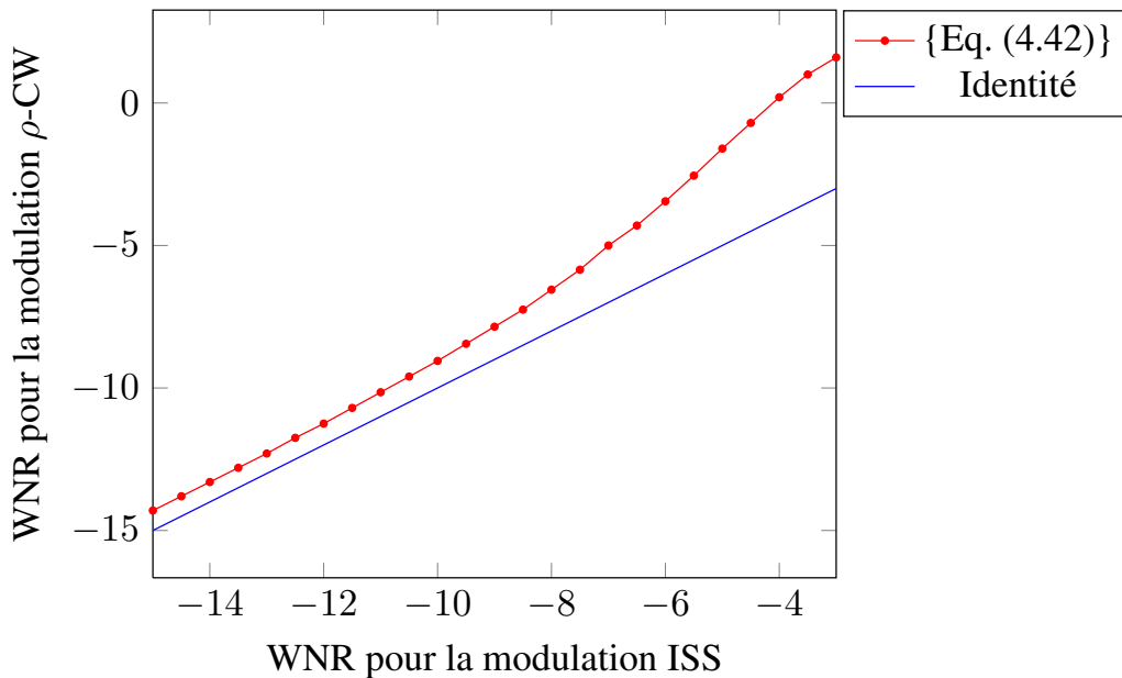
FIGURE 4.11 – WNR pour le \rho -CW (de BER \eta_1 ) en fonction du WNR pour l'ISS (de BER \eta_2 ). Paramètres : N_c = 16 , N_v = 512 , WCR = -10 dB, NCR = -10 dB. La relation entre \eta_1 et \eta_2 est donnée par : R'_s(\theta_{\epsilon WCA}, \epsilon, \eta_1) = R'_s(\theta_{WCA}, 0., \eta_2) . \epsilon = 0.3 est obtenu par ACI avec N_t = 1300 , \rho = 0.04 .
