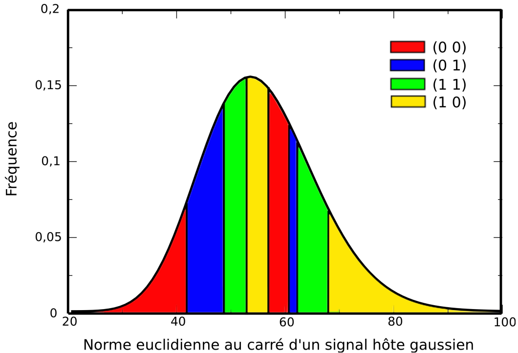
FIGURE 2.6 – Bon exemple de partition secrète pour \chi^2\mathcal{W} . Nous observons une distribution des normes euclidiennes au carré de signaux gaussiens. Ces normes suivent une loi \chi^2(N_v) , N_v = 55 . De plus nous avons N_h = 8 \geq 2^{N_c} = 2^2 = 4 (deux mots de code pour un message). Chaque message apparaît avec la même probabilité mais grâce à la condition donnée par 2.6, les frontières de décodage dépendent d'une clé secrète. L'adversaire ne peut alors déterminer les mots de code, cette construction est stégo-sûre .
