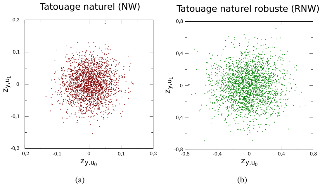
FIGURE 1.14 – Corrélations normalisées entre les signaux tatoués par NW (a) et RNW (b) et deux porteuses secrètes \{\mathbf{u}_0, \mathbf{u}_1\} : sous-espace secret de dimension N_c . Paramètres N_c = 2 , N_v = 512 .
