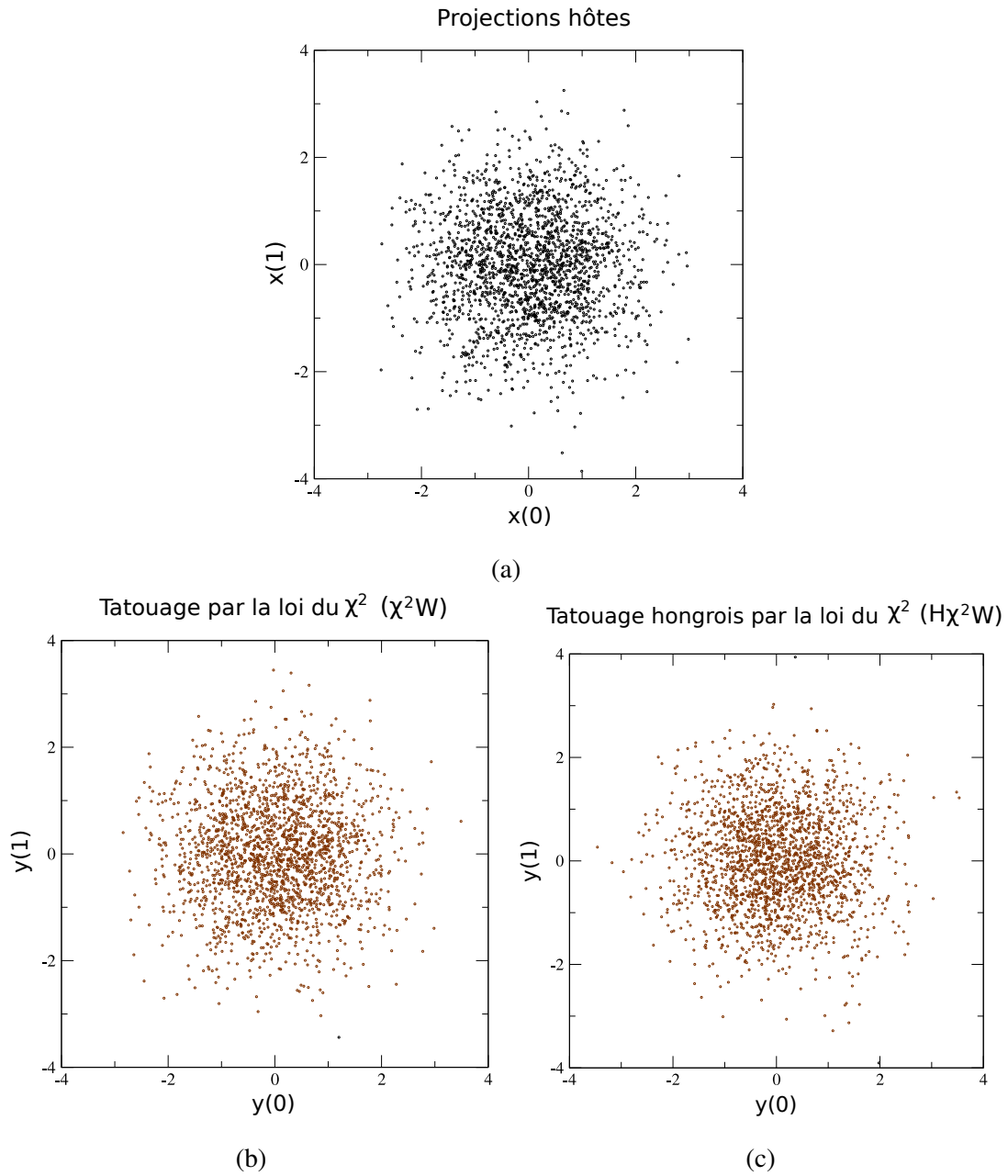
FIGURE 2.18 – (a) : projection des signaux hôtes sur les deux premières composantes des vecteurs. (b) et (c) : projection des signaux tatoués sur les deux premières composantes des vecteurs pour \chi^2W et H\chi^2W .
