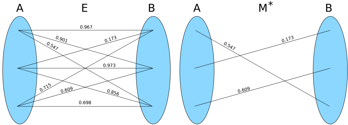
FIGURE 2.11 – Exemple d'un graphe biparti pondéré avec 2 partitions \mathcal{A} et \mathcal{B} de N_m = 3 sommets ainsi que son couplage parfait minimal \mathcal{M}^* (les poids entre deux sommets sont notés sur chaque arête correspondante).
