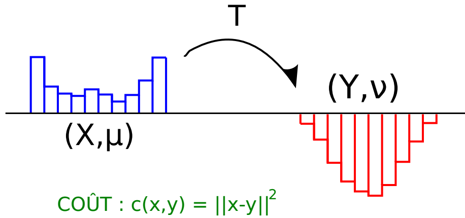
FIGURE 2.20 – Problème du transport : on cherche une bijection T qui minimise le coût total c de déplacement du sable \mathcal{X} de distribution \mu vers les creux \mathcal{Y} de distribution \nu .
