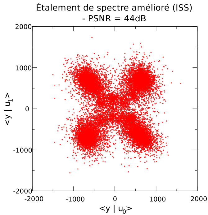
FIGURE 5.7 – Corrélations entre 19800 tuiles ( \equiv 50 images, 2 sec de vidéo) tatouées par ISS et les porteuses secrètes. PSNR = 44 dB.
