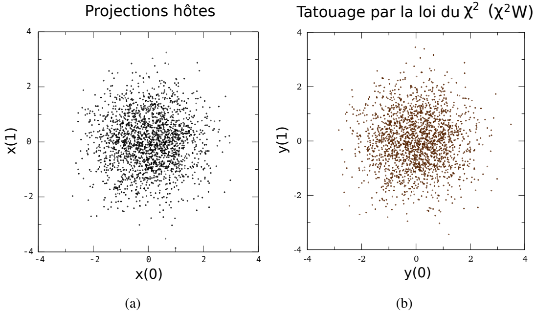
FIGURE 2.8 – Projections sur les deux premières composantes de signaux gaussiens hôtes (a) et tatoués \chi^2W (b) de dimension N_v = 55 . Paramètres : N_c = 2 , N_v = 55 , WCR = -18 dB, N_h = 8 , N_o = 2000 . La distribution des signaux est identique avant et après tatouage, condition suffisante de la stégo-sécurité .
