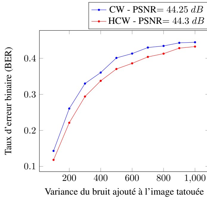
FIGURE 3.18 – Taux d'erreur binaire moyen en fonction de la variance du bruit n ajouté dans le domaine pixelique pour la modulation CW ainsi que son amélioration HCW basée sur une N_m -carte avec une distorsion cible inférieure de façon à obtenir le même PSNR final pour les deux modulations. Nous remarquons la possibilité de convertir le déficit en distorsion qu'offre la méthode basée sur modèle en gain de robustesse lorsque les deux distorsions moyennes finales sont identiques.
