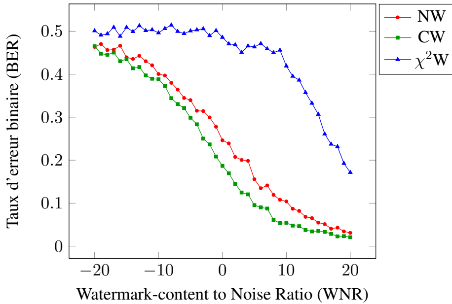
FIGURE 2.9 – BER en fonction du WCNR pour NW, CW et \chi^2W . Pour les trois techniques, nous obtenons : WCR \cong -18 \text{ dB} . La faible robustesse du \chi^2W s'explique par le fait que, pour ce schéma d'insertion, les régions de décodage sont très proches les unes des autres (voir figure 2.4). Par conséquent, un signal tatoué corrompu par l'ajout de bruit aura une plus grande probabilité de basculer dans une autre région de mot de code pour le \chi^2W que pour les méthodes NW et CW.
