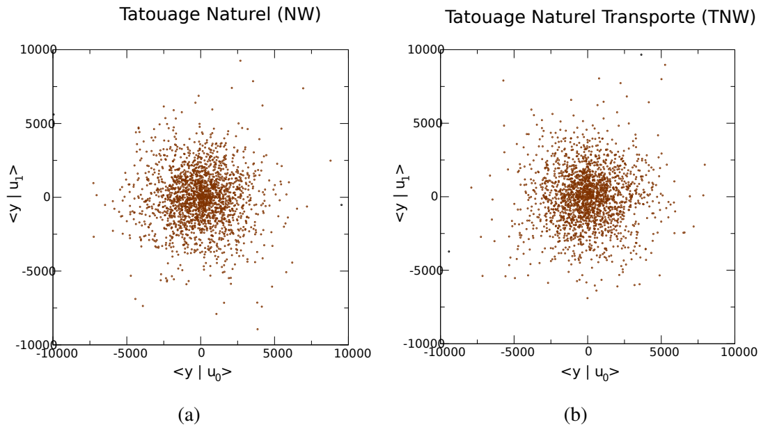
FIGURE 3.11 – Corrélations entre deux porteuses secrètes et 2000 signaux tatoués y pour les modulations NW (a) et TNW (b).
