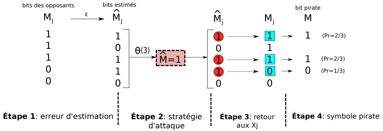
FIGURE 4.6 – Processus d’attaque pour un schéma de tatouage sûr avec c = 5 adversaires et \theta(3) = 1 . Étape 1 : les adversaires estiment trois symboles 1 ( \hat{M}_j ) en parallèle. Étape 2 : nous avons \theta(3) = 1 , la stratégie d’attaque donne \hat{M} = 1 . Étape 3 : la coalition cherche les M_j qui correspondent à \hat{M}_j = \hat{M} = 1 . Étape 4 : le symbole de la séquence pirate M est choisi uniformément parmi les M_j sélectionnés.
