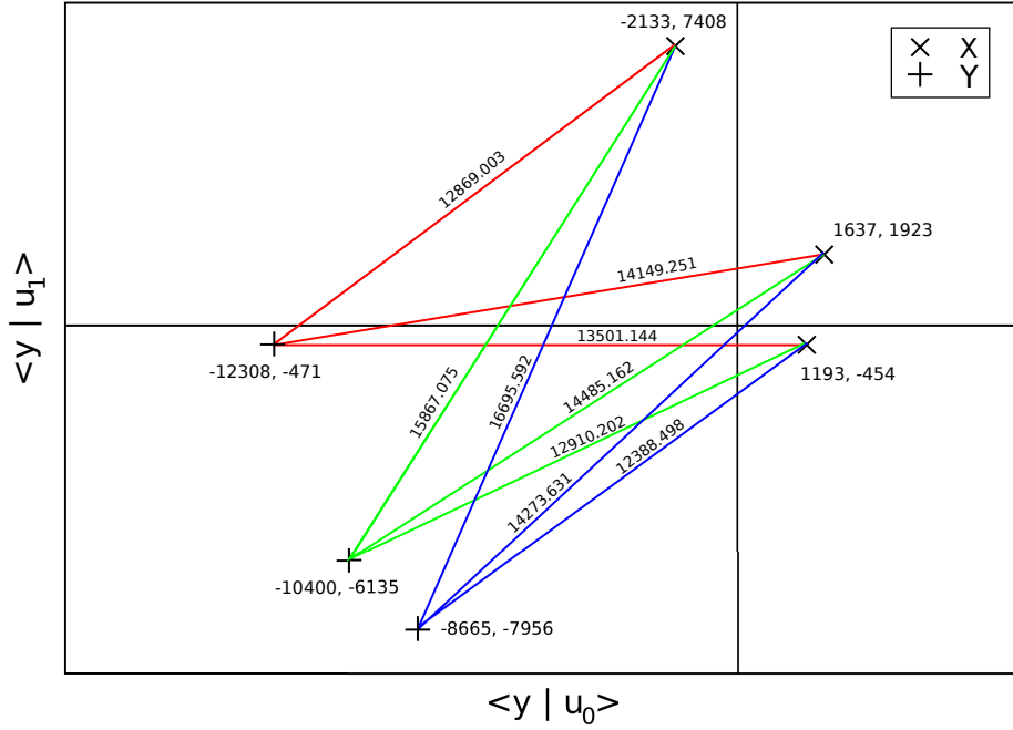
FIGURE 2.12 – Projections de signaux tatoués sur N_c = 2 porteuses secrètes : construction d'un graphe biparti pondéré pour la méthode CW avec 2 partitions de N_m = 3 sommets, corrélations hôtes et corrélations marquées. Les distances euclidiennes (poids) sont notées sur chaque arête.
