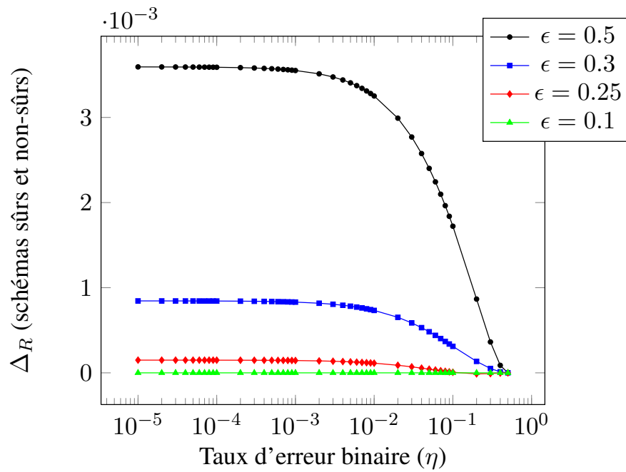
FIGURE 4.10 – \Delta_R = R'_s(\theta_{\epsilon WCA}, \epsilon, \eta) - R'_s(\theta_{WCA}, 0., \eta) en fonction du taux d’erreur binaire \eta pour \epsilon = 0.5, 0.3, 0.25, 0.1, c = 4 .
