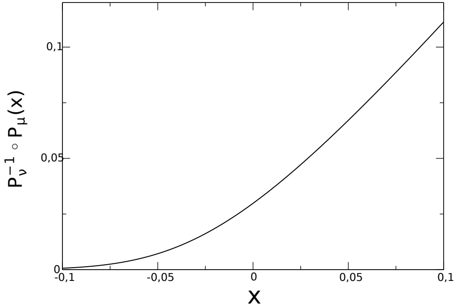
FIGURE 2.22 – Courbe y = P_\nu^{-1} \circ P_\mu(x) avec \eta = 1 , N_\nu = 512 et \sigma_x^2 = 1 .
