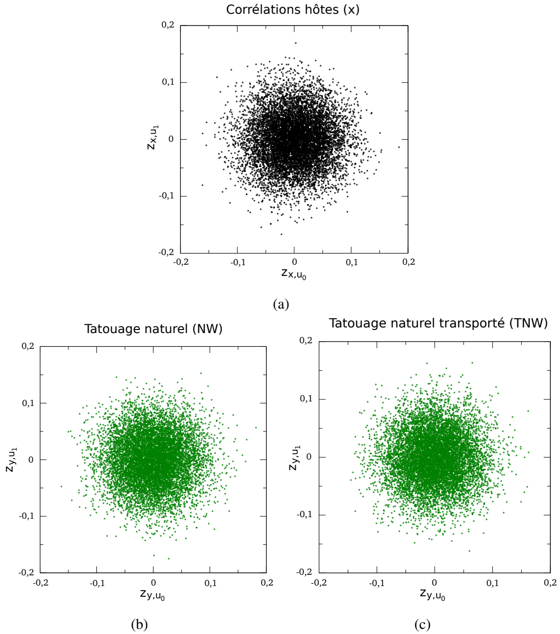
FIGURE 2.24 – Distribution des corrélations entre les signaux hôtes (a), NW (b) et TNW (c) et deux porteuses secrètes avec les paramètres N_o = 2000 , N_v = 512 , N_c = 10 . Comme prévu, les distributions pour NW et TNW sont identiques à la distribution hôte. L'affectation donnée par la théorie du transport ne modifie pas la sécurité su schéma classique NW.
