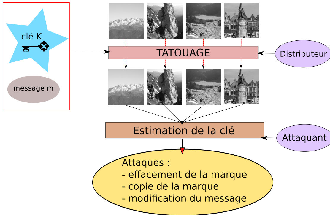
FIGURE 1.6 – Attaque par fuite d’information : un adversaire a accès à plusieurs contenus tatoués avec la même clé secrète. Selon le nombre de contenus en sa possession et la sécurité du schéma de tatouage, ce dernier aura une estimation de la clé secrète partielle ou totale et pourra alors altérer les messages cachés (effacement ou modification des messages) ou copier les messages sur d’autres contenus vierges.
