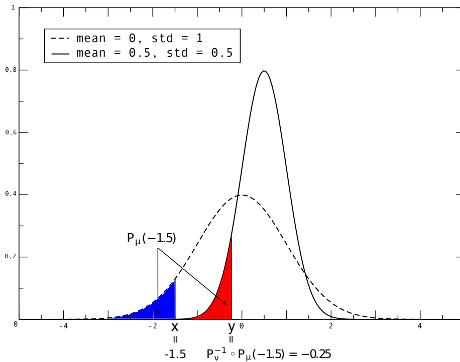
FIGURE 2.20 – Problème du transport : on cherche une bijection T qui minimise le coût total c de déplacement du sable \mathcal{X} de distribution \mu vers les creux \mathcal{Y} de distribution \nu .
