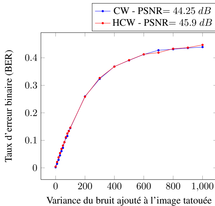
FIGURE 3.17 – Taux d'erreur binaire moyen en fonction de la variance du bruit n ajouté dans le domaine pixelique pour la modulation CW ainsi que son amélioration HCW basée sur une N_m -carte construite avec la même distorsion cible (distributions des corrélations entre signaux tatoués et porteuses secrètes identiques pour les deux méthodes). Nous remarquons que la méthode basée sur modèle ne modifie pas la robustesse du schéma initial.
