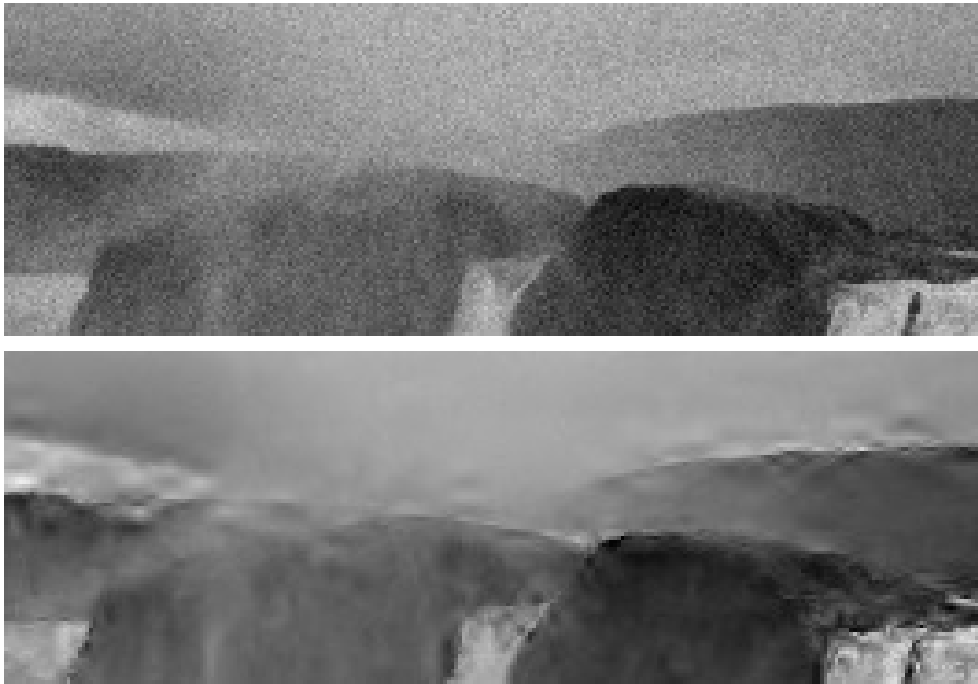
FIGURE 3.3 – Comparaison entre insertion constante (haut) et multiplicative (bas) (agrandissement des images de la figure 3.2). Le PSNR cible vaut 30 \text{ dB} . Modulation : CW ( \text{NCR} = -10 \text{ dB} ).
