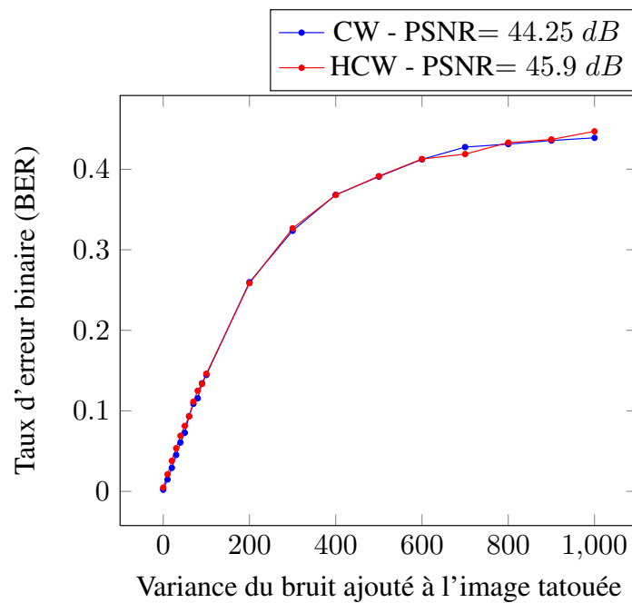
FIGURE 3.17 – Taux d'erreur binaire moyen en fonction de la variance du bruit \mathbf{n} ajouté dans le domaine pixelique pour la modulation CW ainsi que son amélioration HCW basée sur une N_m -carte construite avec la même distorsion cible (distributions des corrélations entre signaux tatoués et porteuses secrètes identiques pour les deux méthodes). Nous remarquons que la méthode basée sur modèle ne modifie pas la robustesse du schéma initial.
