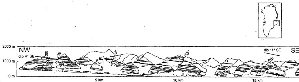
Figure 2.29. Coupe structurale de la zone de flexure de la côte Est-Groenlandaise [Pedersen et al. , 1997]. Noter l'augmentation du pendage des coulées vers l'Est et les failles normales à regard Ouest. Ces basaltes sont interprétés comme étant l'équivalent des SDRS qui sont observés sur les profils sismiques en mer.
