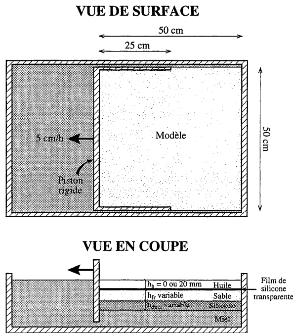
Figure 4.12. Dispositif expérimental. La lithosphère modèle, constituée d'une couche de sable et d'une couche de silicone, est placée dans une boîte remplie de miel. La surcharge glaciaire est modélisée par une couche d'huile disposée sur le modèle. L'huile est séparée du sable par un film de silicone transparent. L'ensemble est soumis à une extension par un piston rigide en U qui se déplace à une vitesse de 5 cm/h.
