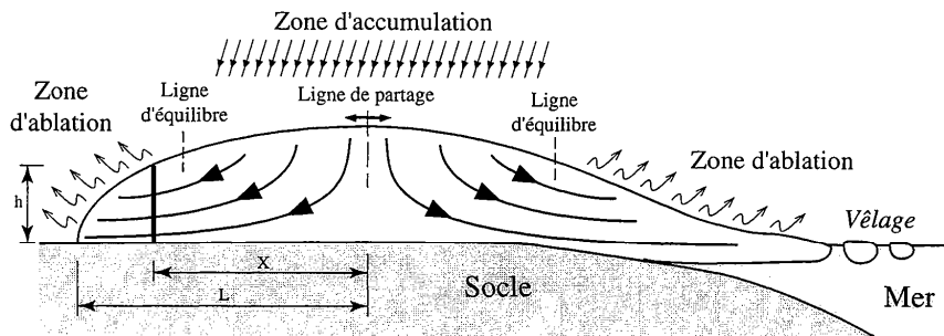
Figure 3.2. Coupe schématique d'une calotte glaciaire montrant les lignes d'écoulement. Le bilan glaciaire est positif dans la zone d'accumulation, négatif dans la zone d'ablation. La glace s'écoule sous l'effet du déséquilibre de masse entre la zone d'accumulation et la zone d'ablation. La vitesse d'écoulement est nulle sous la ligne de partage et au front de la calotte ; elle est maximale au niveau de la ligne d'équilibre.
