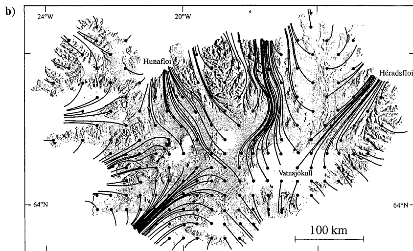
Figure 3.17. Reconstructions de l'écoulement de la calotte glaciaire prenant en compte la distribution des précipitations. Deux cas limites sont envisagés. a) Précipitations uniformes sur l'ensemble de la calotte glaciaire ; ablation uniquement à la périphérie. Les lignes d'écoulement sont tracées à partir des noeuds d'une grille régulière. b) Précipitations deux fois plus abondantes dans la moitié Sud de l'île que dans la moitié Nord ; ablation uniquement à la périphérie. La densité de la grille est deux fois plus petite au Nord qu'au Sud.
