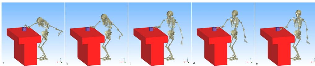
Figure 5.5 – Étapes d'une procédure d'optimisation de posture. Toutes les configurations sont sans collision, respectent les contraintes d'équilibre et la tâche sur la position de la main. De gauche à droite, les configurations sont de plus en plus naturelles.
