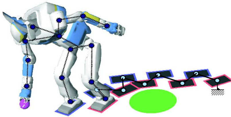
Figure 3.7 – Calcul automatique des empreintes de pas nécessaires à la réalisation d’une tâche d’atteinte. Le calcul se fait en intégrant la position des pas comme une chaîne articulatoire virtuelle dans le calcul de cinématique inverse. Figure tirée de (Kanoun et al. , 2010).
