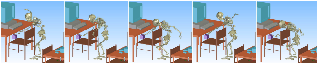
Figure 5.2 – Échantillonnage de sous-variété de \mathcal{CS} . Les contraintes à vérifier sont : les positions des pieds, la position du centre de masse et la position de la main droite. \mathcal{CS} est échantillonné uniformément, chaque échantillon est ensuite projeté sur la sous-variété qui vérifie les contraintes grâce aux outils de cinématique inverse, puis passé au détecteur de collisions.
