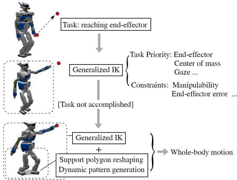
Figure 3.6 – Cinématique inverse hiérarchisée généralisée à la marche. La réalisation de la tâche d’atteinte nécessite que le robot fasse un pas. La position de ce pas est décidée de façon heuristique. Ensuite un même algorithme de résolution de tâches de cinématique inverse génère le mouvement d’atteinte et garantit l’équilibre dynamique. Figure tirée de (Yoshida et al. , 2006).
