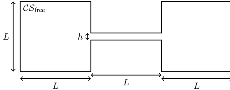
Figure 2.5 – Espace des configurations à deux dimensions. L'espace libre comprend un passage étroit ( h \ll L ). Planifier un chemin qui passe par le passage étroit est difficile car il faut générer des échantillons à l'intérieur du passage, qui est de faible volume comparé à \mathcal{CS} .
