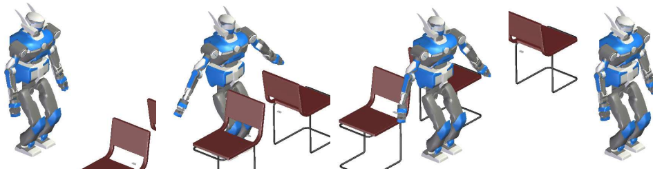
Figure 6.3 – Chemin sans collision pour un robot humanoïde glissant sur le sol. Les contraintes appliquées le long du chemin concernent : (i) les positions relatives des pieds, (ii) la position du centre de masse, (iii) la verticalité du bassin.
