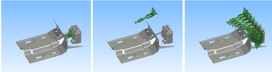
Figure 4.9 – Problème de désassemblage d'un pot d'échappement. Configurations initiale et finale et chemin solution.
