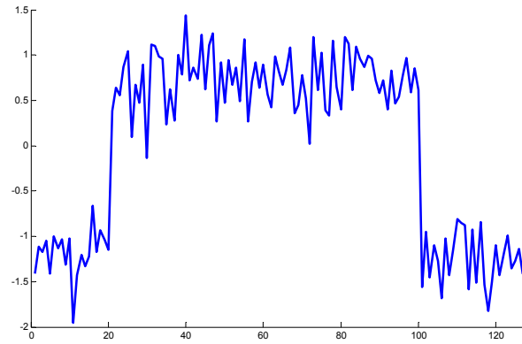
Fig. 3.2 (a). Noise
