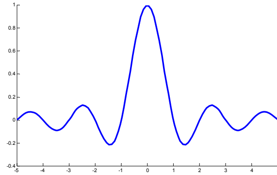
Fig. 3.2 (e). Outlier
