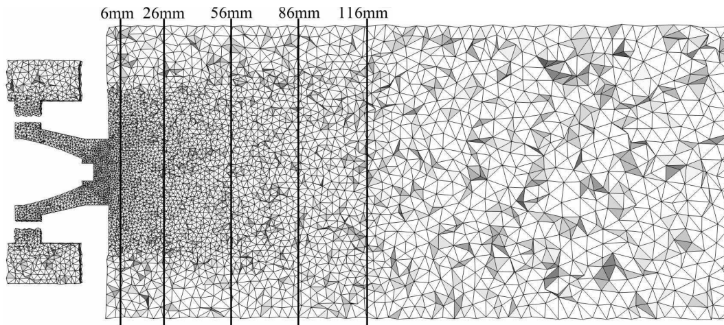
FIGURE 6.5 – Coupe longitudinale du maillage avec les positions des plans de mesure.
