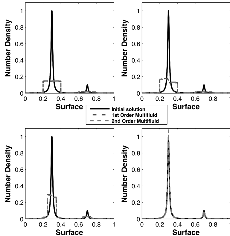
FIGURE 5.15 – Reconstruction initiale de la condition bimodale pour 5 (en haut à gauche), 10 (en haut à droite), 20 (en bas à gauche) et 100 (en bas à droite) sections : solution initiale (ligne continue), modèle d'ordre 1 (ligne point-tirée) et modèle d'ordre 2 (ligne tiretée).
