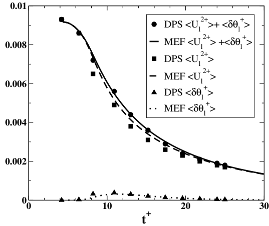
FIGURE 4.4 – Evolution de l'énergie moyenne de la phase dispersée : énergie totale obtenue par DPS (cercles) et par FEM (ligne continue) ; énergie corrélée obtenue par DPS (carrés) et FEM (ligne discontinue) ; énergie décorrélée obtenue par DPS (triangles) et FEM (ligne pointillée).
