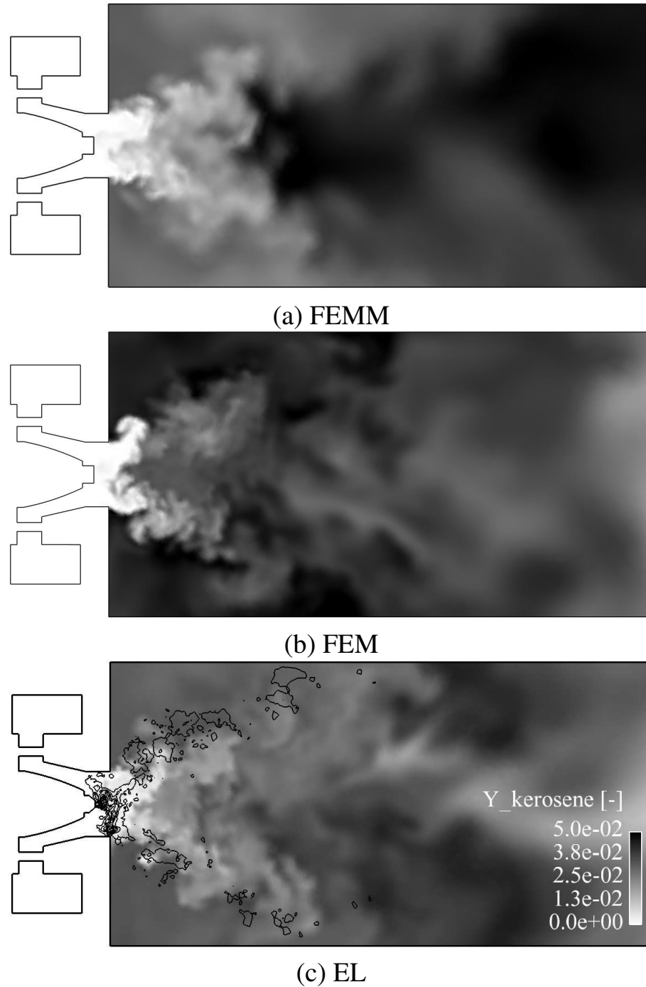
FIGURE 8.26 – Coupe longitudinale de fraction massique de kérosène instantanée : comparaison entre FEMM (a), FEM (b) et EL (c).
