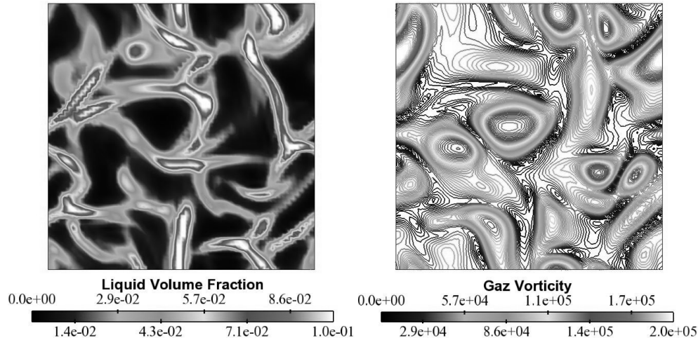
FIGURE 4.3 – Turbulence Homog ne Isotrope (plan de coupe m dian selon z ) : fraction volumique de liquide (gauche) et vorticit  du gaz (droite).
