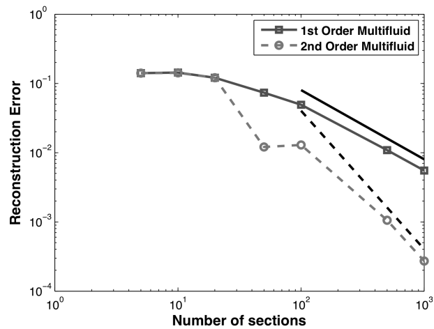
FIGURE 5.16 – Erreur de reconstruction en fonction du nombre de sections pour la condition initiale bi-modale avec le modèle d’ordre 1 (carrés) et le modèle d’ordre 2 (cercles).
