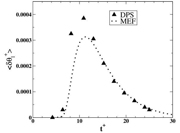
FIGURE 4.5 – Evolution de l'énergie décorrélée : DPS (triangles) et FEM (ligne pointillée).
