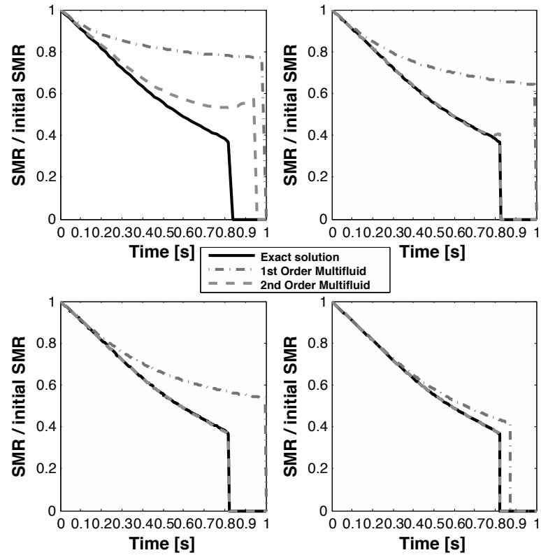
FIGURE 5.9 – Evolution du SMR rapporté au SMR initial pour la solution initiale gaussienne avec 5 (en haut à gauche), 10 (en haut à droite), 20 (en bas à gauche) et 100 (en bas à droite) sections : solution exacte (ligne continue), modèle d’ordre 1 (ligne point-tirée) et modèle d’ordre 2 (ligne tiretée).
