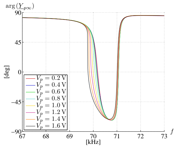
(d) Phase de \underline{Y}_{p\infty} à P = 500 mbar
