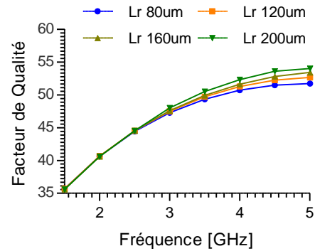
Figure IV - 12 : Facteurs de qualités en fonction de la fréquence et L_r
