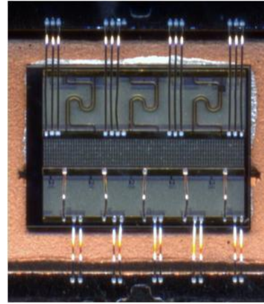
Figure IV - 36 : Puce montée dans son boîtier et câblée
