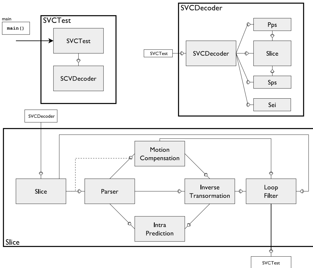
FIGURE 8.4 – Architecture de l’application de décodage SVC implémentée avec des composants Cecilia.
