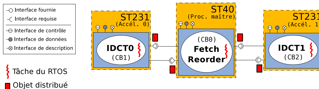
FIGURE 6.3 – Déploiement de l'application de MJPEG sur la plate-forme STi7200
