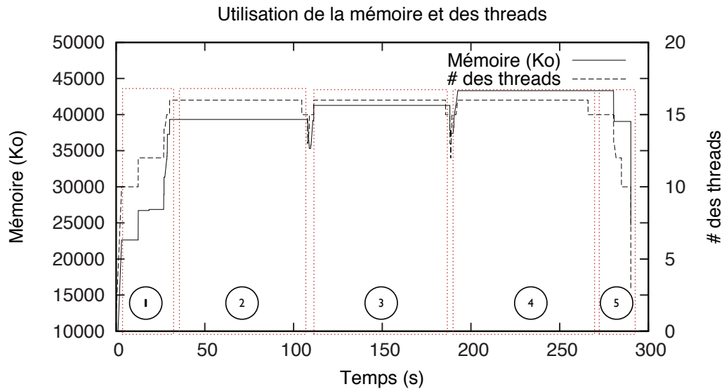
FIGURE 7.9 – Évolution de l’utilisation de la mémoire et des threads utilisées par l’application sur trois exécutions
