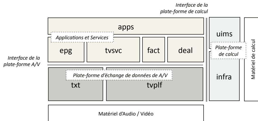
FIGURE 3.3 – Niveaux d’abstraction gérés par Koala
