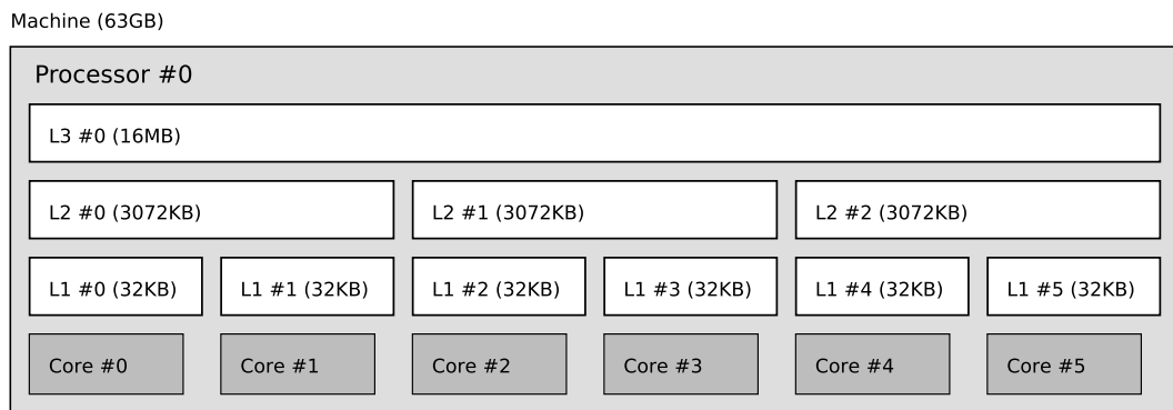
FIGURE 8.1 – Organisation des cœurs et de la mémoire cache dans le processeur Intel x7460
