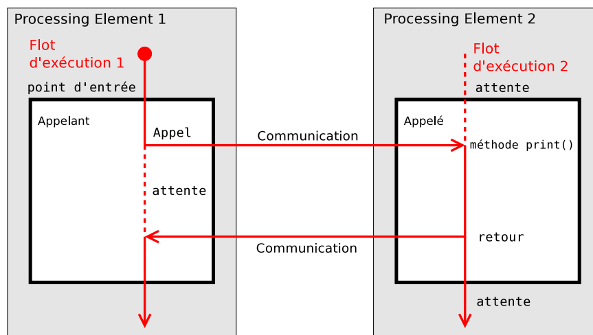
FIGURE 8.5 – Modèle d'exécution de Comete
