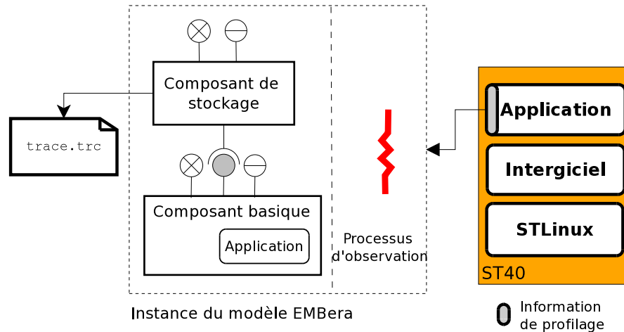
FIGURE 7.3 – Composants EMBerA utilisés pour observer l'application de décodage
