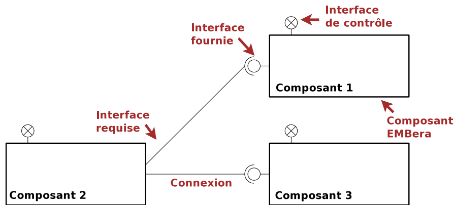
FIGURE 5.1 – Le modèle à composants EMBera
