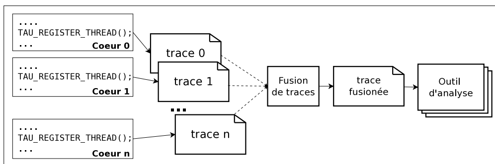
FIGURE 2.5 – Gestion des traces dans TAU
