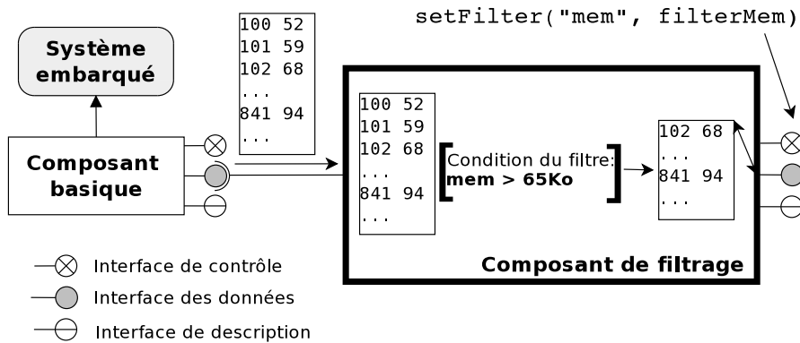
FIGURE 5.4 – Exemple de composant de filtrage
