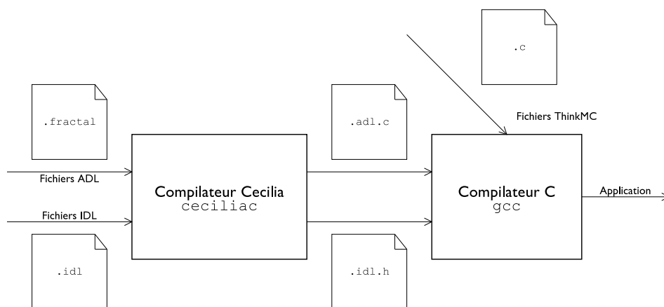
FIGURE 8.2 – Chaîne d'outils Cecilia
