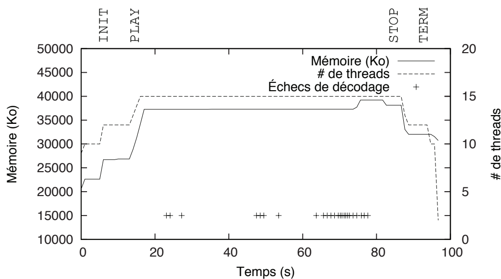
FIGURE 7.10 – Corrélation des événements applicatifs avec l'intergiciel et le système
