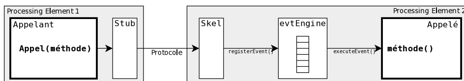
FIGURE 3.2 – Schéma de communication dans Comete
