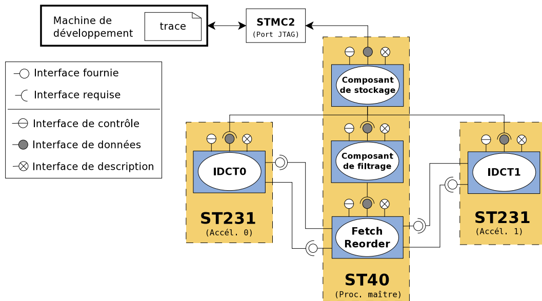
FIGURE 6.8 – Déploiement des composants d’observation EMBerA
