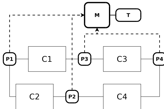
FIGURE 3.4 – Observation d’une application CCA avec PMM
