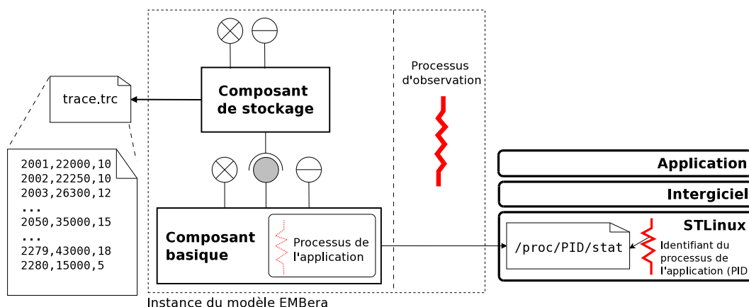
FIGURE 7.5 – Composants EMBera utilisés pour observer le processus de l'application
