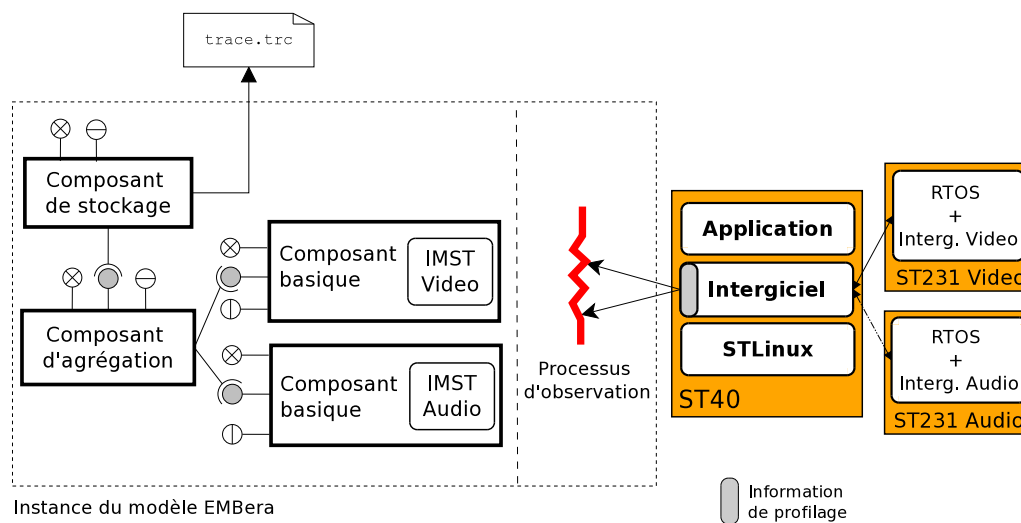
FIGURE 7.4 – Composants EMBera utilisés pour observer l'intergiciel multimédia
