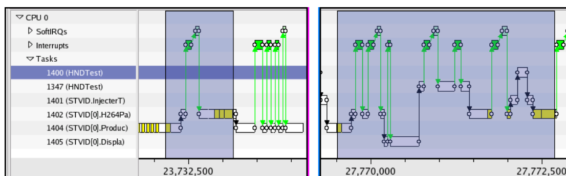
FIGURE 7.8 – Différences des temps d'exécution des fonctions de décodage
