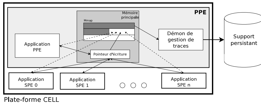
FIGURE 2.4 – Collecte de traces du processeur CELL
