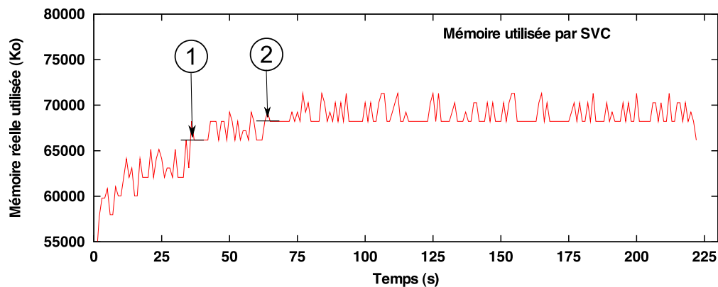
FIGURE 8.14 – Évolution de l'utilisation mémoire de l'application SVC
