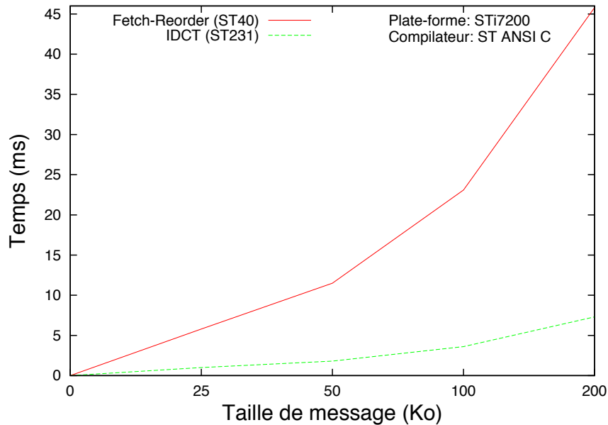
FIGURE 6.10 – Temps de communication en utilisant la primitive send
