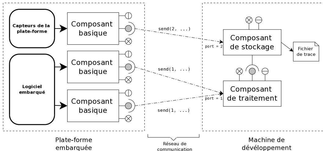
FIGURE 7.2 – Exemple de déploiement des composants EMBerA
