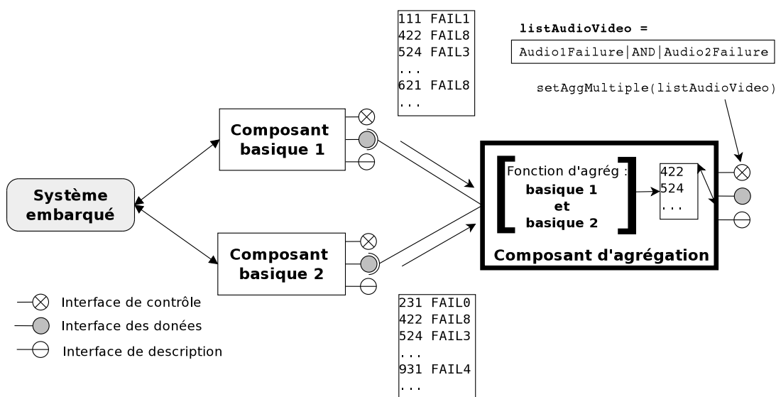
FIGURE 5.5 – Exemple de composant d'agrégation
