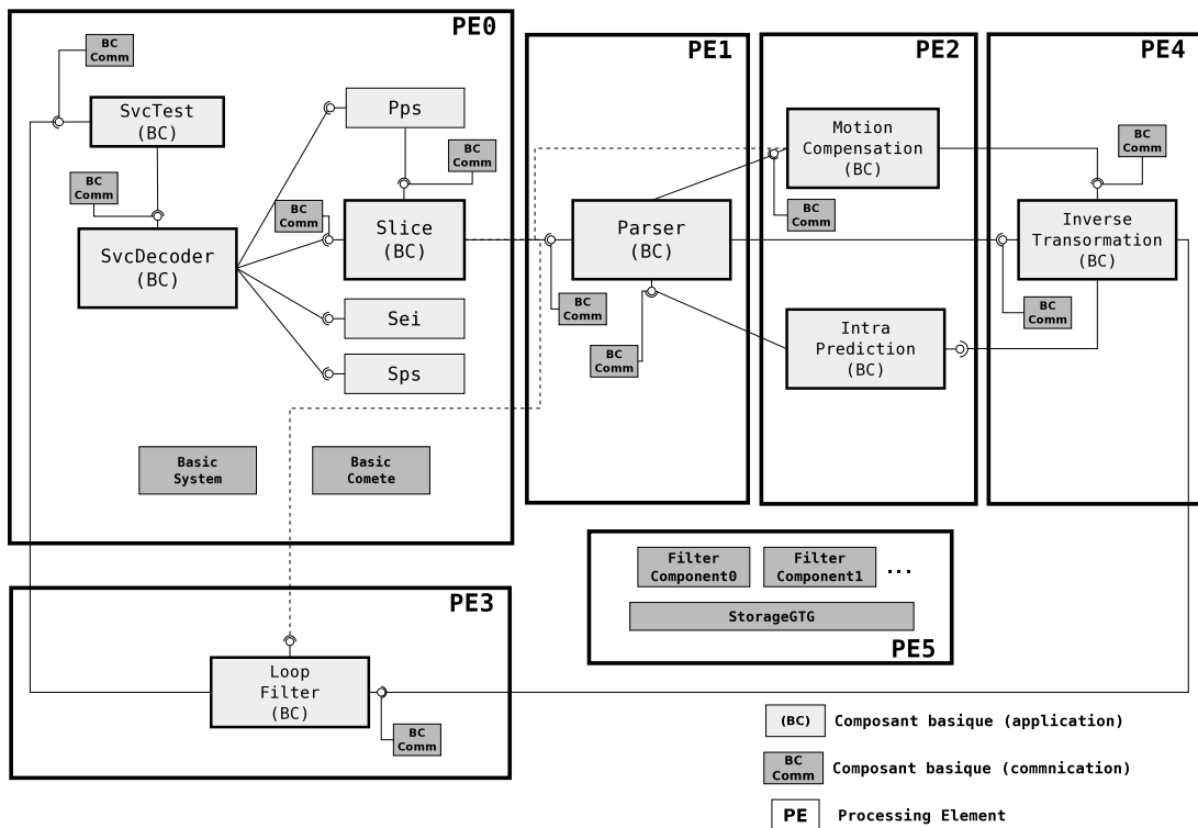
FIGURE 8.12 – Déploiement des composants SVC et EMBera
