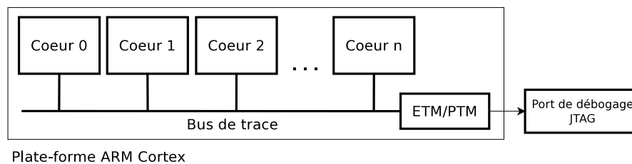
FIGURE 2.3 – Plate-forme multi-cœur ARM avec des composants de traçage ETM/PTM
