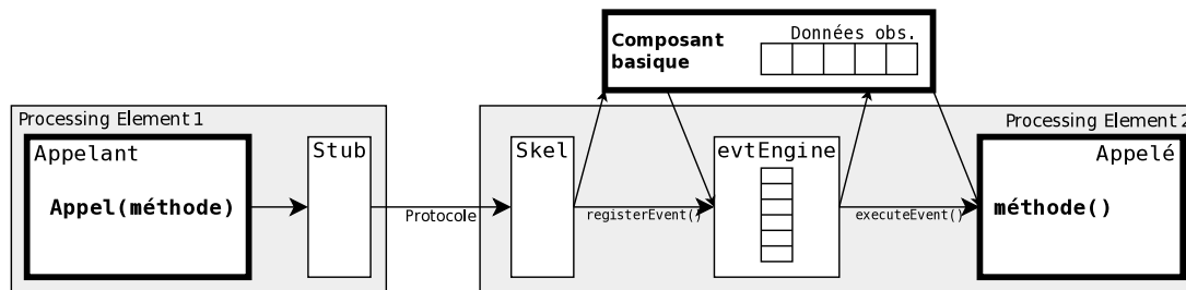
FIGURE 8.7 – Composant basique observant la communication dans Comete
