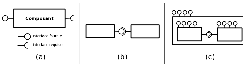
FIGURE 3.1 – Interfaces, connexions et composition des composants
