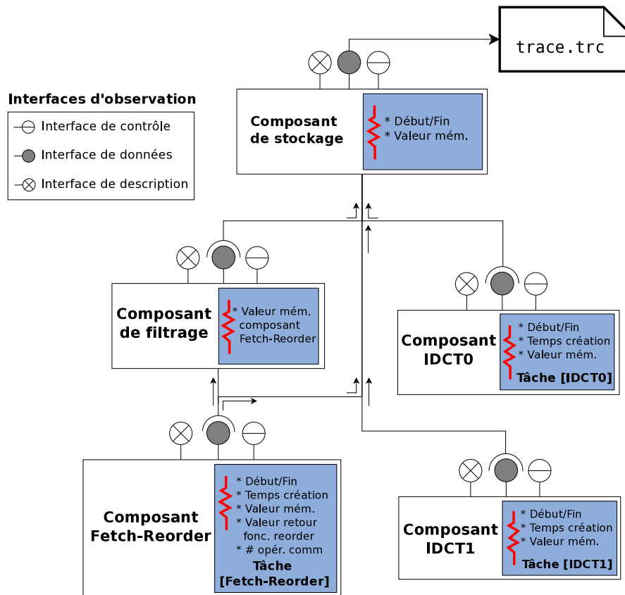
FIGURE 6.6 – Composants EMBERA utilisés pour l'observation de l'application MJPEG
