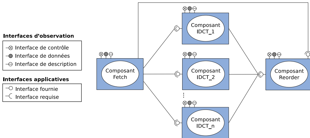
FIGURE 6.2 – Application de décodage MJPEG avec des composants EMBera
