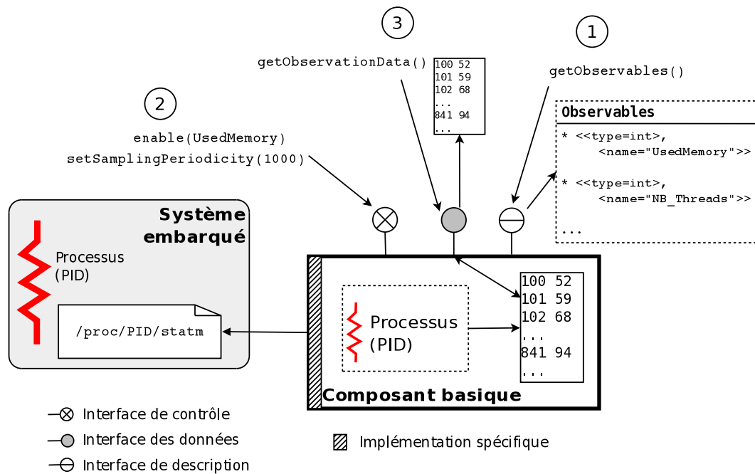
FIGURE 5.3 – Exemple de composant basique : observation de la mémoire utilisée par un processus
