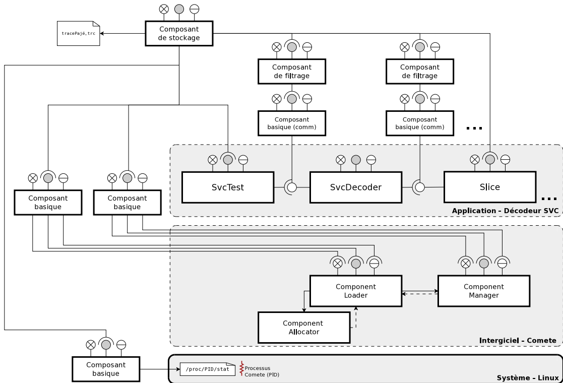
FIGURE 8.8 – Composants EMBera utilisés pour l'observation du décodeur SVC
