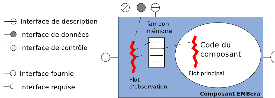
FIGURE 5.8 – Implémentation des composants d’observation EMBera
