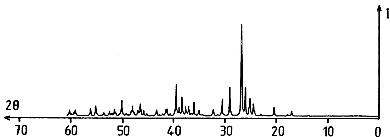
(b) \text{Cs}_4\text{Mg}_3\text{F}_{10}
