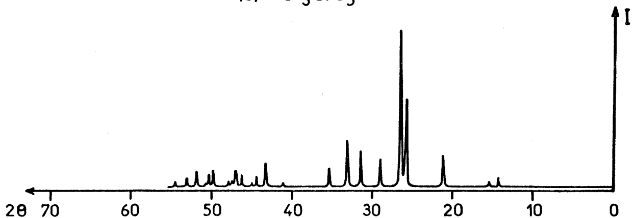
(b) \text{Rb}_3\text{MgH}_5
