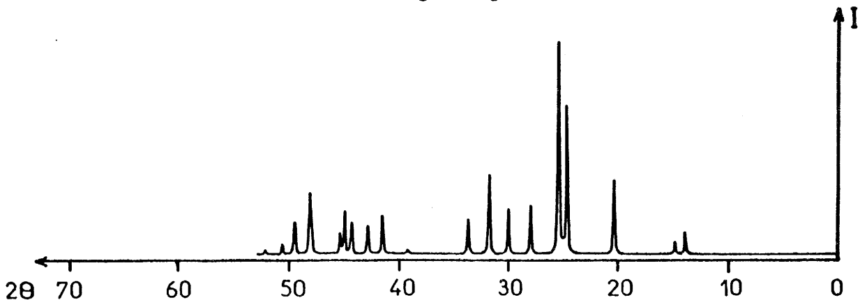
(a) \text{Cs}_3\text{MgH}_5
