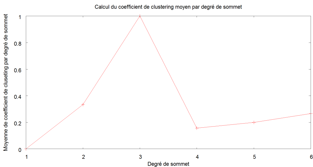
FIGURE 9.4: Coefficient de clustering moyen par degré de sommet de l'exemple présenté dans la figure 9.3.
