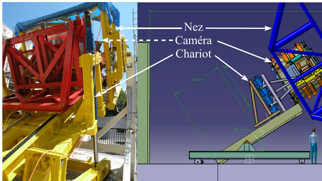
FIGURE 8.4 – Système de mise au point : deux systèmes symétriques sont situés de part et d'autre de la caméra (à gauche), composés d'un moteur assurant le déplacement sur un rail le long de l'axe optique (à droite), et de deux pinces hydrauliques pour le maintien de la caméra (Photographie et schéma du LAPP : janvier 2008).
