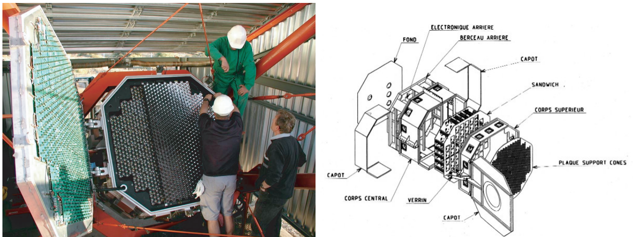
FIGURE 6.6 – Caméra de H.E.S.S. Image de gauche : Photographie de la face avant d'une des caméras de H.E.S.S. avec le capot de protection des PM ouvert.
