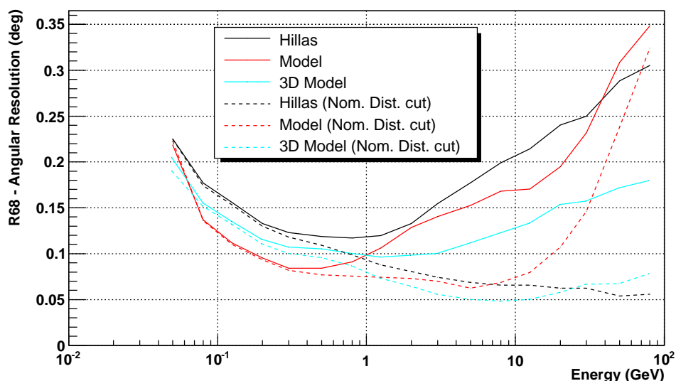
FIGURE 7.7 – Résolution des différentes méthodes de reconstruction pour une coupure définie. Les résultats obtenus avec et sans coupure sur la distance nominale (distance du centre de l'image de la gerbe au centre de la caméra) [64].
