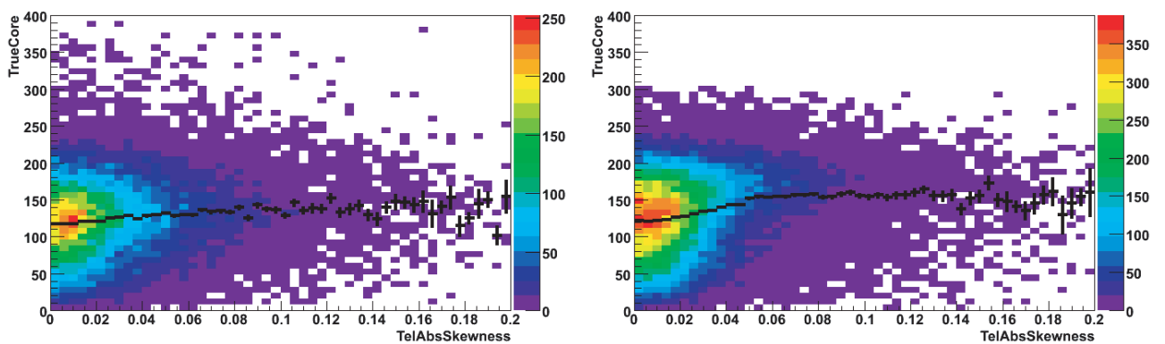
Corrélation du skewness avec le paramètre d'impact.
