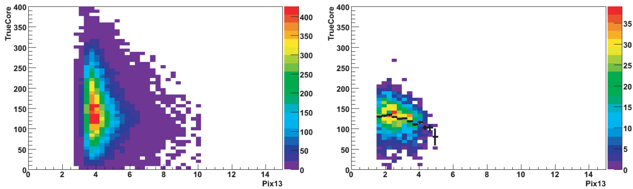
Corrélation de PixMax13 avec le paramètre d'impact.
