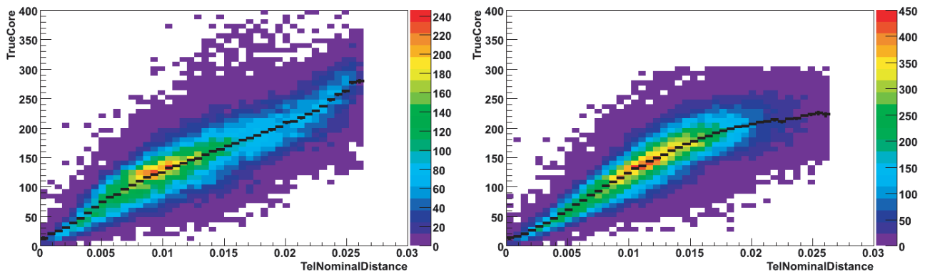
Corrélation de la distance nominale avec le paramètre d'impact.
