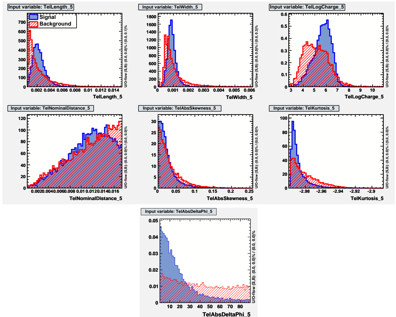
FIGURE 11.11 – Distribution des 7 variables utilisées en entrée des analyses multivariables pour la discrimination photons / hadrons. En bleu sont représentées les variables des gerbes électromagnétiques simulées de 50 et 80 GeV, en rouge les variables des gerbes hadroniques simulées de 30 GeV à 100 TeV.
