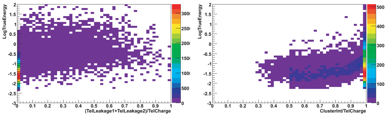
Corrélation de la fuite (leakage) et du fractionnement de l'image avec l'énergie.
