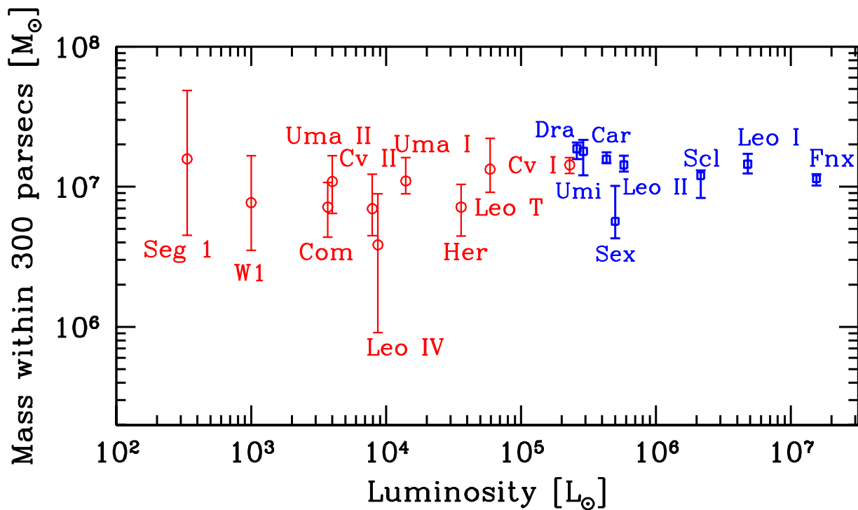
FIGURE 18.3 – Masses des galaxies naines du Groupe Local en fonction de leur luminosité dans le visible. [214].
