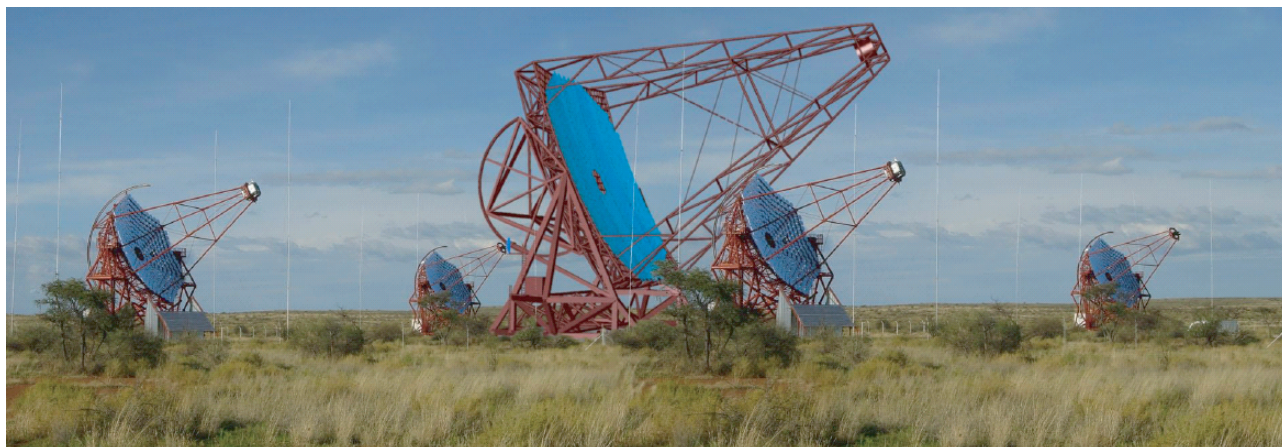
FIGURE 8.1 – Montage photographique représentant le télescope de la phase II au milieu des quatre télescopes actuels de la phase I.
