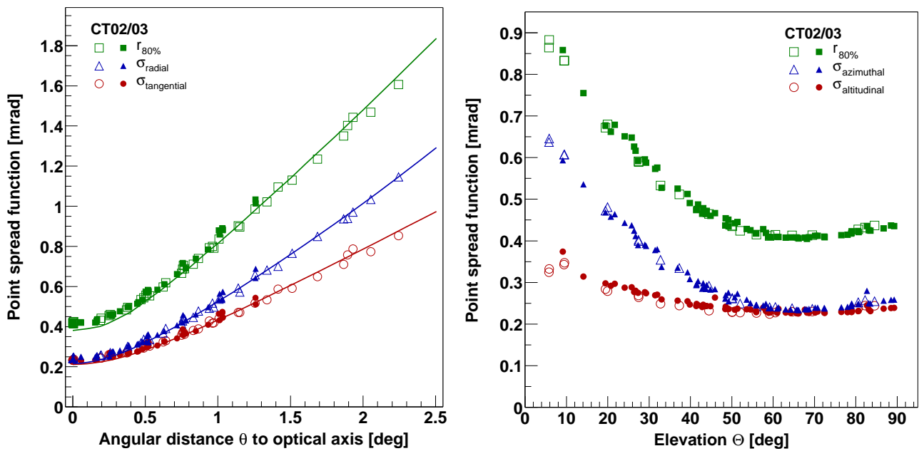
FIGURE 6.5 – Image de gauche : Evolution de la fonction d'étalement d'une source ponctuelle avec l'angle à l'axe optique. La variable r_{80\%} est le rayon incluant 80 % de l'image. \sigma_{radial} et \sigma_{tangential} sont les largeurs de l'image par rapport à l'axe optique. Image de droite : Evolution de la fonction d'étalement d'une source ponctuelle avec l'élévation. \sigma_{azimuthal} et \sigma_{altitude} sont les largeurs de l'image par rapport au pointé du télescope.
