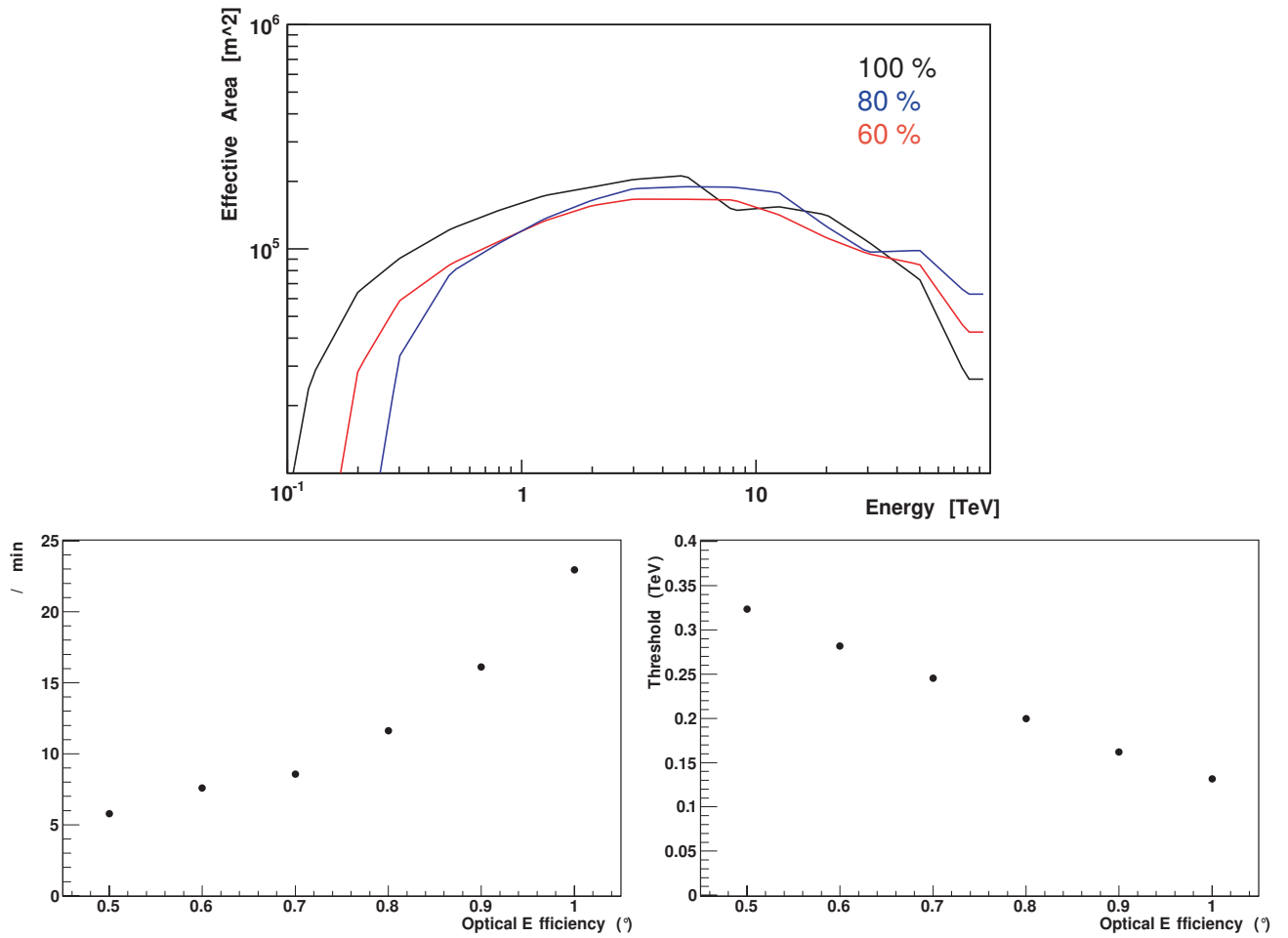
FIGURE B.3 – Evolution de l'acceptance, du seuil en énergie ainsi que du nombre de photons détectés par minute en fonction de l'efficacité optique.
