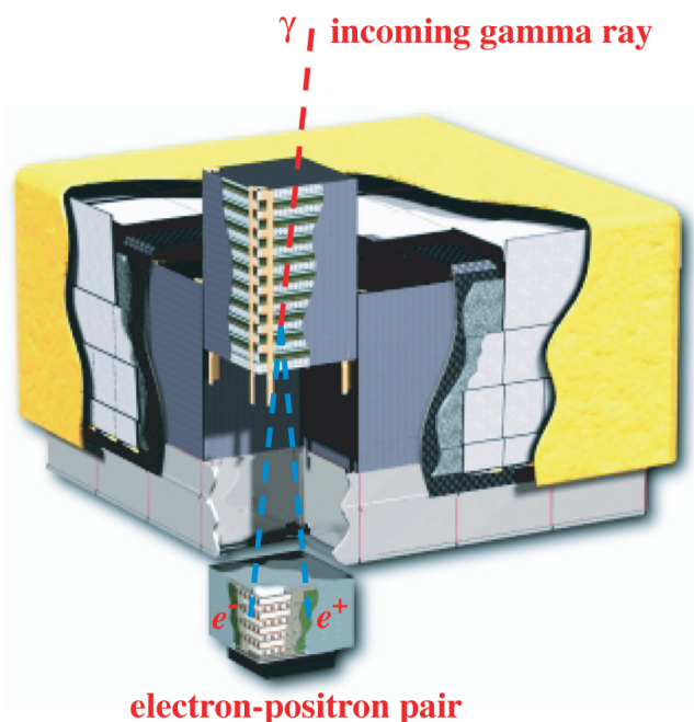
FIGURE 2.1 – Illustration de détecteur FERMI [23].
