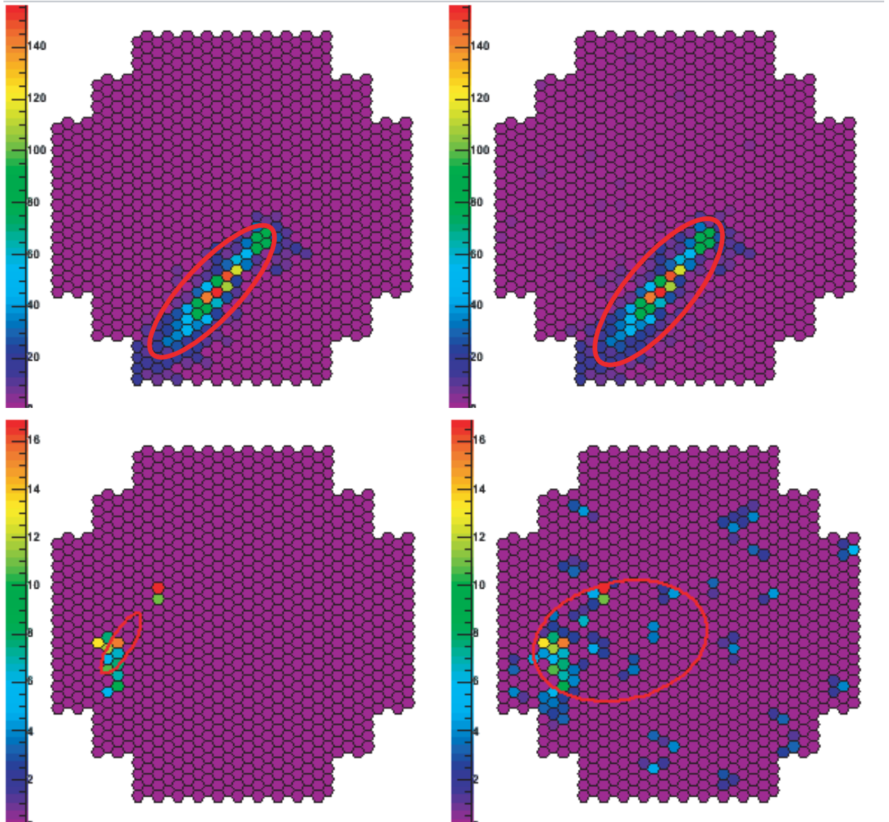
FIGURE 10.22 – Exemples d’images Cherenkov de gerbes atmosphériques simulées pour deux nettoyages différents. La colonne de gauche correspond à un nettoyage 5/10, la colonne de droite à 1/3. Les deux images du haut représentent une même gerbe électromagnétique, celles du bas une même gerbe hadronique, pour les deux différents nettoyages. Les gerbes elliptiques semblent être bien moins dépendantes du nettoyage que les gerbes hadroniques.
