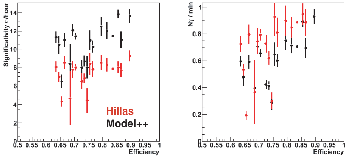
FIGURE 17.3 – Evolution de la significativité ( gauche ) et du taux de photons ( droite ) en fonction de l'efficacité optique pour les observations du centre galactique.
