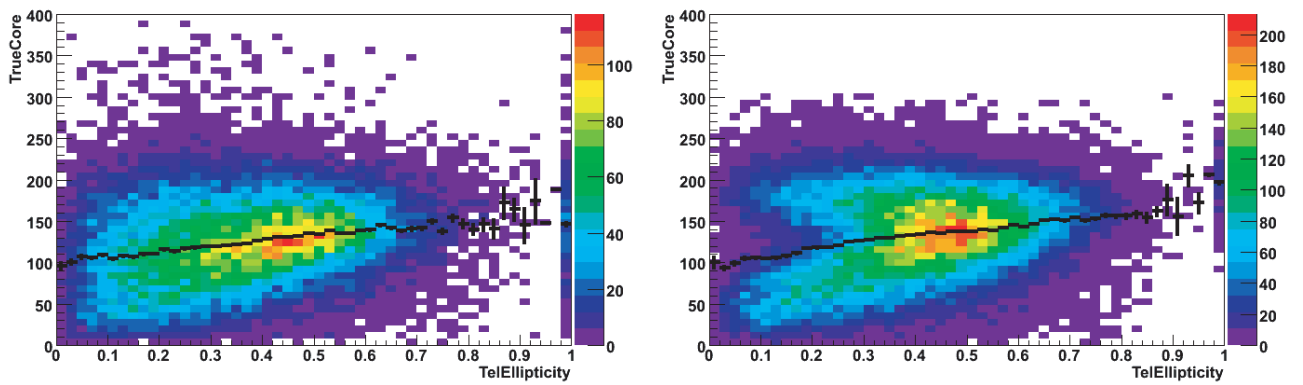
Corrélation de l'ellipticité avec le paramètre d'impact.
