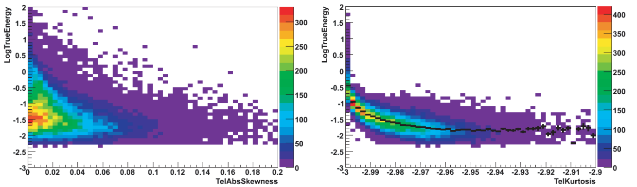
Corrélation du skewness et du kurtosis avec l'énergie.
