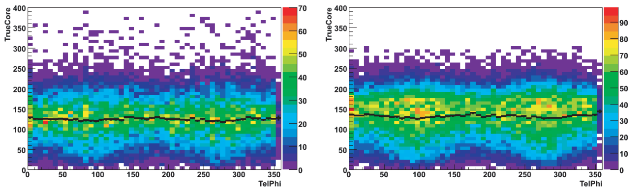
Corrélation de Phi avec le paramètre d'impact.
