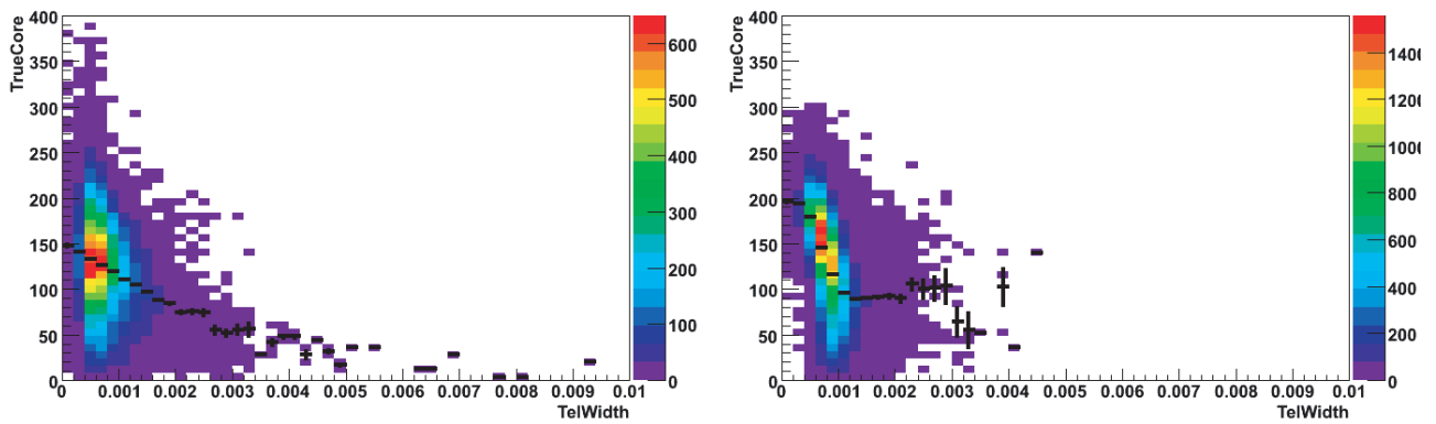
Corrélation de la largeur avec le paramètre d'impact.
