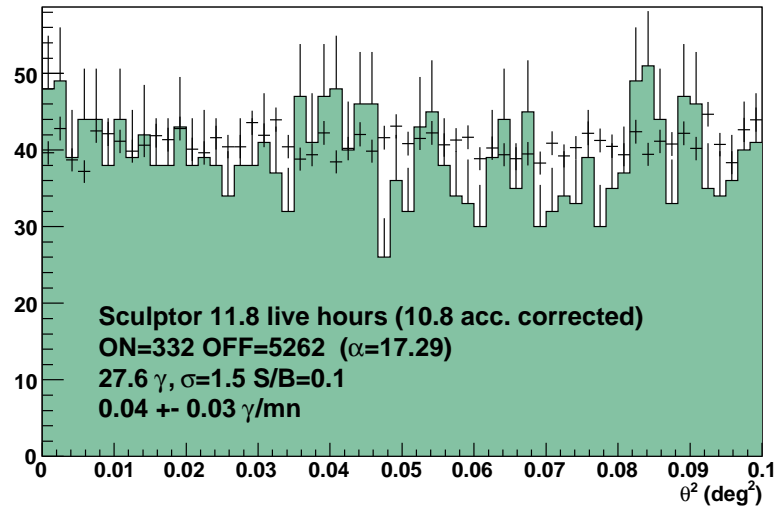
FIGURE 19.4 – Distribution radiale carré des événements par l'analyse Xeff de Sculptor .
