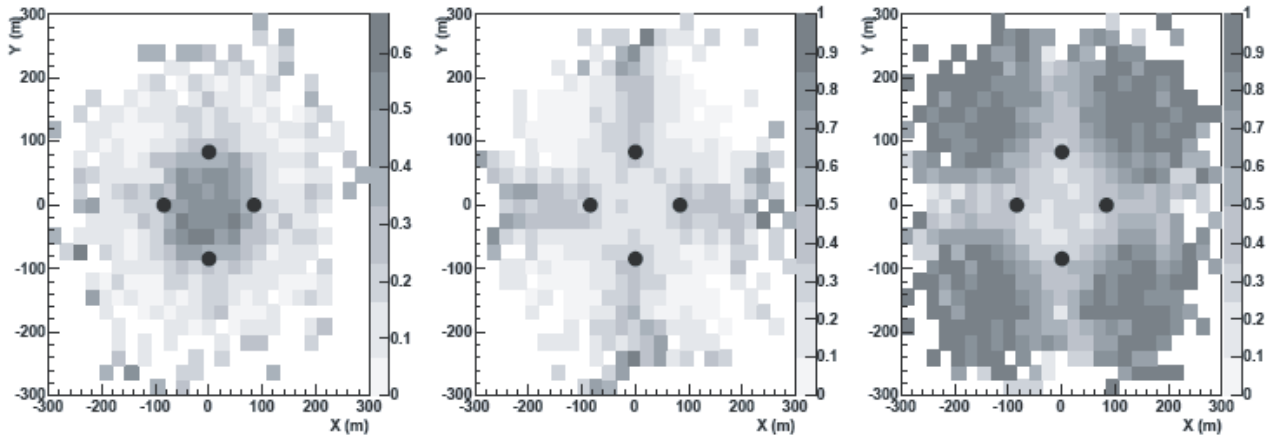
FIGURE 14.1 – Fraction des gerbes verticales de \gamma déclenchant n_T télescopes en fonction de la position du paramètre d'impact (de coordonnées X et Y) au sol. De gauche à droite : n_T = 4 , n_T = 3 , n_T = 2 . Cette figure a été obtenue en utilisant une simulation de loi de puissance d'indice 2.4. Les points noirs indiquent la position des télescopes de H.E.S.S.. Cette figure est issue de [148].
