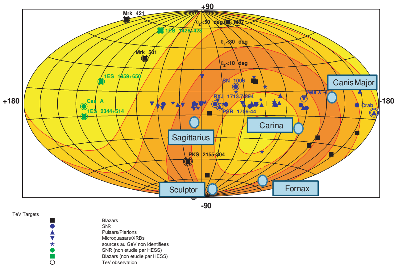
FIGURE 19.1 – Visibilité du ciel depuis le site de H.E.S.S., en coordonnées galactiques. Les contours en couleurs indiquent l'angle zénithal maximal dans chaque région du ciel sur toute l'année. L'angle zénithal maximal est indiqué dans chaque bande. La bande la plus foncée correspond à la région observable à moins de 10^\circ du zénith; les bandes les plus claires aux régions observables qu'à grand angle zénithal ( >50^\circ ).
