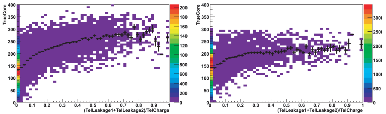
Corrélation de la fuite (leakage) avec le paramètre d'impact.
