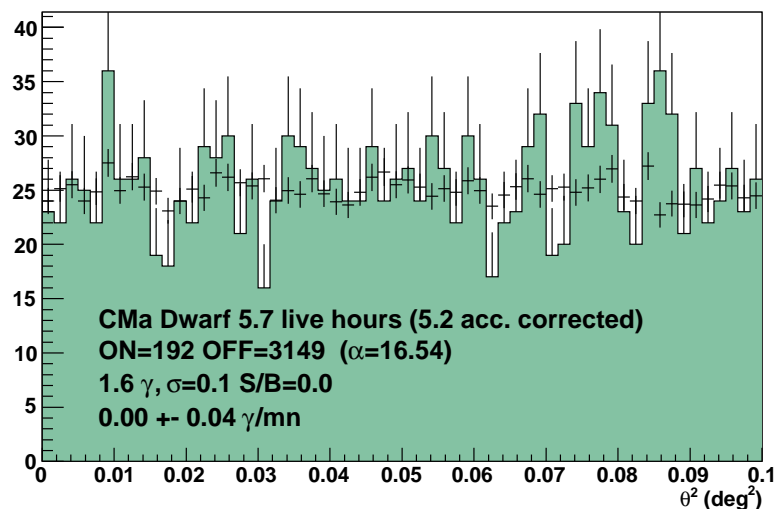
FIGURE 19.2 – Distribution radiale carré des événements par l'analyse Xeff de Canis Major .
