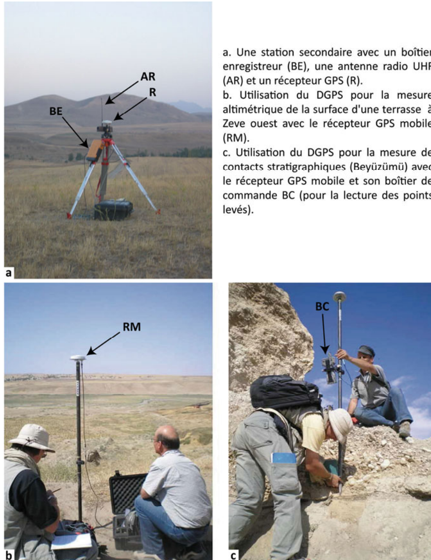
Figure 4-1. Présentation du DGPS
