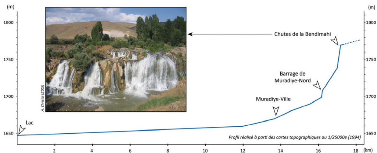
Figure 5-3. Le profil longitudinal de la Bendimahi
