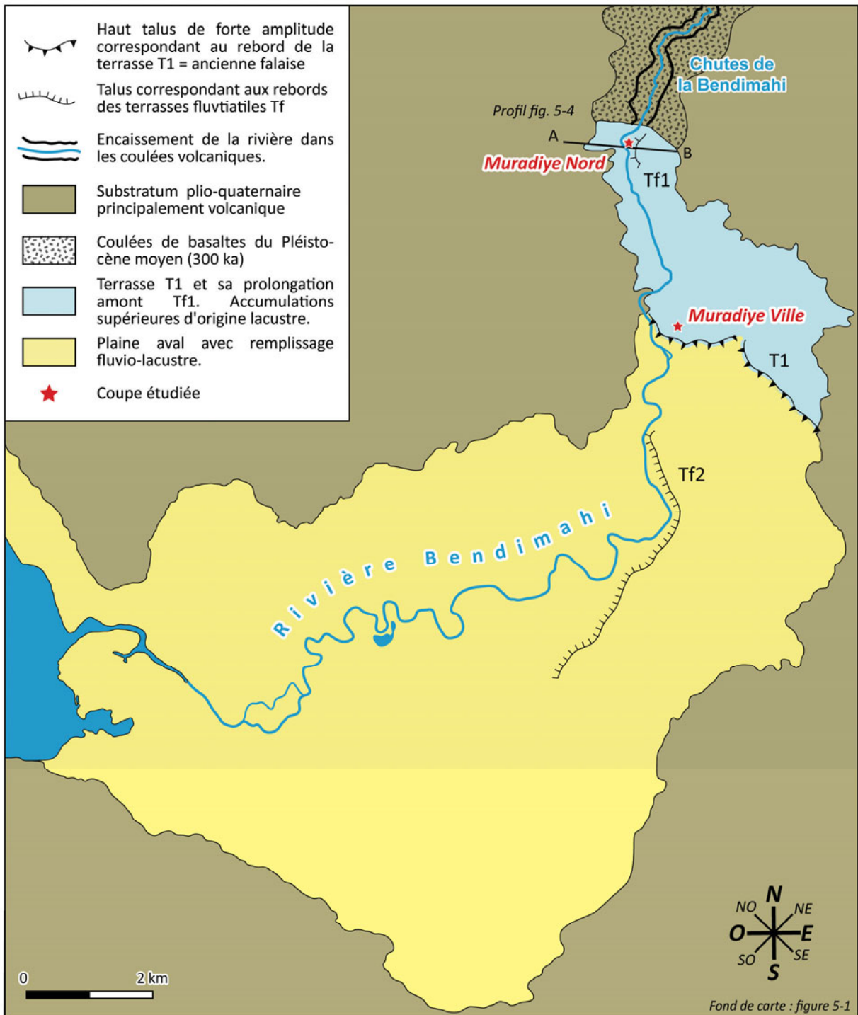
Figure 5-2. Schéma géomorphologique de la basse vallée de la Bendimahi
