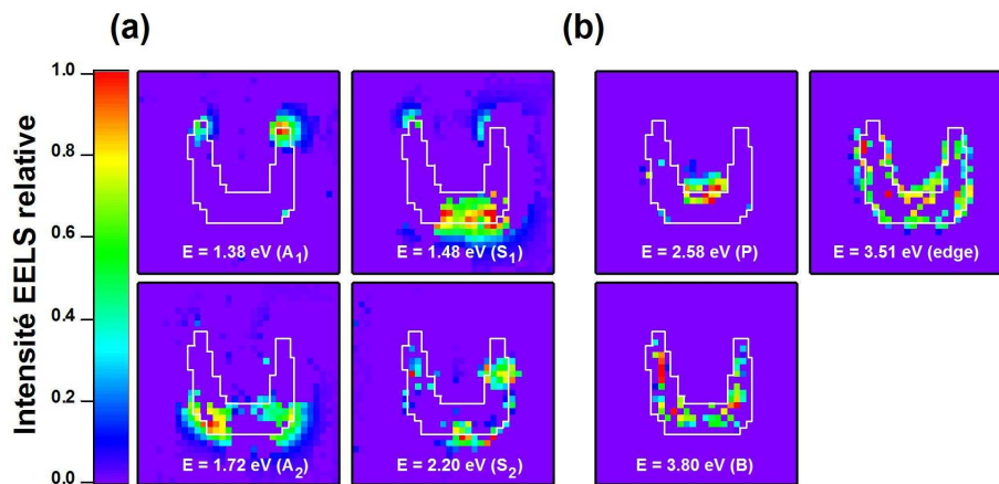
FIGURE 11.10 – Cartes d'intensité des résonances qui ont été résolues pour l'échantillon SRR3. (a) Résonances associées aux modes de surface qui sont interprétables en terme d'ondes stationnaires plasmoniques. (b) Résonances supplémentaires de plus haute énergie que nous avons détectées sur SRR3. Ces modes sont décrits dans la section 11.3. Le rapport entre les maxima comparé avec A_1 est (ordonné par ordre croissant d'énergie des plasmons) : 1/0.8/1.2/0.7/1.1/0.9/0.9 .
