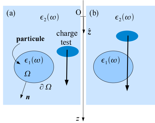
FIGURE 13.1 – On considère une particule de forme arbitraire en présence d'une charge test dont la trajectoire est soit non pénétrante (a) ou pénétrante (b). \hat{z} est un vecteur directeur porté par l'axe Oz et \mathbf{n} est un vecteur normal à la surface de la particule dirigé vers l'extérieur.
