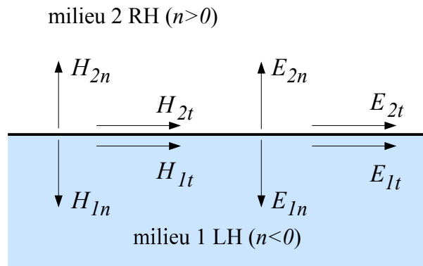
FIGURE 6.4 – Continuité des composantes tangentielles et discontinuité des composantes normales du champ magnétique et du champ électrique à l'interface entre un milieu RH ( n > 0 ) et un milieu LH ( n < 0 ).
