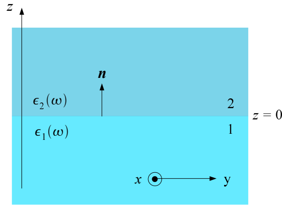
FIGURE C.1 – Interface plane séparant deux milieux semi-infinis caractérisés par les permittivités diélectriques locales \epsilon_1(\omega) ( z < 0 ) et \epsilon_2(\omega) ( z > 0 ). \mathbf{n} est un vecteur unitaire normal à l'interface et dirigé du milieu 1 vers le milieu 2.
