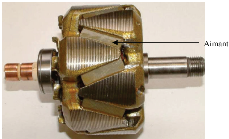
Fig 2.59-Rotor à griffes avec aimants interpolaires
