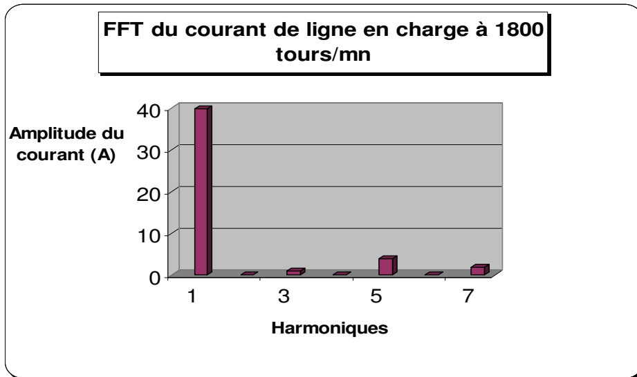
Fig 2.16 Transformée de Fourier du Courant dans une phase à 1800 tours/mn
