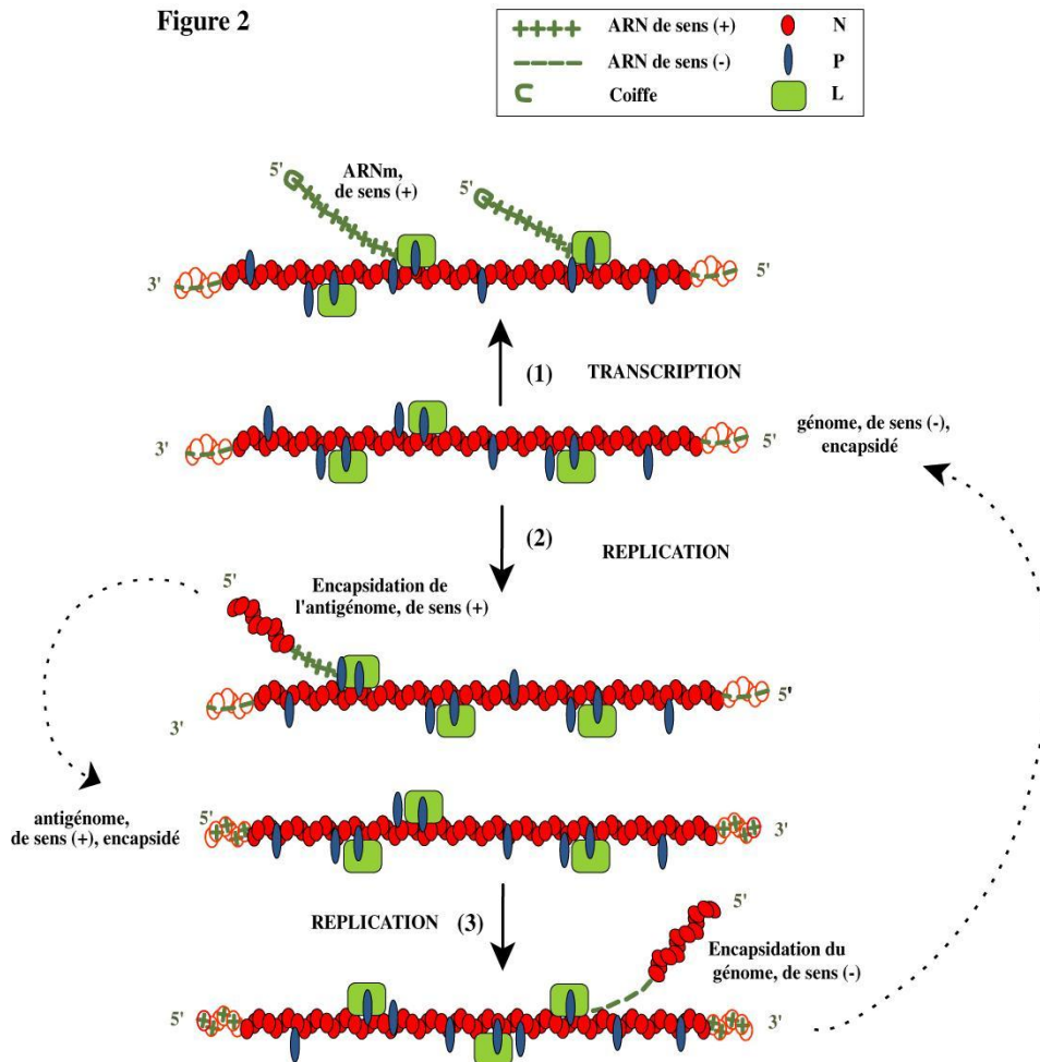
Figure 2. Cycle réplcatif.
