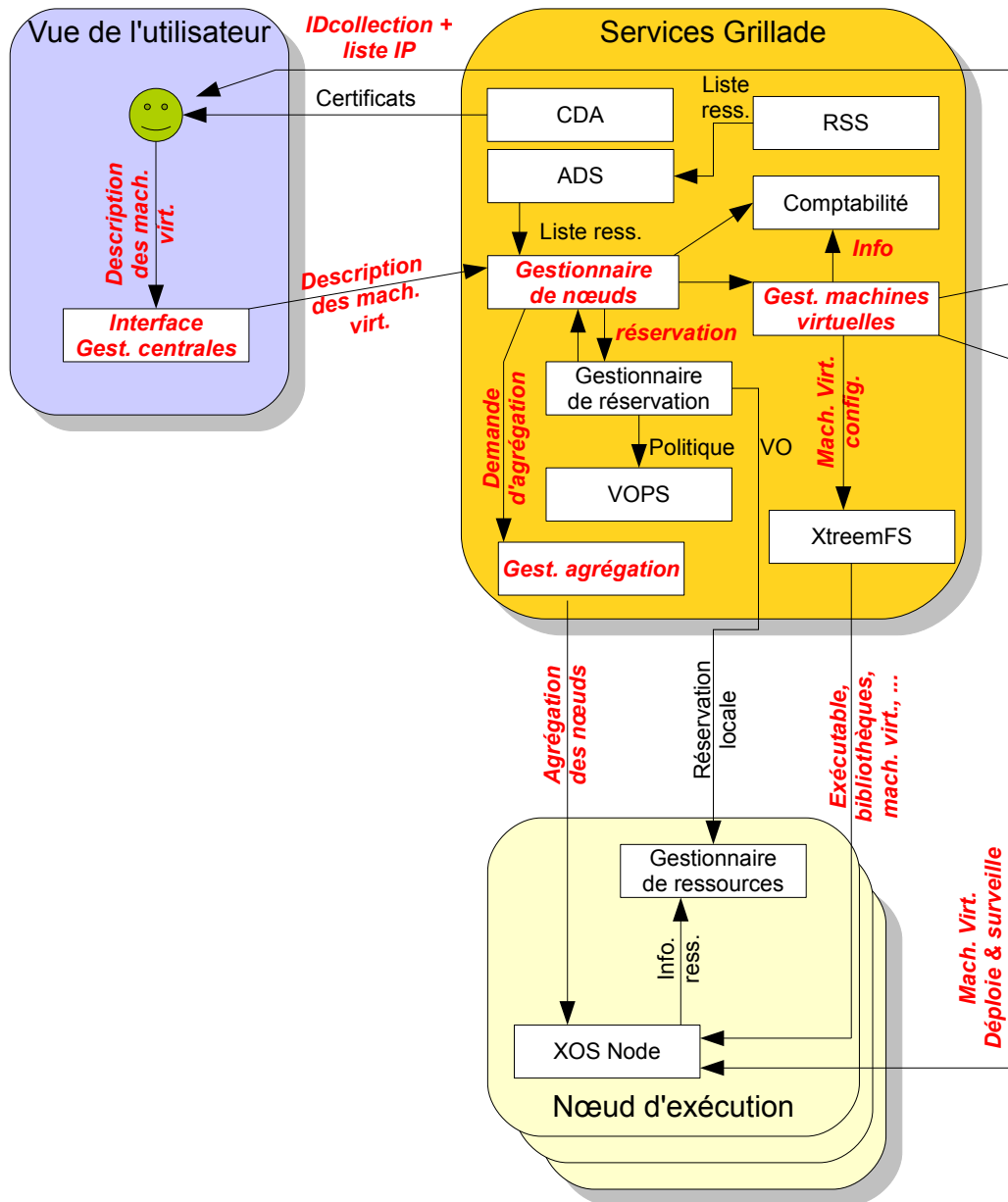
FIGURE 3.12 – Architecture de Grillade tenant compte des contraintes de mises en œuvre liées à XtreamOS pour le déploiement et la gestion des collections des machines virtuelles. Cette figure est un raffinement de la figure 3.11.
