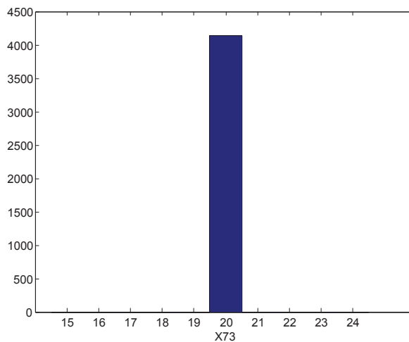
Figure 6.2 – Histogramme du test X_{73} (filtre).
