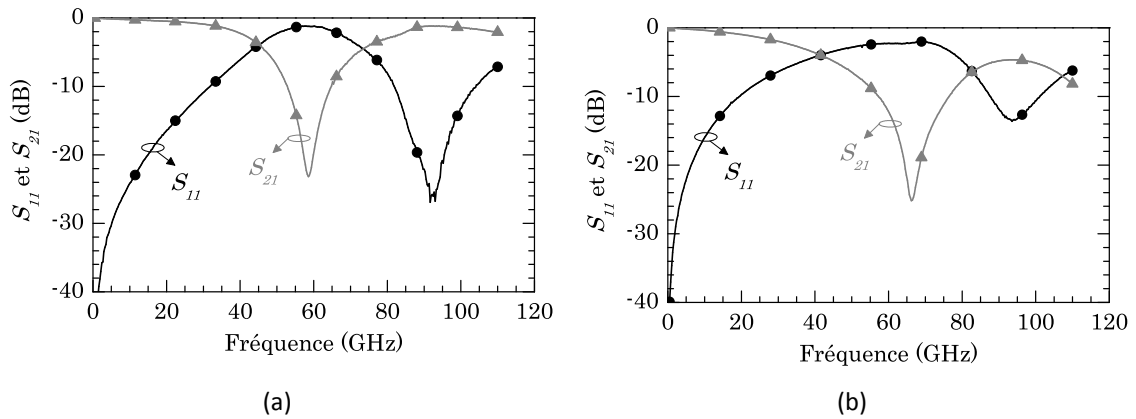
Figure 4.3 : Mesure de stubs S-CPW résonant à 60 GHz : a) Té-70 \Omega et b) Té-35 \Omega .
