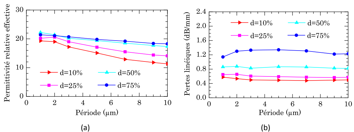
Figure 2.7 : a) Permittivité relative effective à 60 GHz et b) Pertes linéiques à 60 GHz en fonction de la période pour différents taux de remplissage, ( W = 7 \mu\text{m} , G = 50 \mu\text{m} , W_g = 10 \mu\text{m} , h = 1 \mu\text{m} , R = 10 \mu\text{m} ).
