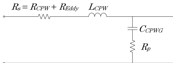
Figure 2.12 : Modèle équivalent RLRC choisi.
