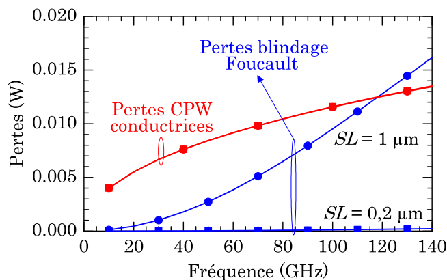
Figure 2.21 : Pertes dans une portion de longueur 1,2 \mu\text{m} de ligne S-CPW pour différents taux de remplissage du blindage flottant.
