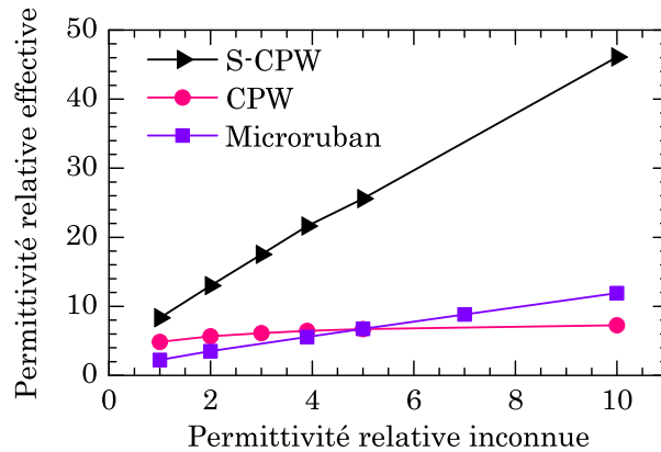
Figure 5.5 : Comparaison de la sensibilité de caractérisation de la permittivité relative avec différentes topologies de lignes (microruban, coplanaire et coplanaire à ondes lentes) à 60\ \text{GHz} .
