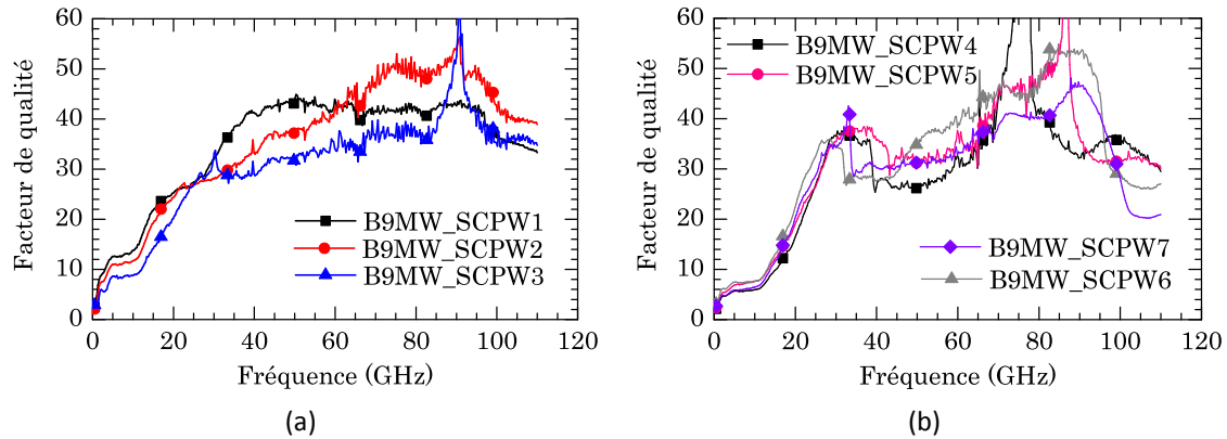
Figure 3.11 : Mesure du facteur de qualité pour différentes lignes à ondes lentes en technologie B9MW.
