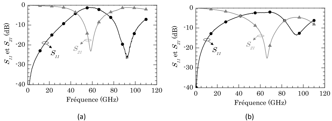
Figure 4.3 : Mesure de stubs S-CPW résonant à 60 GHz : a) Té-70Ω et b) Té-35Ω.
