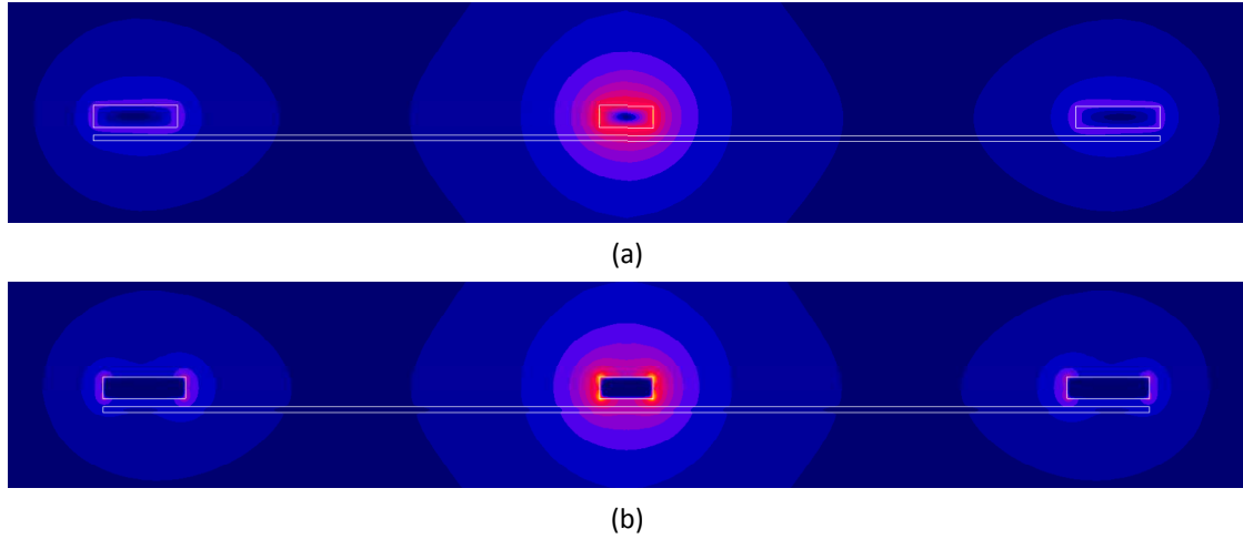
Figure 2.15 : Champ magnétique dans une ligne S-CPW, coupe dans un plan orthogonal à la propagation : a) en magnétostatique et b) à 60 GHz,
