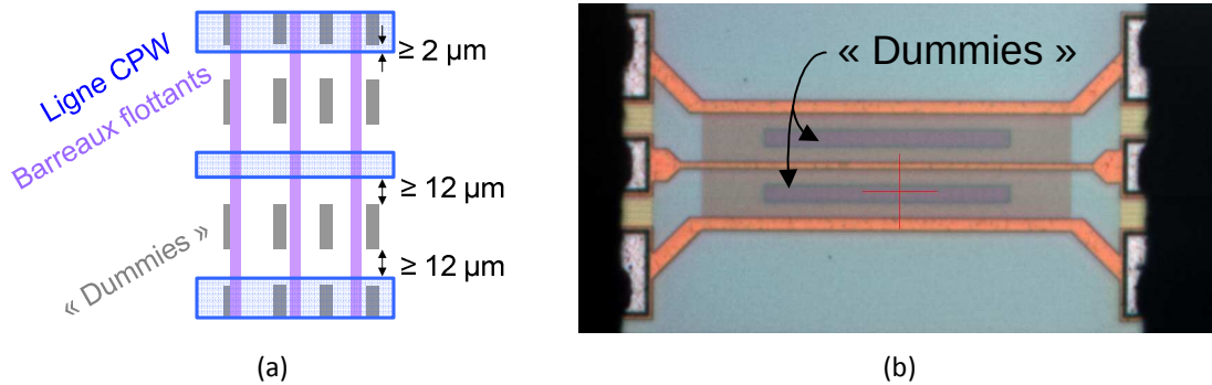
Figure 3.18 : a) Schéma de la disposition des dummies sur une couche métallique, b) photo d'une ligne B9MW_SCPW5 de longueur 200 \mu\text{m} comportant des dummies.
