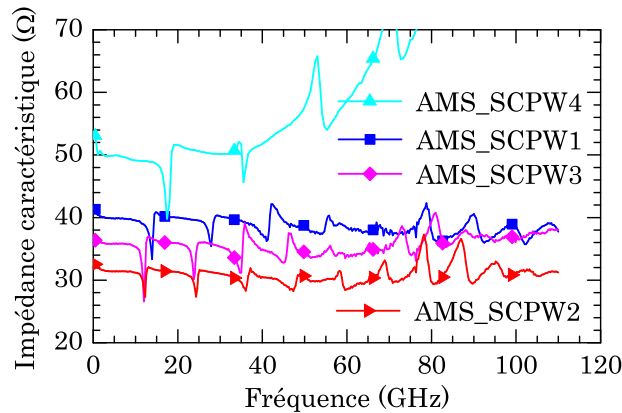
Figure 3.4 : Mesure de l'impédance caractéristique de quatre lignes de propagation en technologie AMS 0,35\ \mu\text{m} .
