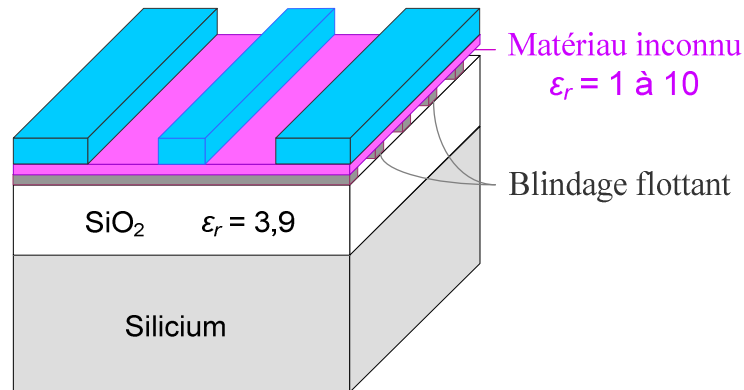
Figure 5.3 : Coupe transversale dans le plan d'un barreau flottant d'une ligne S-CPW support de test.
