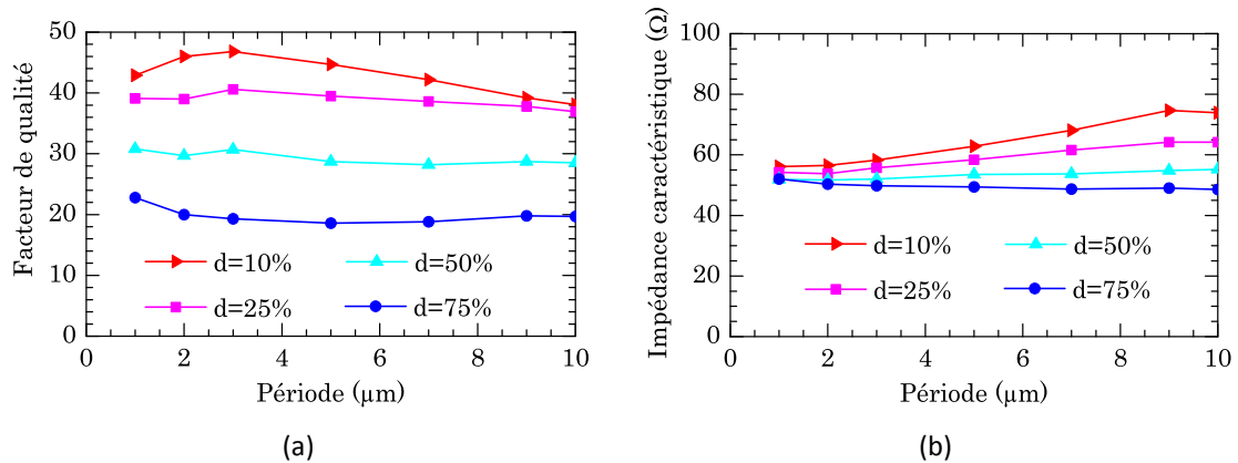
Figure 2.8 :a) Facteur de qualité à 60 GHz et b) impédance caractéristique à 60 GHz en fonction de la période pour différents taux de remplissage, ( W = 7 \mu\text{m} , G = 50 \mu\text{m} , W_g = 10 \mu\text{m} , h = 1 \mu\text{m} , R = 10 \mu\text{m} ).
