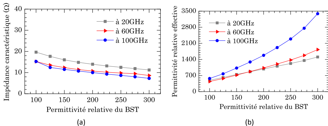
Figure 5.9 : (a) Impédance caractéristique et (b) permittivité relative effective en fonction de la permittivité relative du BST, à différentes fréquences.
