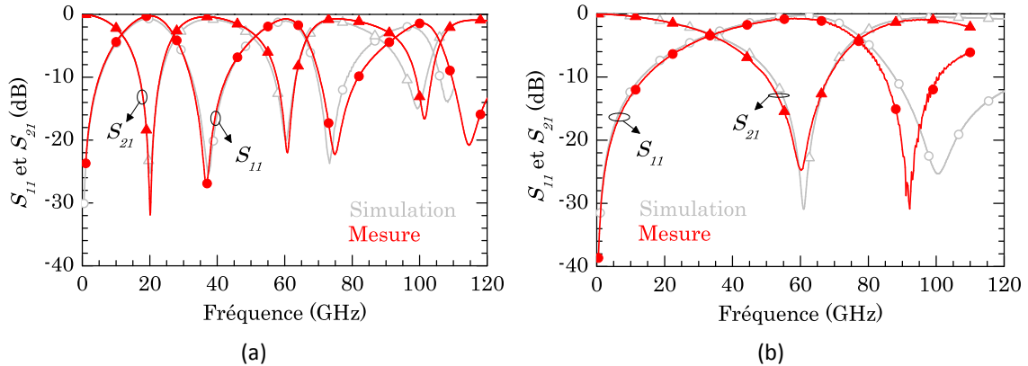
Figure 4.6 : Mesure d'un stub en S-CPW avec une jonction microruban : a) 20 GHz, b) 60 GHz.
