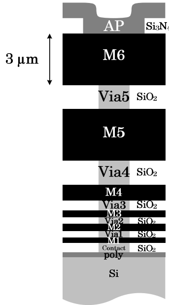
Figure 3.7 : Empilement de la technologie BiCMOS9MW de STMicroelectronics.
