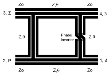
Figure 4.18 : Schéma d'un rat-race en CPW comportant un inverseur d'impédance, [Chirala, 2006a].
