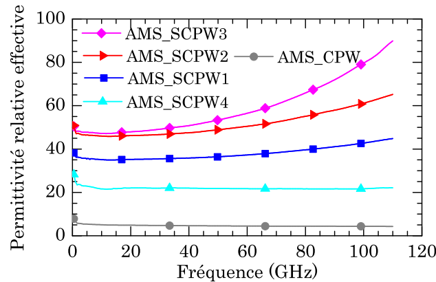
Figure 3.5 : Mesure de la permittivité relative effective de quatre lignes de propagation S-CPW et d'une ligne CPW en technologie AMS 0,35 \mu\text{m} .
