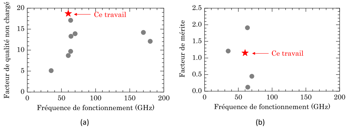
Figure 4.12 : a) Facteur de qualité non chargé et b) facteur de mérite en fonction de la fréquence pour des filtres de la littérature.
