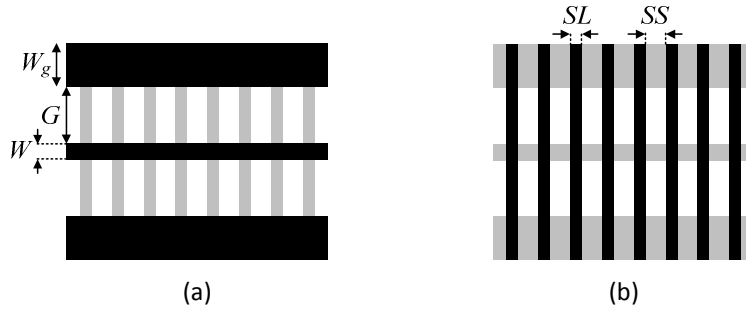
Figure A1.1 : Vue schématique d'une ligne à ondes lentes en technologie PCB, a) Vue de dessus, b) Vue de dessous.
