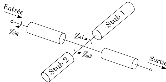
Figure 4.7 : Schéma d'un filtre DBR d'ordre 1.
