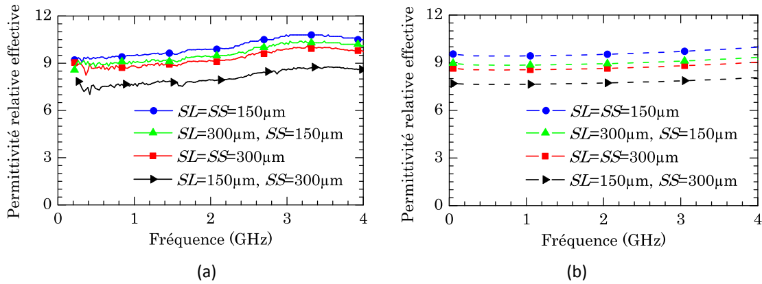
Figure A1.5 : Permittivité relative effective a) mesurée et b) simulée en fonction de la fréquence pour différents couples de SL et SS avec W = 1,5 \text{ mm} , G = 2 \text{ mm} , h = 203 \text{ }\mu\text{m} .
