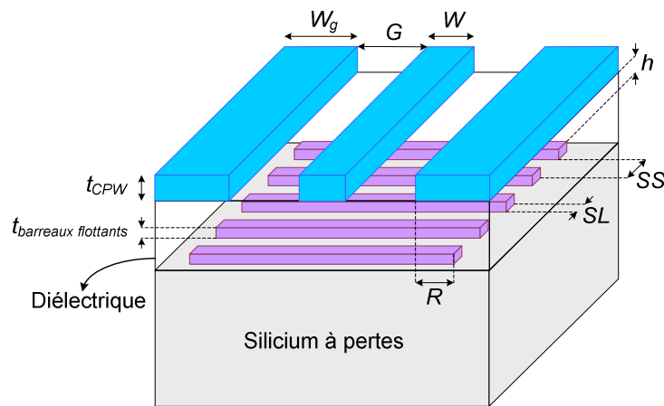
Figure 2.2 : Dimensions physiques d'une ligne de propagation S-CPW.
