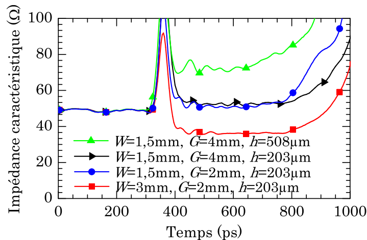
Figure A1.6 : Mesures TDR d'impédances caractéristiques pour des lignes avec SL = SS = 150 \mu\text{m} .
