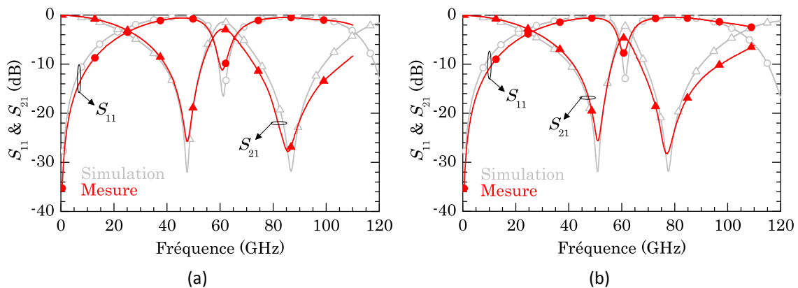
Figure 4.10 : Mesures des paramètres S de deux résonateurs DBR à 60 GHz : a) large bande passante et faibles pertes d'insertion, b) bande passante étroite et pertes d'insertion élevées.
