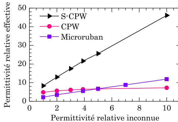
Figure 5.5 : Comparaison de la sensibilité de caractérisation de la permittivité relative avec différentes topologies de lignes (microruban, coplanaire et coplanaire à ondes lentes) à 60 GHz.
