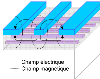
Figure 1.6 : Topologie d'une ligne à ondes lentes et allure du champ électromagnétique dans la structure.
