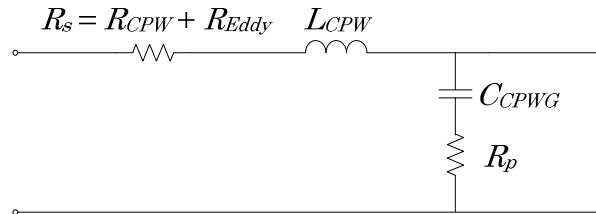
Figure 2.12 : Modèle équivalent RLRC choisi.
