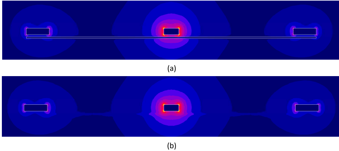
Figure 2.16 : Représentation du champ magnétique à 500 GHz dans le sens orthogonal à la propagation : a) coupe au milieu d'un barreau flottant et b) coupe entre deux barreaux flottants, ( W = 7 \mu\text{m} , G = 50 \mu\text{m} , W_g = 10 \mu\text{m} , h = 1 \mu\text{m} , R = 10 \mu\text{m} , SL = 0,6 \mu\text{m} , SS = 1 \mu\text{m} ).
