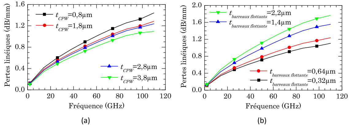
Figure 2.9 : Effet de l'épaisseur de a) la ligne CPW et b) du blindage flottant sur l'atténuation linéique, ( W = 7 \mu m , G = 50 \mu m , W_g = 10 \mu m , R = 10 \mu m , SL = 0.6 \mu m , SS = 1 \mu m ).
