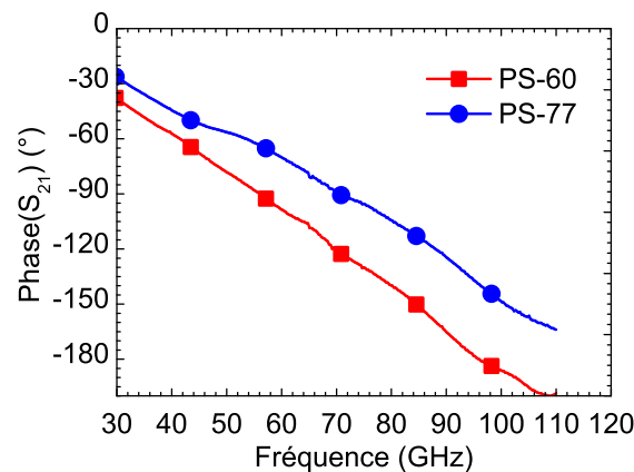
Figure 4.17 : Mesure de la phase de S_{21} après « de-embedding ».
