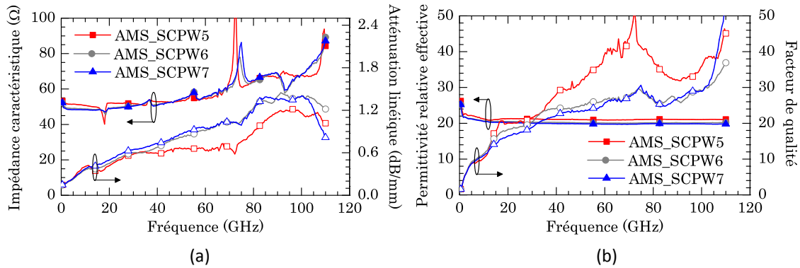
Figure 3.15 : Mesure pour trois largeurs de plans de masse différentes de a) l'impédance caractéristique et l'atténuation linéique et b) la permittivité relative effective et le facteur de qualité.
