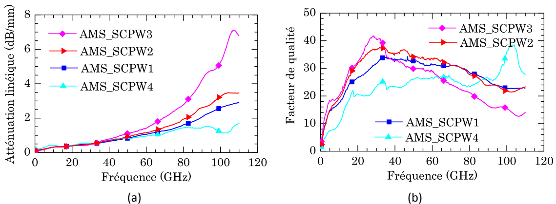
Figure 3.6 : Extraction à partir des mesures pour les quatre lignes de propagation S-CPW en technologie AMS 0,35 \mu\text{m} de l'atténuation linéique et a) du facteur de qualité b).
