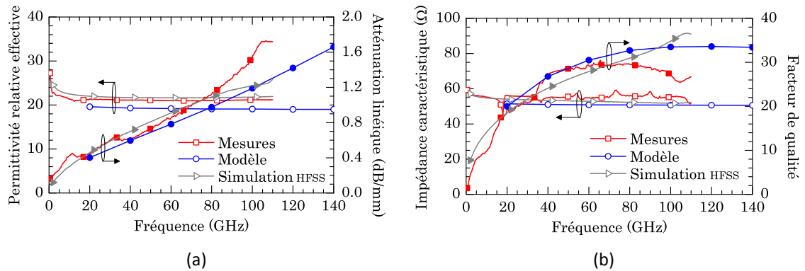
Figure 2.18 : Comparaison des résultats de mesure, de simulation et du modèle pour a) la permittivité relative effective et l'atténuation linéique, b) l'impédance caractéristique et le facteur de qualité, ( W = 7 \mu\text{m} , G = 50 \mu\text{m} , W_g = 10 \mu\text{m} , h = 1 \mu\text{m} , R = 10 \mu\text{m} , SL = 0,6 \mu\text{m} , SS = 1 \mu\text{m} ).
