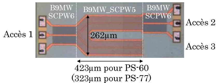
Figure 4.14 : Photographie du diviseur de puissance PS-60 et dimensions pour PS-77.
