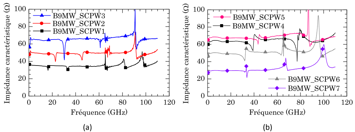
Figure 3.8 : Mesure de l'impédance caractéristique pour différentes épaisseurs de dioxyde en technologie B9MW.
