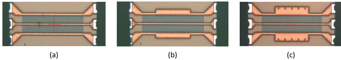
Figure 3.14 : Photos des lignes à ondes lentes avec différentes largeurs de plan de masse : a) AMS_SCPW5 : W_g = 10 \mu\text{m} , b) AMS_SCPW6 : W_g = 30 \mu\text{m} et c) AMS_SCPW7 : W_g = 50 \mu\text{m} .
