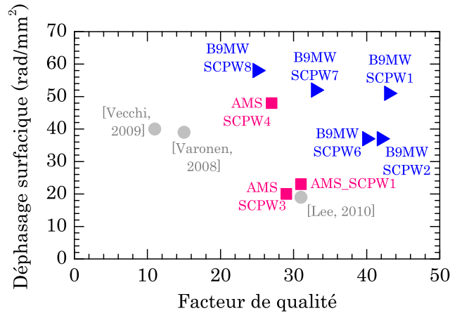
Figure 3.13 : Déphasage surfacique en fonction du facteur de qualité à 60 GHz.
