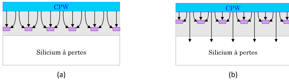
Figure 2.6 : Schéma de répartition des lignes de champ électrique dans une ligne S-CPW pour différents rapports SS/h , coupe dans le sens de la propagation.
