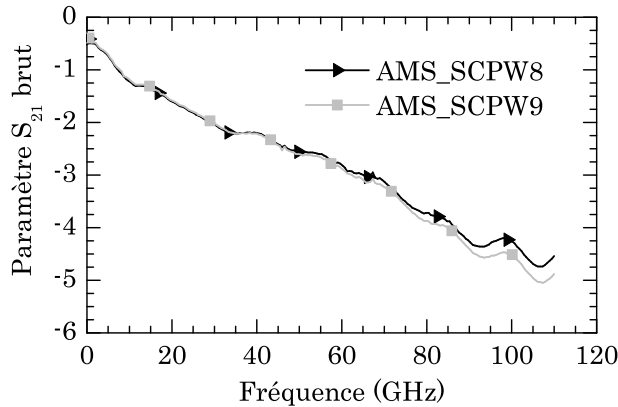
Figure 3.17 : Mesure du paramètre de transmission pour deux épaisseurs de blindage différentes.
