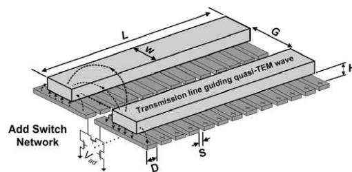
Figure 1.10 : Lignes couplées à ondes lentes accordables, d'après [LaRocca, 2008].
