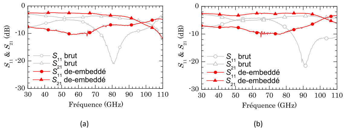
Figure 4.16 : Mesure du module des paramètres S bruts et « de-embeddés » : a) PS-60, b) PS-77.
