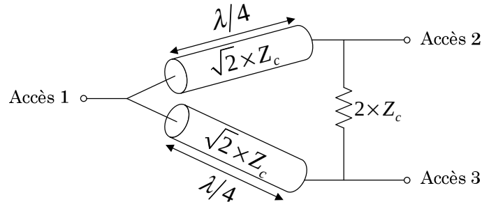
Figure 4.13 : Diviseur de puissance de Wilkinson.
