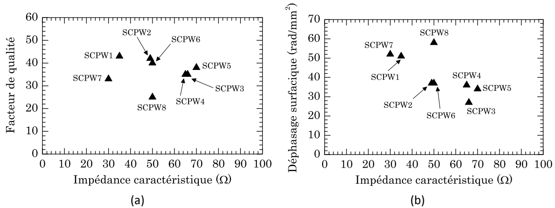
Figure 3.23 : a) Facteur de qualité à 60 GHz et a) déphasage surfacique à 60 GHz en fonction de l'impédance caractéristique pour les lignes à ondes lentes réalisées en technologie B9MW.
