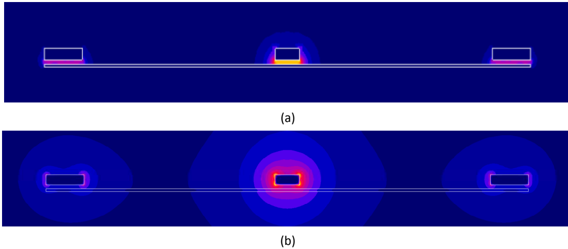
Figure 2.13 : Allure du champ électromagnétique simulé d'une ligne à ondes lentes : champ électrique (a) et magnétique(b) dans un plan transversal à celui de la propagation, ( W = 7 \mu\text{m} , G = 50 \mu\text{m} , W_g = 10 \mu\text{m} , h = 1 \mu\text{m} , R = 10 \mu\text{m} , SL = 0,6 \mu\text{m} , SS = 1 \mu\text{m} ).
