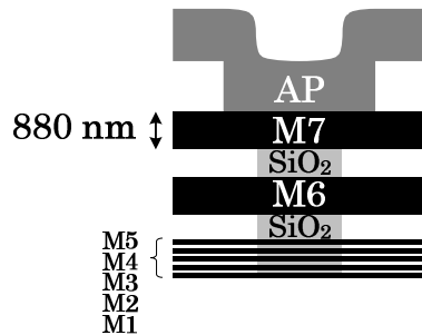
Figure 5.1 : Empilement de la technologie CMOS 28 nm de STMicroelectronics.
