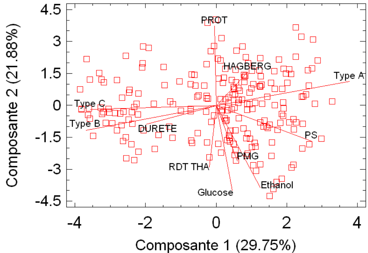
Figure 33. Analyse en composantes principales des lignées françaises réalisée sur les valeurs moyennes des données multilocales pluriannuelles et des traitements.
