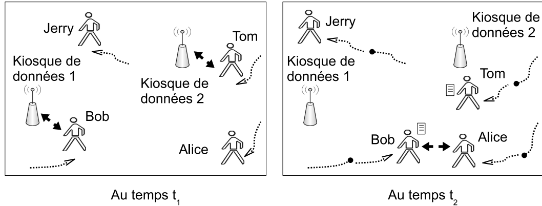
FIGURE B.2 – Diffusion de contenu dans un DTN avec la présence des kiosques de données.
