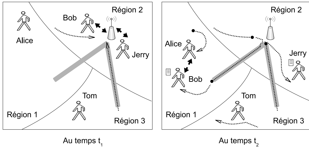
FIGURE B.3 – Diffusion de contenu dans un DTN avec la présence des kiosques de données associé à un plan de métro.
