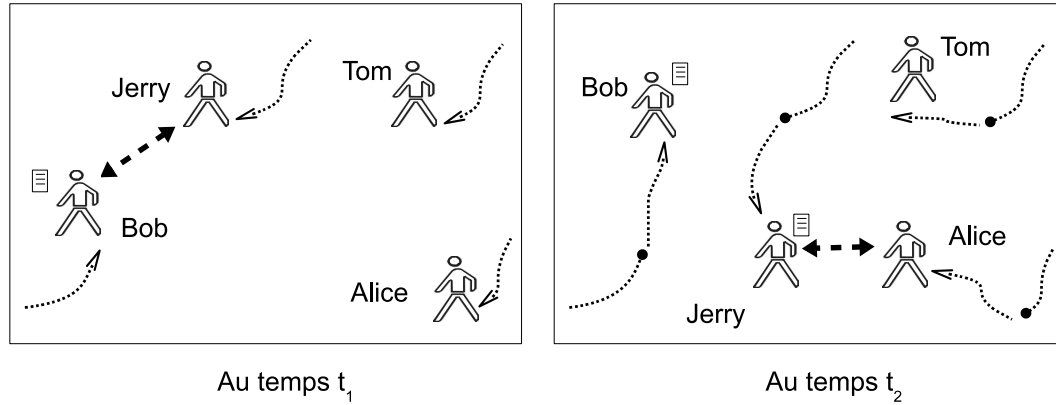
FIGURE B.1 – Diffusion de contenu dans un DTN sans la présence des kiosques de données.
