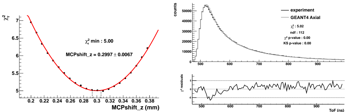
FIGURE V.37 – À gauche : détermination de \Delta z_{MCP} par la minimisation de la statistique du test \chi^2_P pour le modèle Axial à température fixe C_t = 1.05 . À droite : test \chi^2_P de la distribution de temps de vol correspondant au meilleur ajustement de la distance nuage-détecteur.
