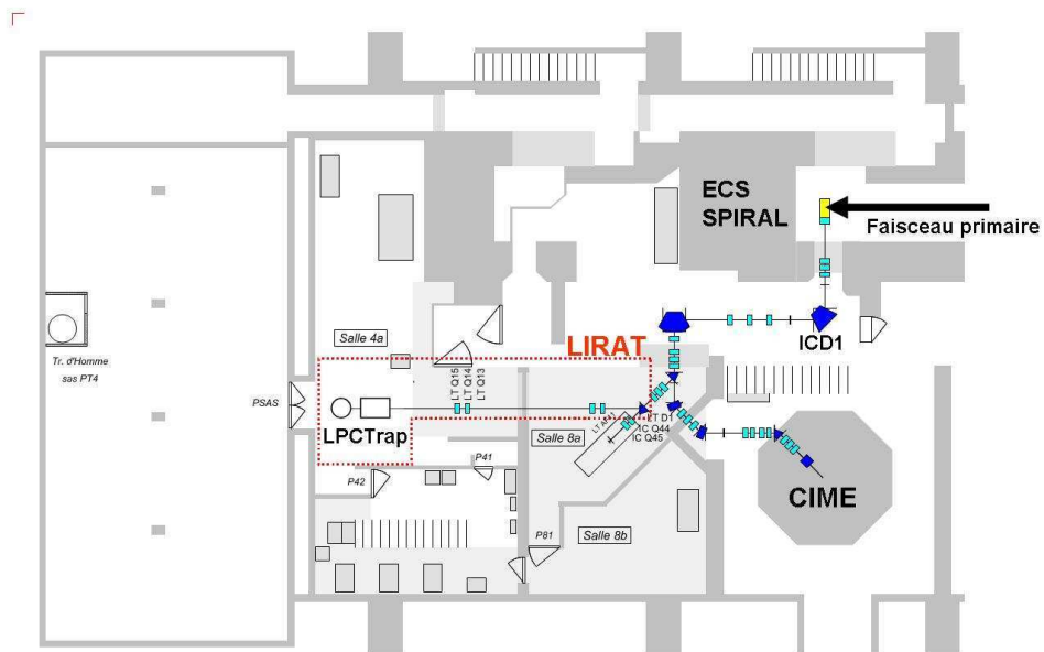
FIGURE II.6 – Implantation de la ligne basse énergie LIRAT.
