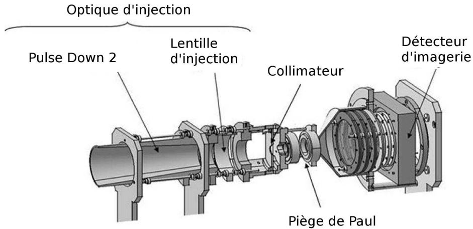
FIGURE II.12 – Système d’injection dans le piège.
