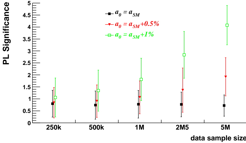
FIGURE IV.9 – Significativité du test de vraisemblance profilée H_A/H_{A+T} en fonction de la statistique pseudo-expérimentale et pour trois valeurs de a_0 .
