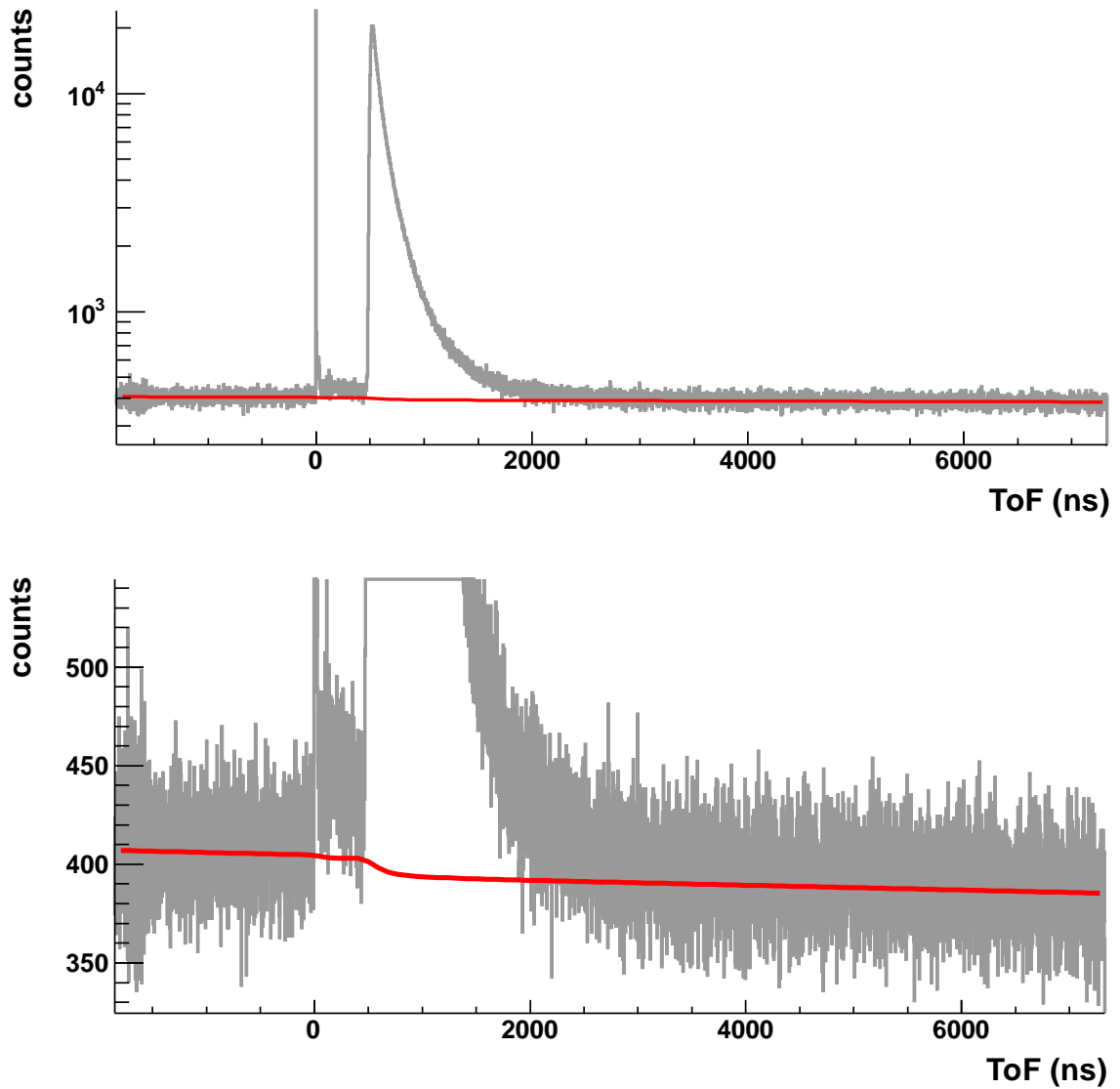
FIGURE V.29 – Forme de la composante des coïncidences fortuites ajustée sur la distribution brute de temps de vol des événements en coïncidence. En haut : pleine échelle logarithmique, en bas : zoom sur la base de la distribution.
