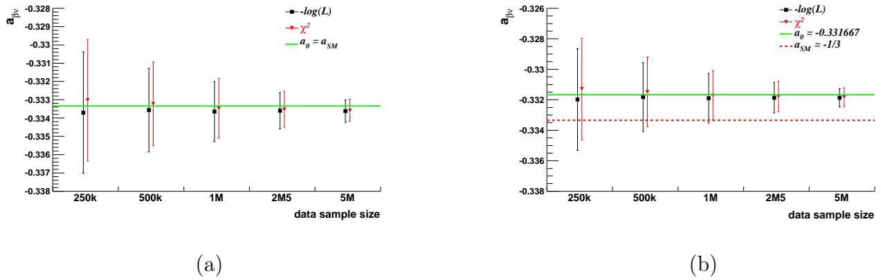
FIGURE IV.7 – Évolution de la moyenne de l'estimation de a_{\beta\nu} en fonction de la statistique expérimentale dans les cas a) a_0 = a_{SM} et b) a_0 = -0.331667 .
