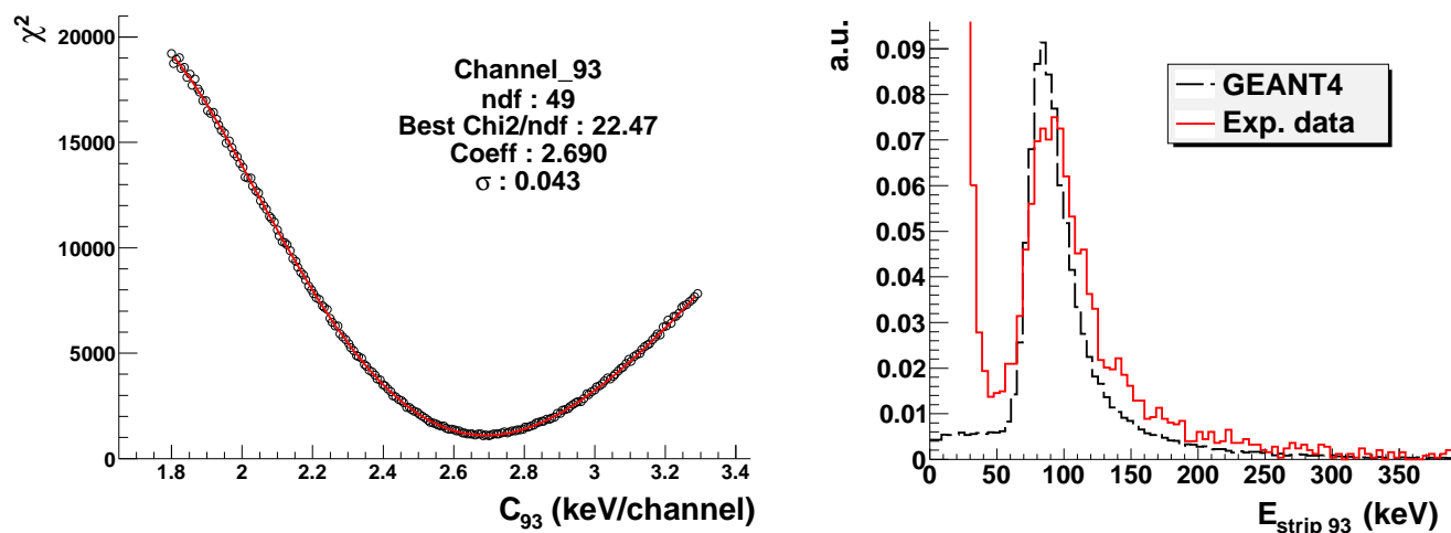
FIGURE V.6 – À gauche : détermination du coefficient de calibration de la piste numéro 93 à l’aide de la comparaison entre le spectre expérimental et celui simulé par GEANT4 par la méthode du \chi^2 . À droite : comparaison des spectres correspondant au meilleur ajustement du coefficient de calibration.
