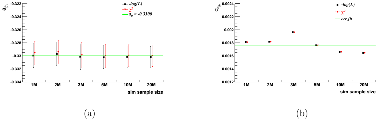
FIGURE IV.5 – a) Valeurs moyennes des estimations de a_{\beta\nu} en fonction de la taille des échantillons simulés. L'échantillon de pseudo-données contient 10^6 événements. (b) Écart-types de l'estimateur d' a_{\beta\nu} en fonction de la taille des échantillons simulés. La ligne horizontale est l'erreur fournie par la procédure d'ajustement.
