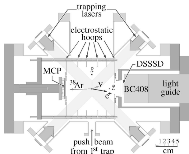
FIGURE I.11 – Schéma de la chambre de détection utilisée dans l'expérience de TRIUMF [G + 05b].
