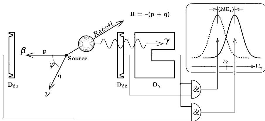
FIGURE I.14 – Schéma du principe de détection en coïncidence du double décalage Doppler
