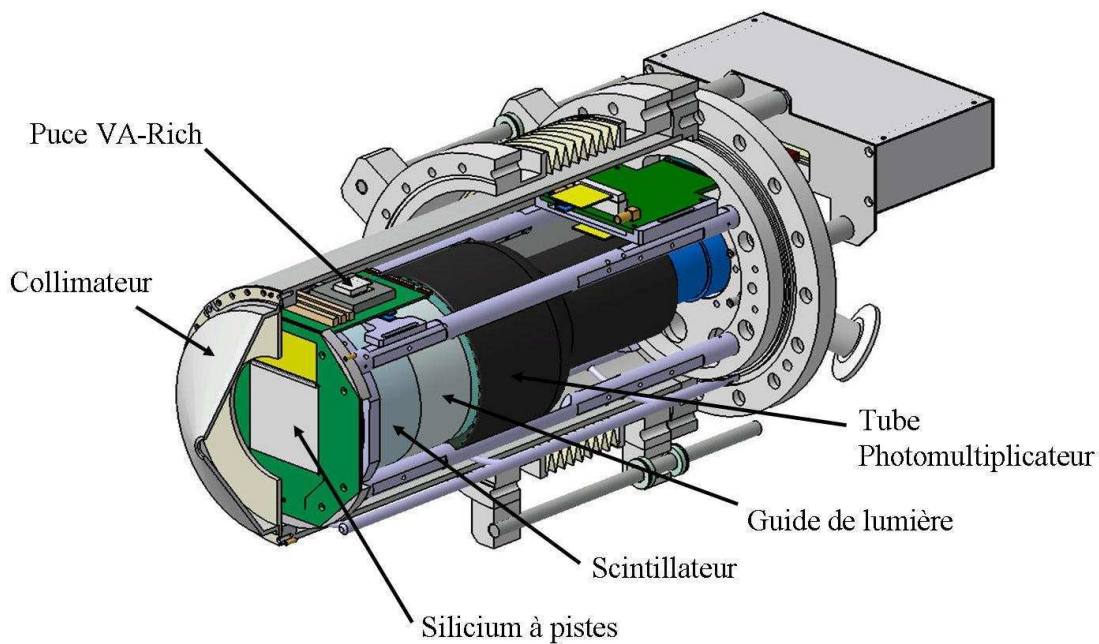
FIGURE II.26 – Le télescope \beta et sa structure. La découpe effectuée permet de distinguer les deux étages constituant le détecteur : le silicium à pistes et ses puces électroniques pour traiter les 120 signaux, suivi du scintillateur plastique couplé au tube photomultiplicateur.
