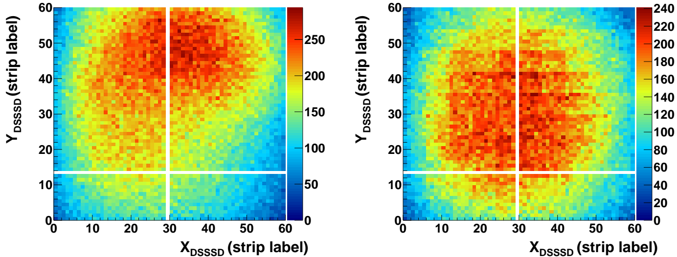
FIGURE V.12 – Position du \beta donnée par le silicium à pistes pour des événements en coïncidence dont la charge codée par le QDC du télescope \beta est supérieure à 7000 canaux avant (gauche) et après (droite) correction du gain du scintillateur.
