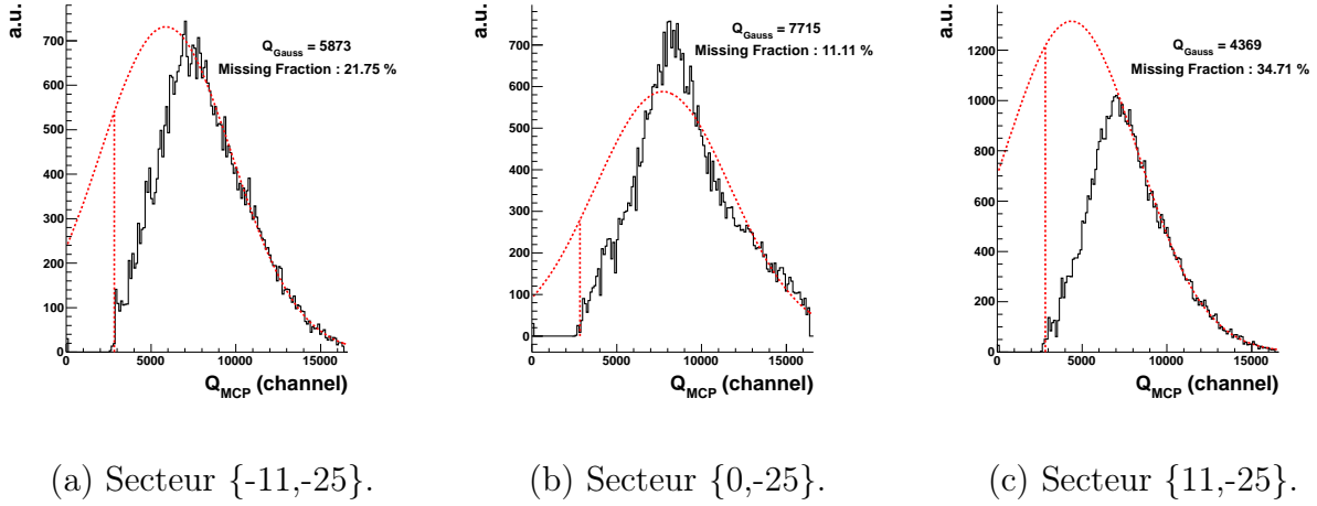
FIGURE V.26 – Spectres en charge présentant une déformation dont l'origine n'est pas la coupure du seuil électronique (indiqué par un trait pointillé vertical).
