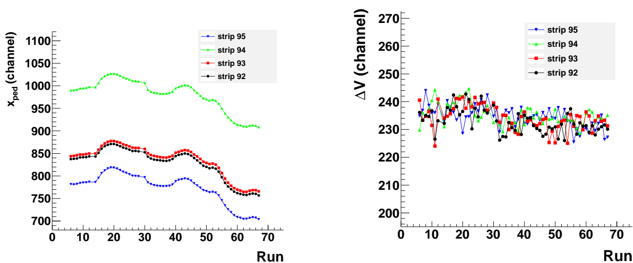
FIGURE V.4 – Évolution de la position du piédestal (gauche) et de \Delta Q (droite) des pistes 92, 93, 94 en fonction des runs.
