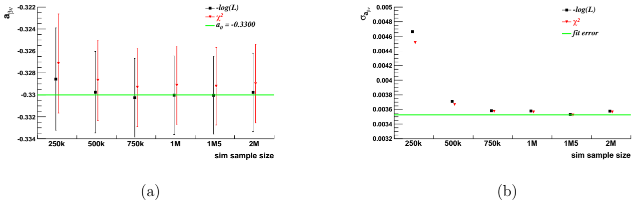
FIGURE IV.6 – Idem que la figure précédente hormis que l'échantillon de pseudo-données ne contient que 2.5 \times 10^5 événements.
