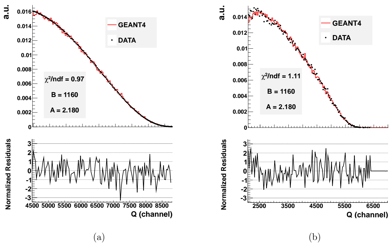
FIGURE V.14 – Meilleurs ajustements obtenus pour les coefficients de la fonction de calibration pour les événements de décroissances d' {}^6\text{He}^+ sans coïncidence (à gauche) et ceux avec la source {}^{90}\text{Sr} (à droite).
