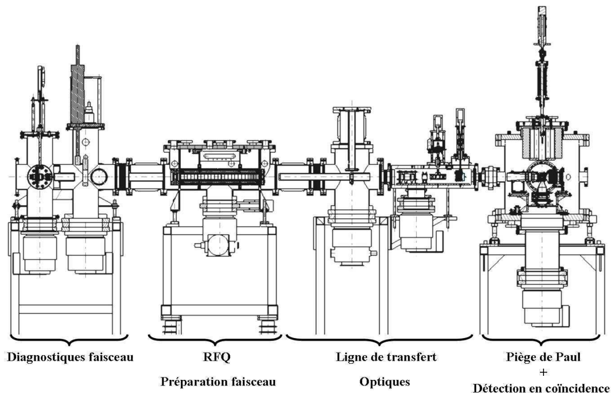
FIGURE II.8 – Schéma de la ligne de préparation du faisceau.
