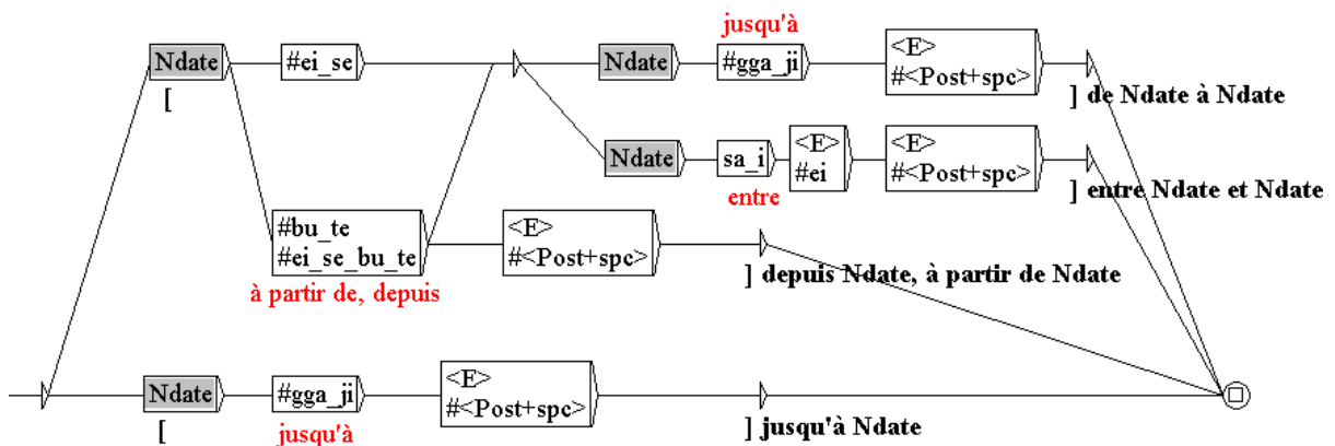
Figure 47 : Graphe bute-ggaji
