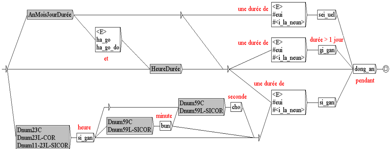
Figure 40 : Graphe DnumNtpsDongan
