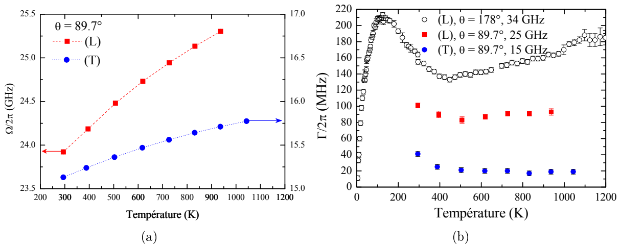
FIGURE 2.17 – (a) Fréquences Brillouin des modes TA et LA en fonction de la température avec un angle de diffusion de \theta = 89,7^\circ . Les lignes pointillées sont des guides pour les yeux. (b) Largeurs Brillouin en fonction de la température, pour différentes polarisations et géométries de diffusion.
