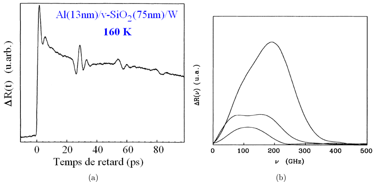
FIGURE 3.11 – Variations des fluctuations de réflectivité \Delta R en fonction du retard pompe-sonde, mesurées à 160 K dans le cas d’une couche de silice d’épaisseur 75 nm (a) et représentation de la transformée de Fourier des trois échos (b), d’après [163].
