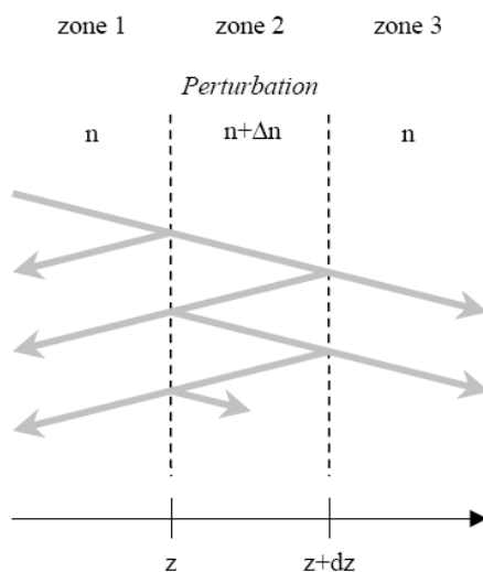
FIGURE 3.6 – Représentation schématique d'une perturbation située entre z et z + dz et produisant une variation d'indice \Delta n (figure extraite de la référence [193]).
