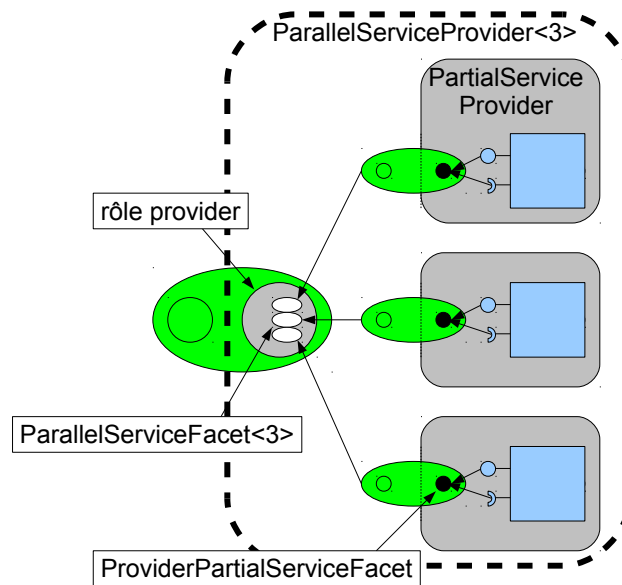
FIGURE 7.21 – Exemple d'instance de ParallelServiceProvider avec un degré de réplification de 3. Elle contient 3 instances du composant PartialServiceProvider . Les connexions ouvertes qu'elles exposent sont regroupées au sein d'une bundle de type ParallelServiceFacet<3> . Ce bundle remplit le rôle provider de la connexion ouverte exposée par le composant.
