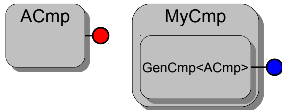
FIGURE 4.4 – Exemple de spécialisation du type de composant GenCmp avec le type de composant ACmp comme argument
