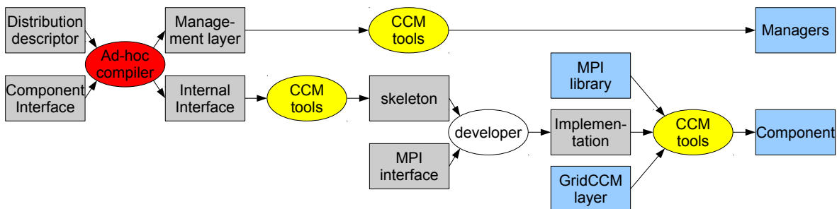
FIGURE 3.1 – Chaîne de compilation dédiée de GRIDCCM
