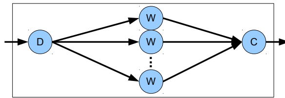
FIGURE 3.3 – Le squelette de ferme de tâches comportant un distributeur (D) qui répartie le flux de données en entrée entre les travailleurs (W) qui effectuent le calcul et un collecteur (C) qui ré-assemble le flux en sortie.
