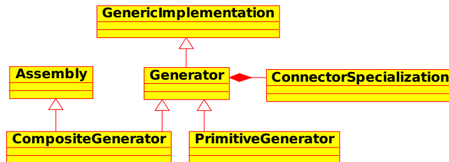
FIGURE 5.9 – Présentation de la modélisation du concept de générateur.
