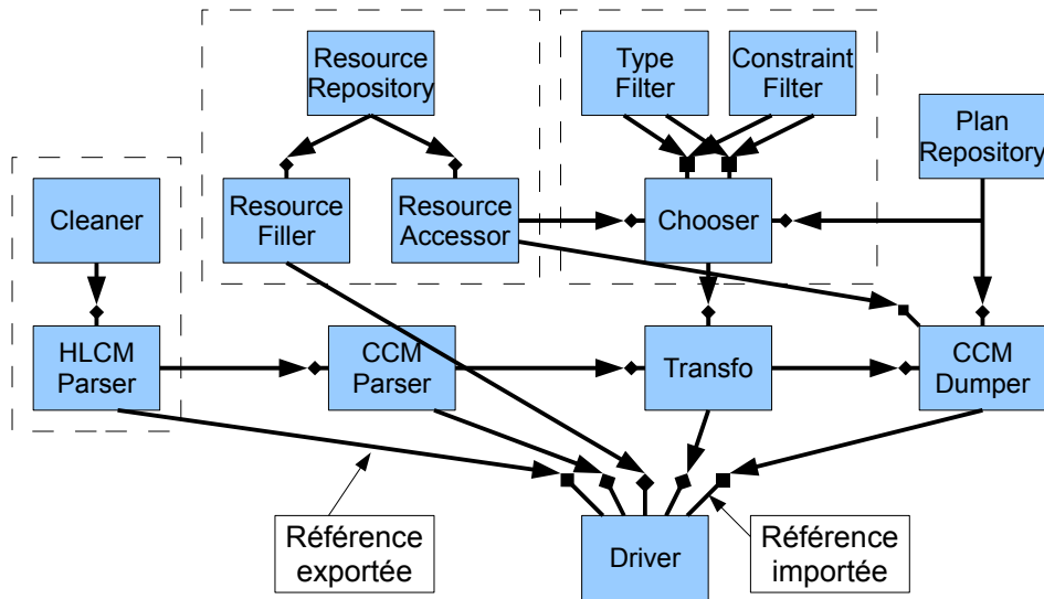
FIGURE 6.8 – Présentation de l'architecture de HLCM i /CCM en terme d'assemblage de composants LCCM j . Les rectangles en tirets représentent des regroupements logiques d'instances qui constitueraient de bon candidats à la création de composite dans un modèle comportant ce concept.
