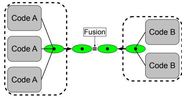
FIGURE 5.6 – Fusion des connexions exposées par deux composites pour ne plus former qu'une unique connexion logique.
