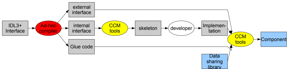
FIGURE 3.2 – Chaîne de compilation dédiée pour la mise en œuvre du partage de données dans CCM
