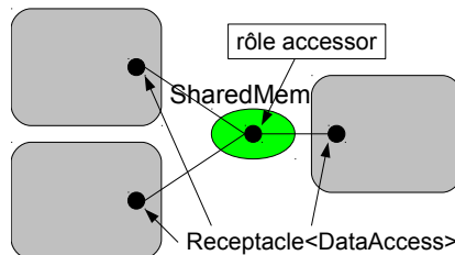
FIGURE 7.3 – Assemblage intermédiaire où tous les composants participent à une même connexion indépendamment de leur distribution initiale au sein de la hiérarchie.
