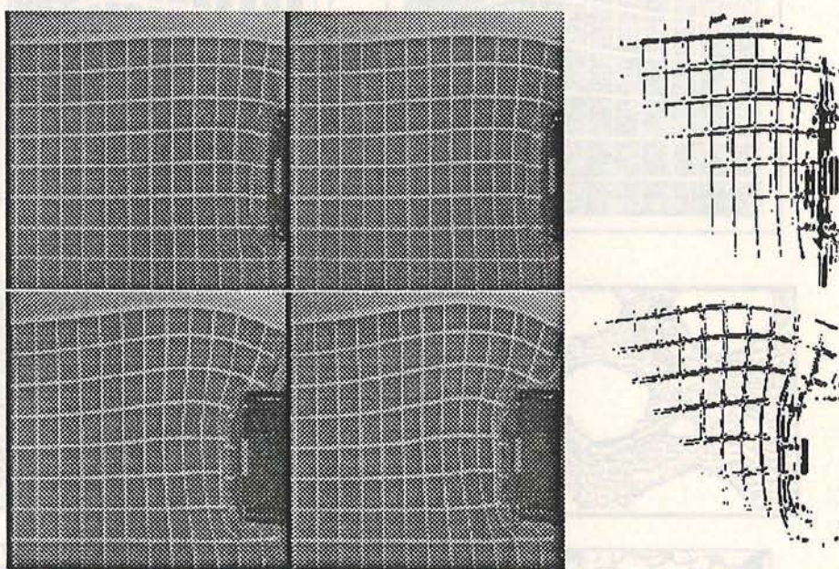
Figure III.2 : Séquence d'image d'une modélisation analogique avec détermination d'une zone de mouvement. Les zones (en noir) représentées sur les images binaires (c et d) traduisent les zones qui se sont déplacées entre les deux images (schématiquement c = b-a et d=e-b ).
