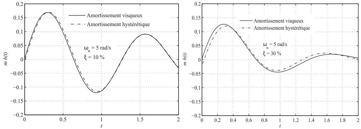
Figure 1.4 : Fonction de transfert h(t) dans le domaine temporel
