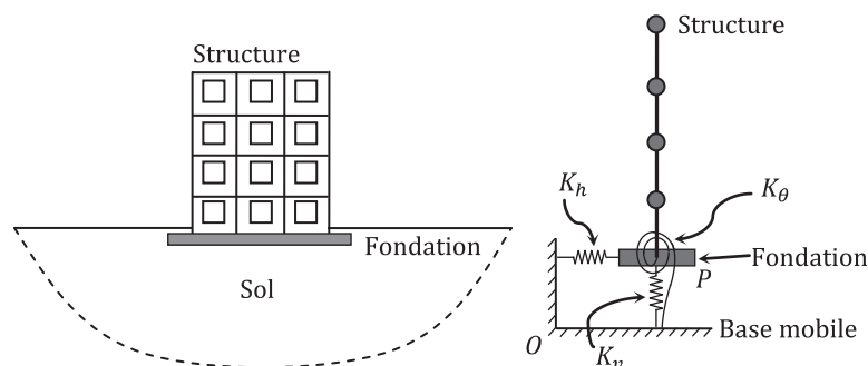
Figure 2.1 : Schématisation de l'interaction sol-structure
