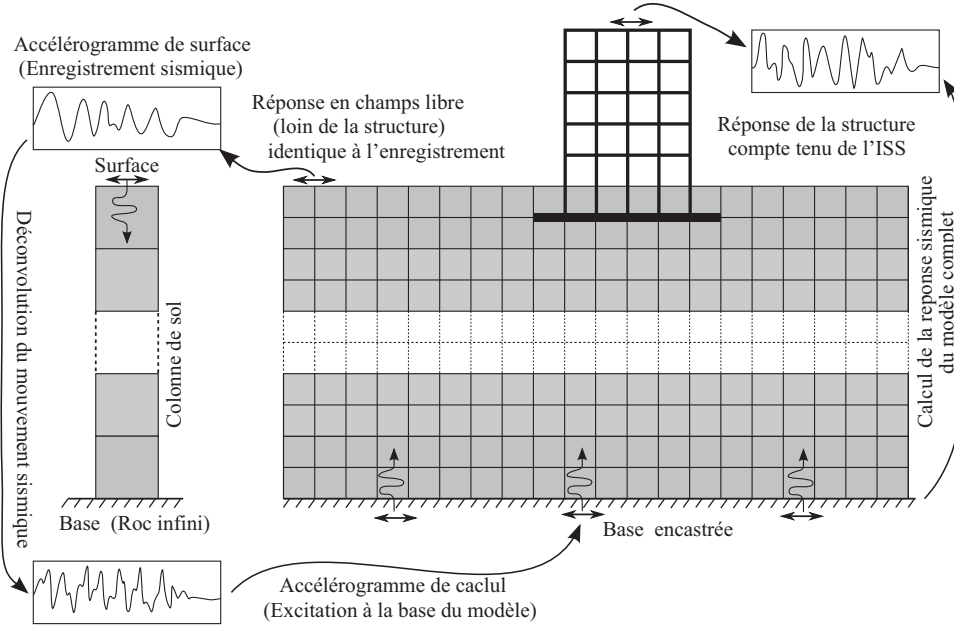
Figure 2.3 : Modélisation de l'ISS par le méthode globale [104]
