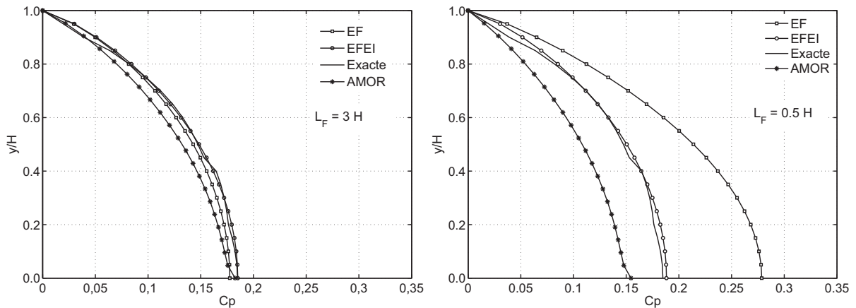
Figure 3.9 : Pression maximale normalisée par la pression hydrostatique
