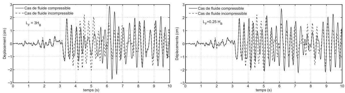
Figure 5.14 : Effet de la compressibilité du fluide sur les déplacements du barrage (Modèle FE-IE)
