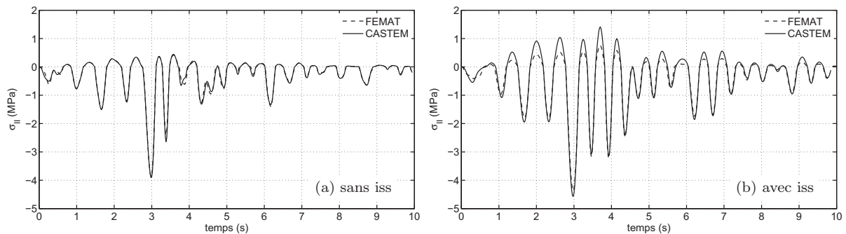
Figure 2.12 : Variations de la contrainte minimale au pied amont du barrage
