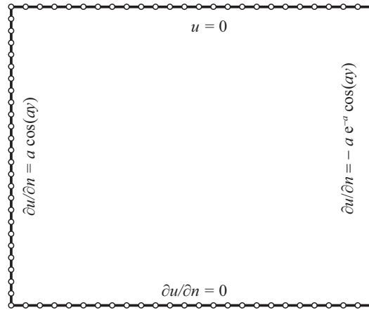
Figure 4.9 : Géométrie et définition du problème de validation
