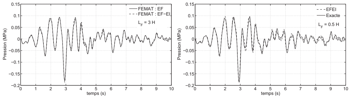
Figure 3.7 : Comparaison entre le modèle de couplage éléments finis - éléments infinis et solution exacte
