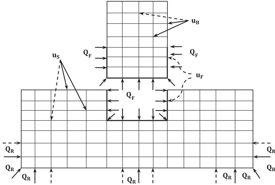
Figure 2.5 : Sous-Structure
