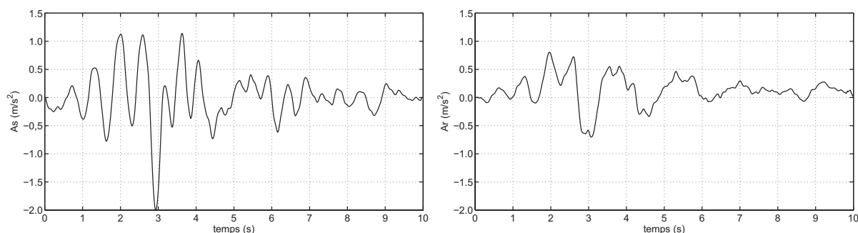
Figure 2.7 : Accélérogrammes enregistré en champs libre et calculé en profondeur à 300m
