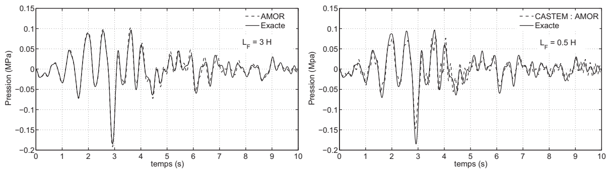
Figure 3.8 : Comparaison entre les éléments infinis et l'opérateur AMOR de CASTEM
