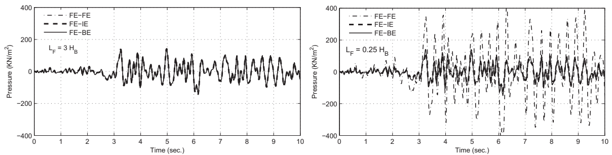
Figure 5.10 : Histoire de réponse temporelle des pressions au pied amont du barrage
