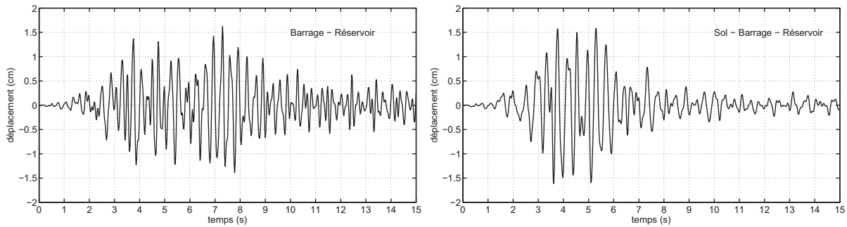
Figure 6.10 : Effet de l'IFS et de l'ISS sur les déplacements en crête
