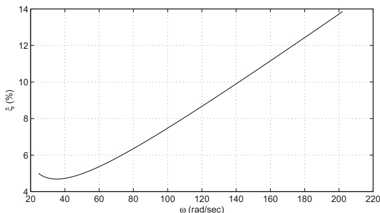
Figure 1.5 : Evolution du taux d'amortissement de Rayleigh
