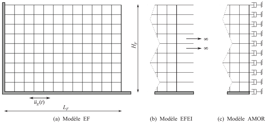
Figure 3.4 : Modèle FEM du réservoir
