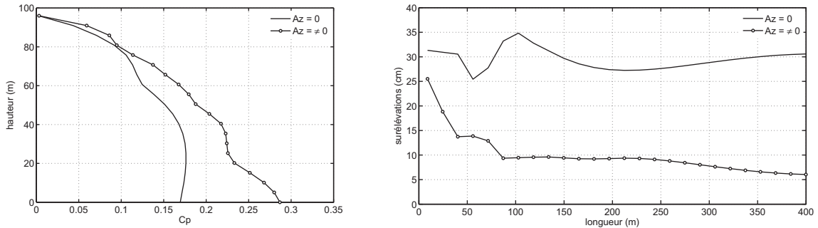
Figure 6.17 : Effet de la composante verticale sur la distribution des pressions sur le parement du barrage et les fluctuations de la surface libre
