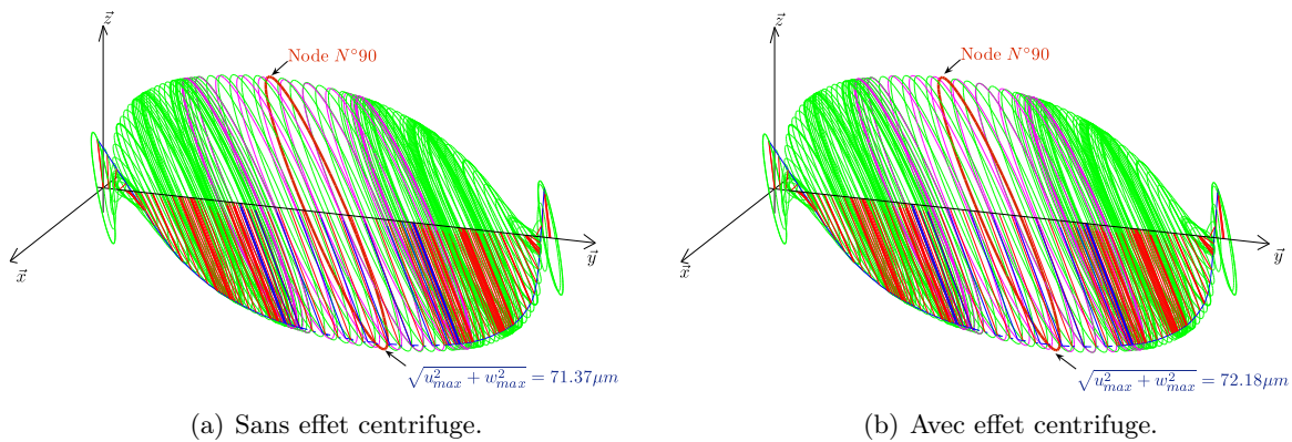
FIGURE 5.25 – Déformée du rotor à \dot{\phi}_r = 3\,250 rpm, configuration \mathcal{C}_1 .
