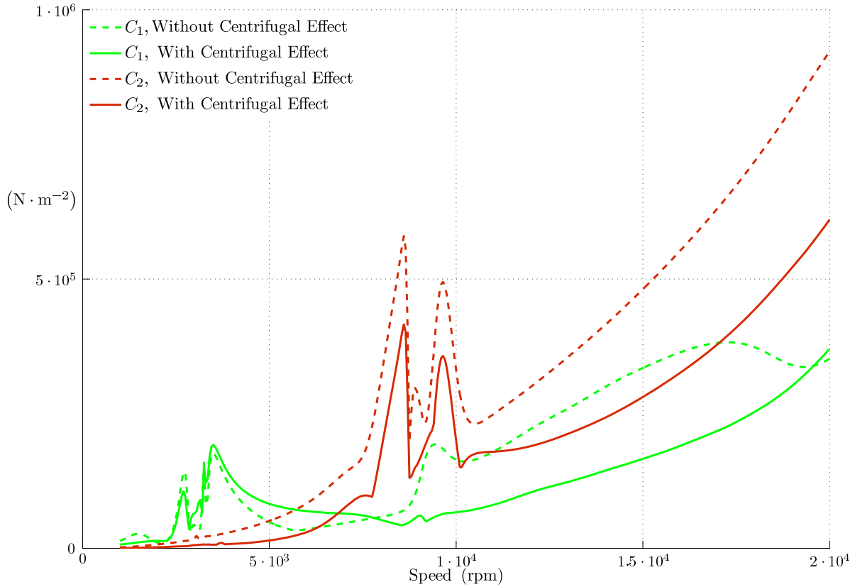
FIGURE 5.30 – Évolution du maximum des contraintes de \mathcal{V} on \mathcal{M} ises des tirants due uniquement aux balourds, pour les configurations \mathcal{C}_1 (—) et \mathcal{C}_2 (---).
