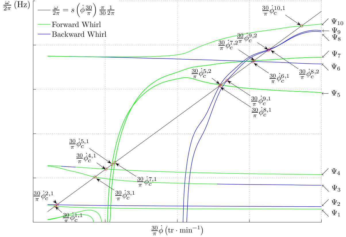
FIGURE 2.17 – Repérage de vitesses critiques de rotation (○) sur un diagramme de Campbell, induites par une excitation asynchrone de facteur s .
