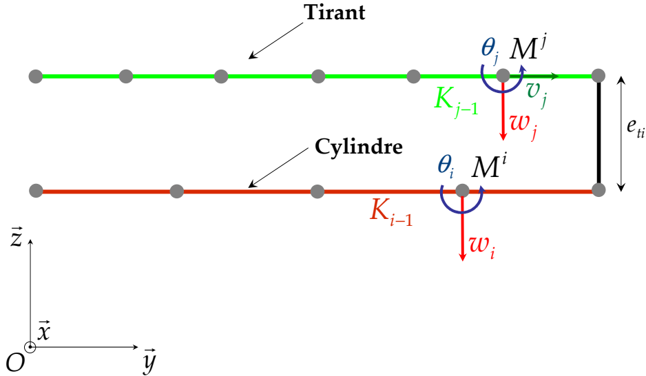
FIGURE B.4 – Modèle éléments finis \mathcal{M}_1 . ■ : Éléments de flexion-extension, ■ : Éléments de flexion, ■ : Élément rigide \Rightarrow Relation cinématique.
