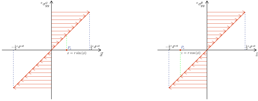
(a) Répartitions des champs de contraintes e \sigma_{yy}^{\psi} .
