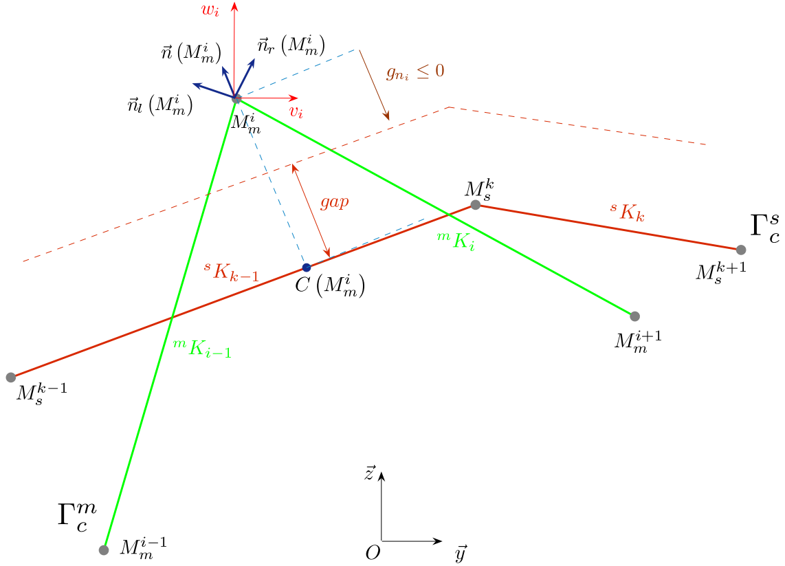
FIGURE 5.6 – Représentation de la normale de contact \bar{n}(M_m^i) dans une situation d'interpénétration des domaines maître \Omega_m et esclave \Omega_s .
