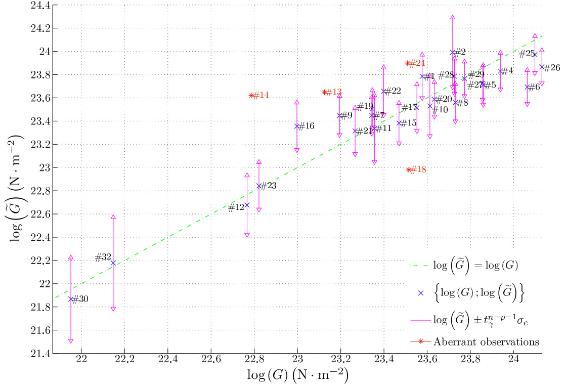
FIGURE 4.43 – Loi logarithmique du module de Coulomb \tilde{G} en fonction des modules de Coulomb identifiés G . R^2 = 0.897519 , n = 26 , p = 6 , \gamma = 0.025 .
