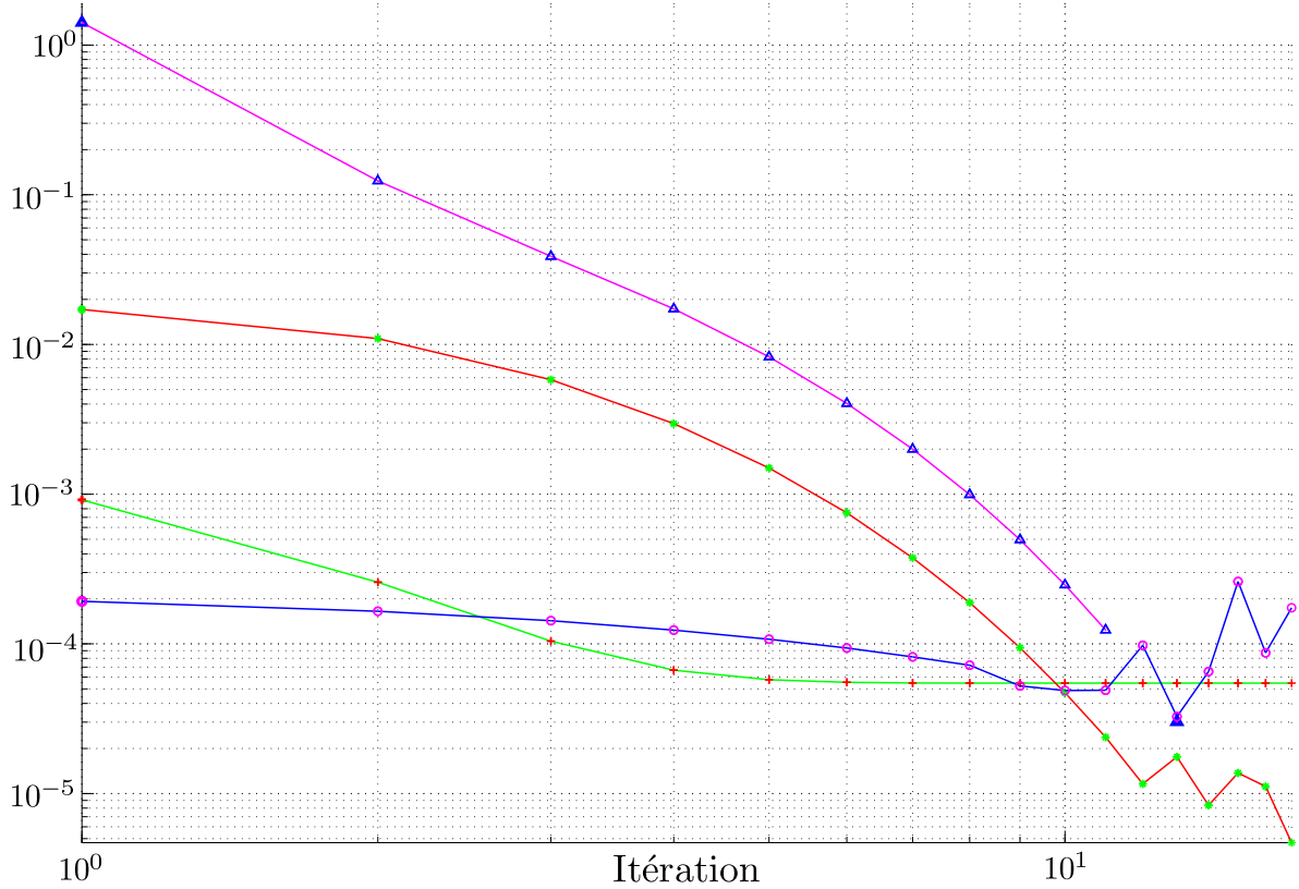
FIGURE E.3 – Évolution de la norme de la différences des itérés successifs ( \Delta ), fonctionnelle (+), norme de gradient (*) et paramètre d'amortissement ( \circ ) au cours des 17 itérations. La convergence est atteinte en 219 s.
