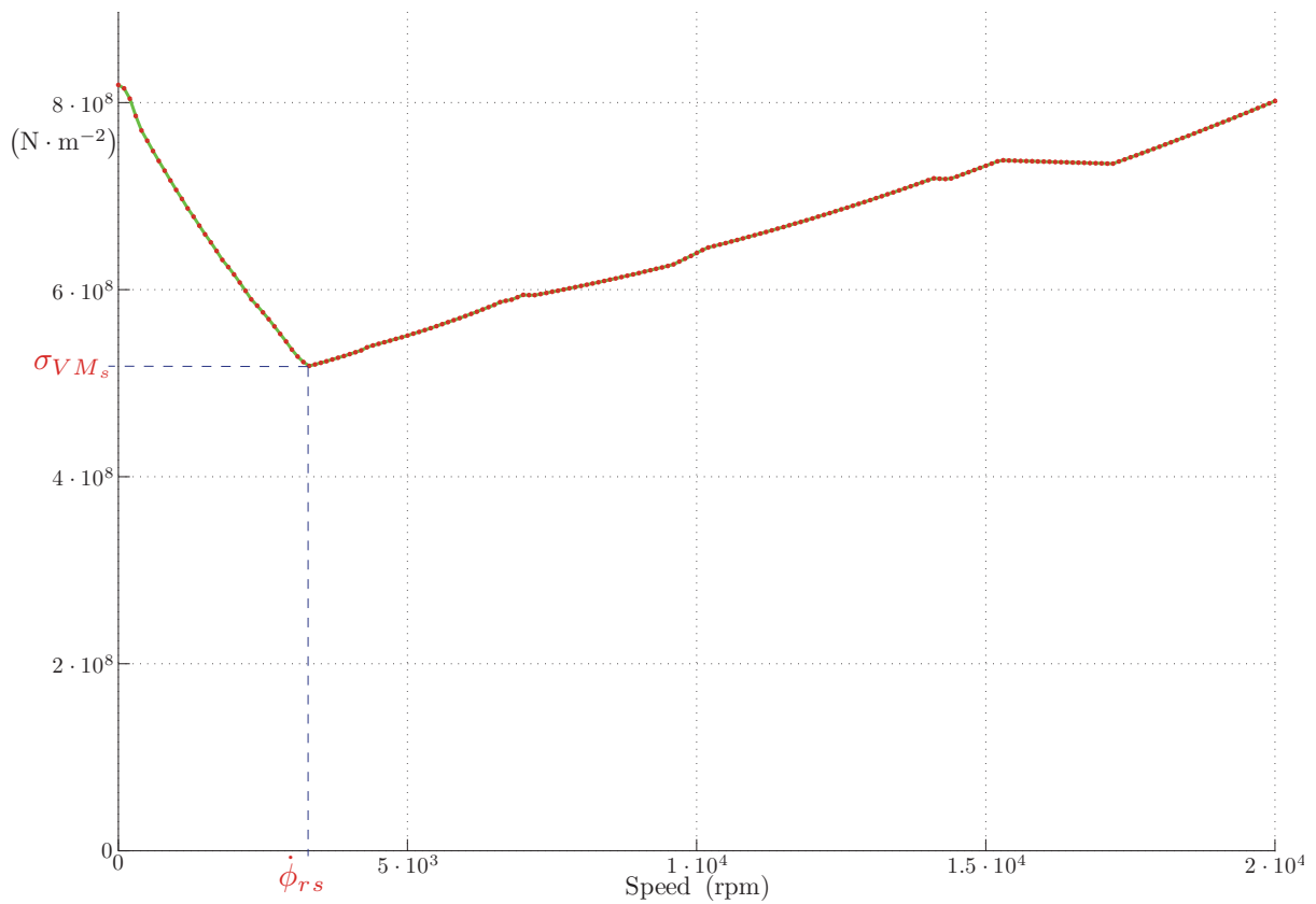
FIGURE 5.23 – Contraintes de \mathcal{V} on \mathcal{M} ises maximales des tirants en fonction de la vitesse de rotation.
