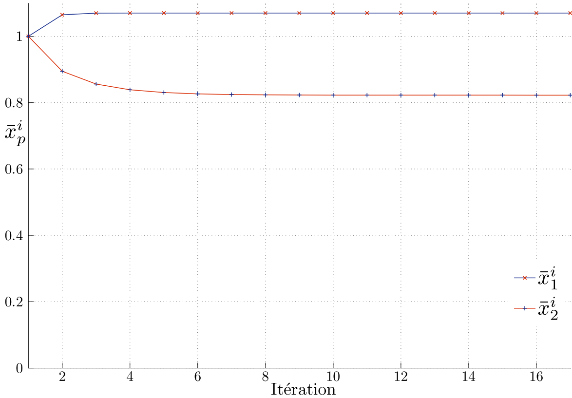
FIGURE E.4 – Évolution des itérés successifs \bar{x}_p , i.e. valeurs relatives des modules d' \mathcal{V} oung (X) et de \mathcal{C} oulomb (+) au cours des itérations.
