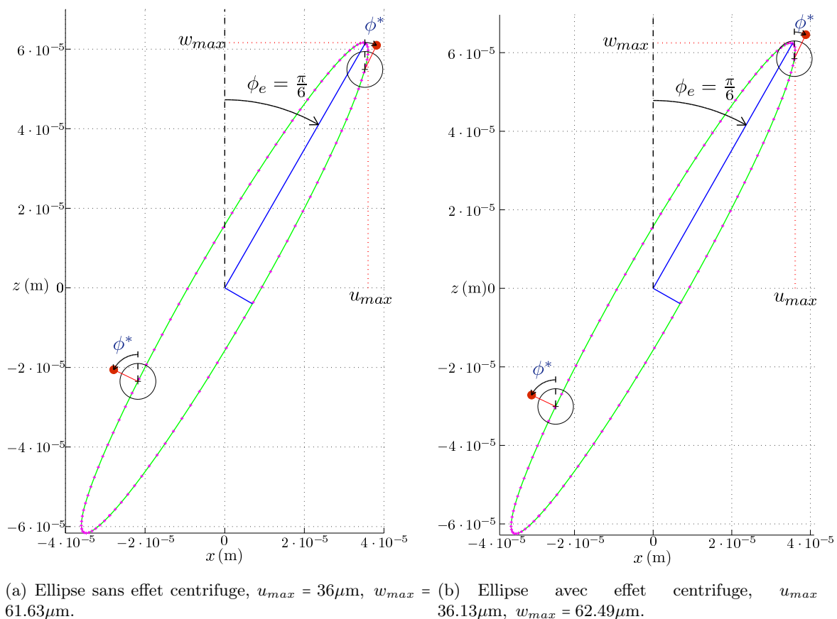
FIGURE 5.26 – Orbites elliptiques au nœud N°90, \dot{\phi}_r = 3\,250 rpm, configuration \mathcal{C}_1 .
