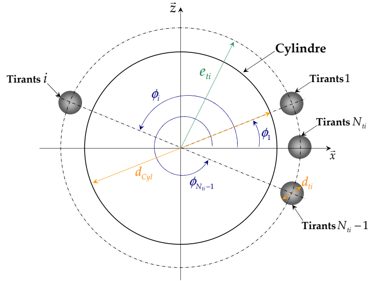
FIGURE B.10 – Paramétrage d'une section droite composée de tirants équirépartis.
