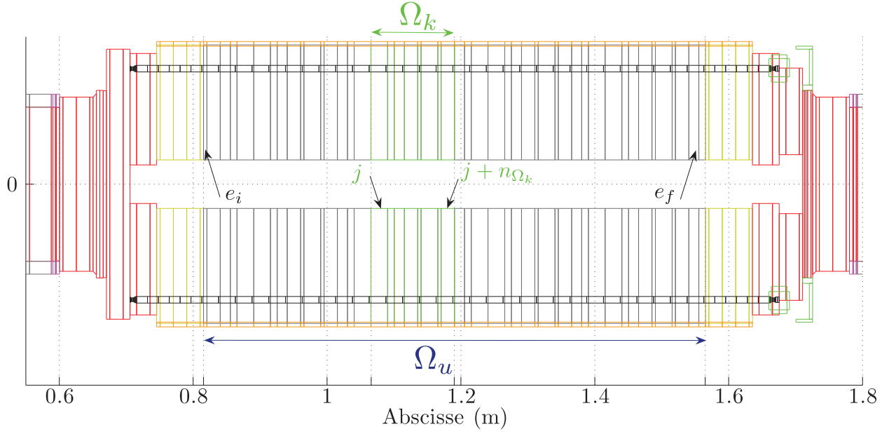
FIGURE 4.1 – Définition d'un sous-domaine sur la masse magnétique discrétisée.
