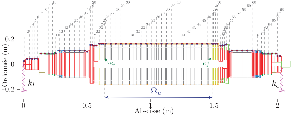
FIGURE 4.13 – Modèle éléments finis contenant n_{\delta_c} = 68 points de mesure (●), n_{\delta} = 352 .
