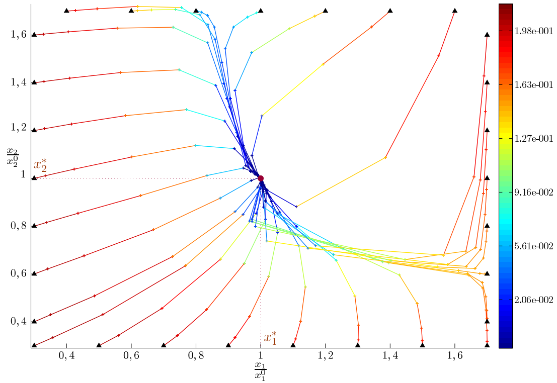
FIGURE 4.19 – Évolution des itérés successifs relatifs (+) au cours du processus de minimisation pour différentes valeurs initiales de paramètres x^0 ( \blacktriangle ). La plage de variation des valeurs initiales x^0 est de \pm 70\% des valeurs optimales de E et G \{x_1^*, x_2^*\} ( \bullet ).
