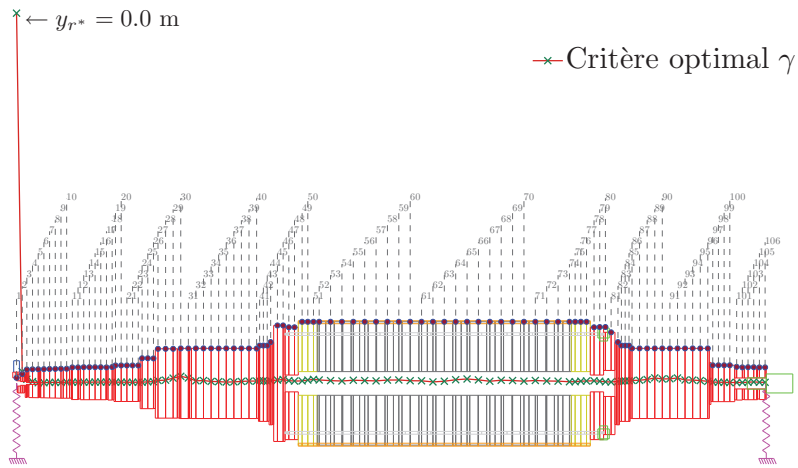
FIGURE 3.12 – Positionnement optimal de l’accéléromètre en x_{r^*} en fonction du critère \gamma (x), 106 points de mesures (•).
