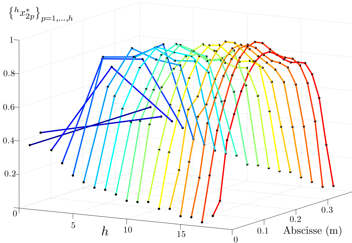
FIGURE 4.11 – Distribution de module de \mathcal{C} oulomb normalisé le long de l’empilement de tôles en fonction du nombre de sous-domaines h = [1, \dots, 18] .
